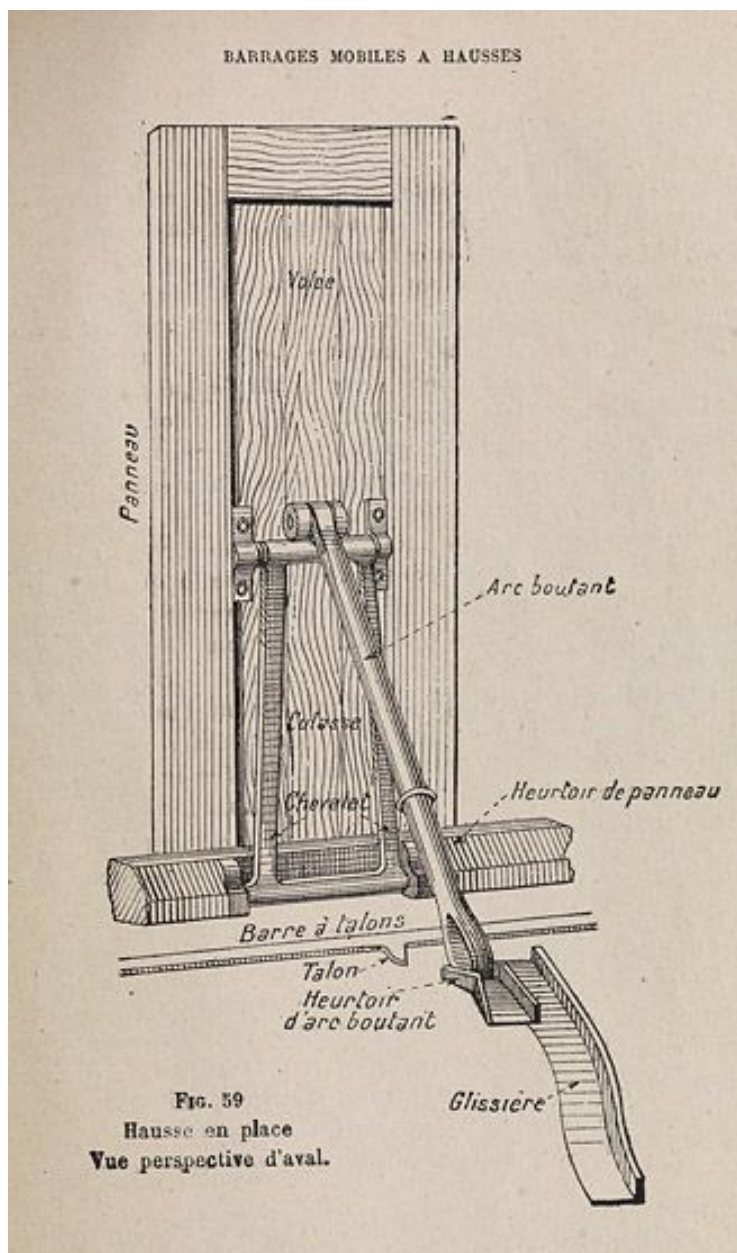
Barrages mobiles à hausses. Hausse en place. Vue perspective d'aval. Tiré de : Notions de navigation intérieure / M. Fourrey. Paris : Ecole spéciale des travaux publics, 1929.
