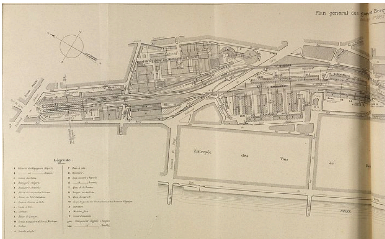
Plan de la tête de ligne du réseau de Paris, Lyon, Méditerranée. Plan général des gares de Bercy (1ère partie). Tiré de : Les gares de Paris et de Villeneuve-Saint-Georges, la tête de ligne du réseau de Paris à Lyon à la Méditerranée, N°1 / Jules Michel. In "Revue Générale des Chemins de Fer", 2e semestre 1887. (Association pour l'histoire des chemins de fer, Paris)
