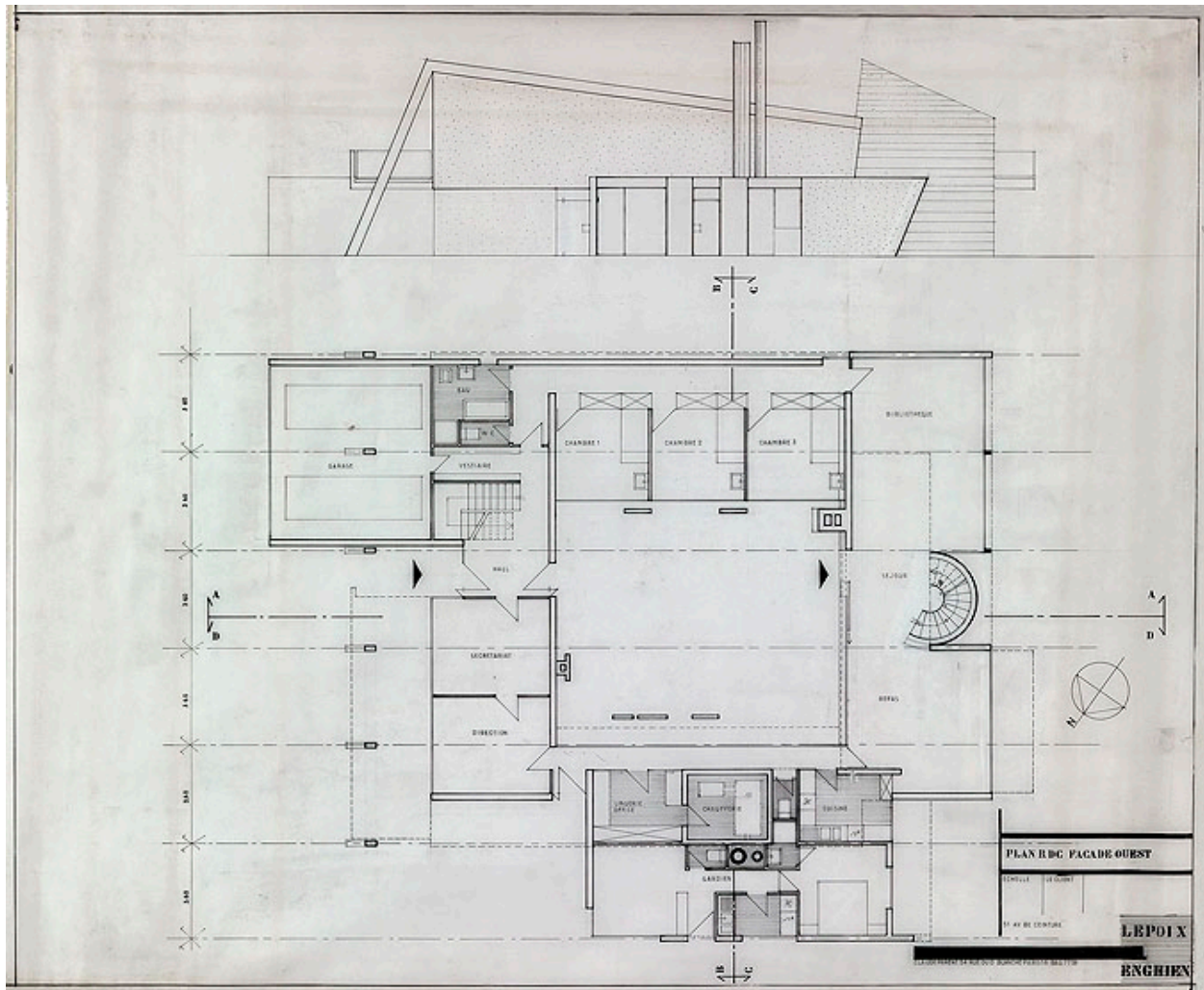
Projet de Claude Parent : plan du rez-de-chaussée et élévation de la façade ouest, 1963. (Institut français d'architecture, Fonds Parent Claude, PARCL-B-63-01)
