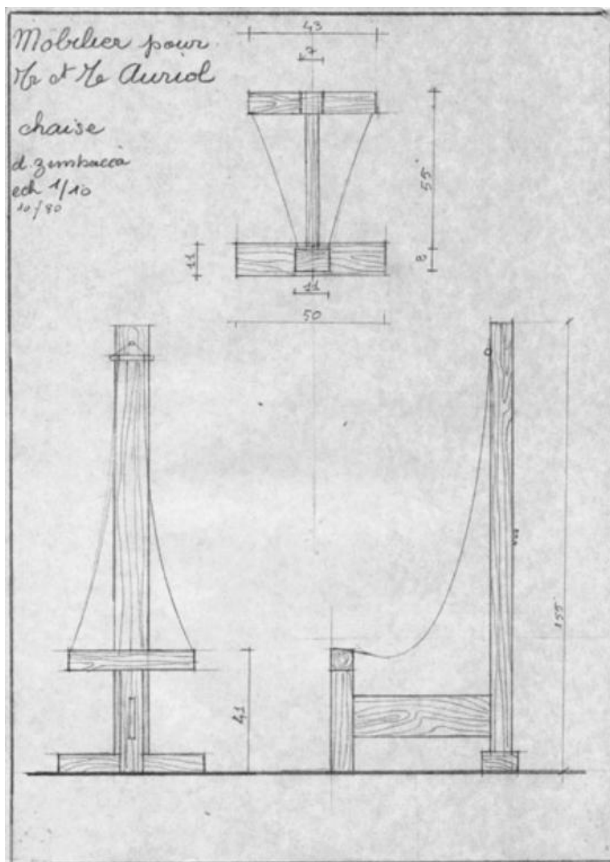
Dessin préparatoire pour la chaise "Elaphe"
