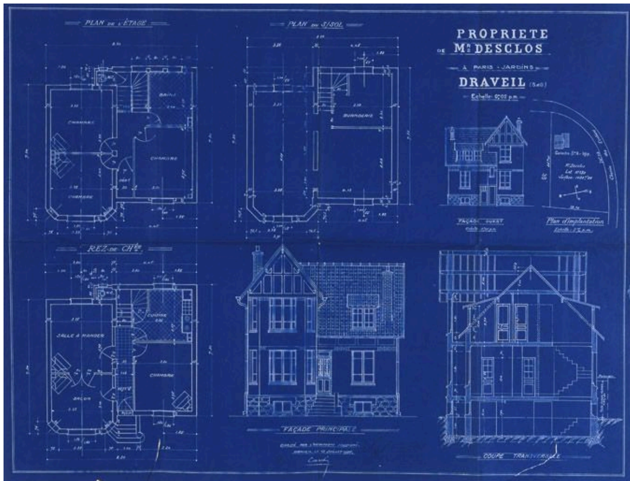
Plans de la maison de M. Desclos : implantation, élévations, coupe et plans par niveaux. (Société coopérative "Paris-Jardins" de Draveil, dossier 130)
