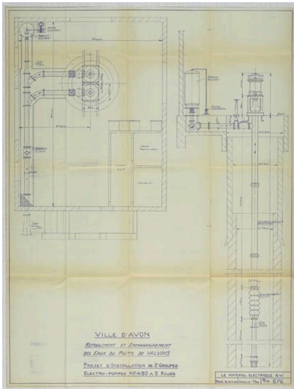
Plan et coupe des groupes électro-pompes installés à la station de pompage de Valvins par Le Matériel électrique S-W en 1954. (AD Seine-et-Marne, 3353W1169 )
