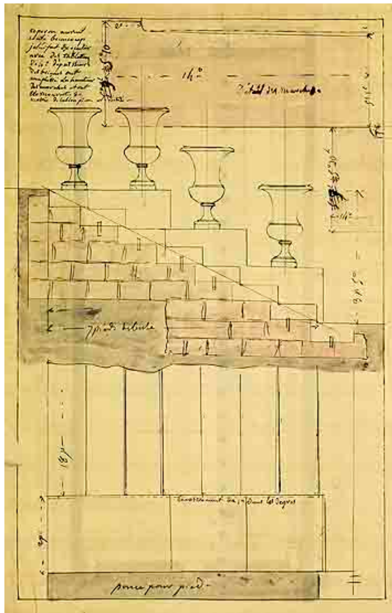
Dessin, aménagement et décors de l'escalier du perron. Projet pour le château? (Ecole nationale des ponts et chaussées, Champs-sur-Marne. Fonds Charles-François Mandar)
