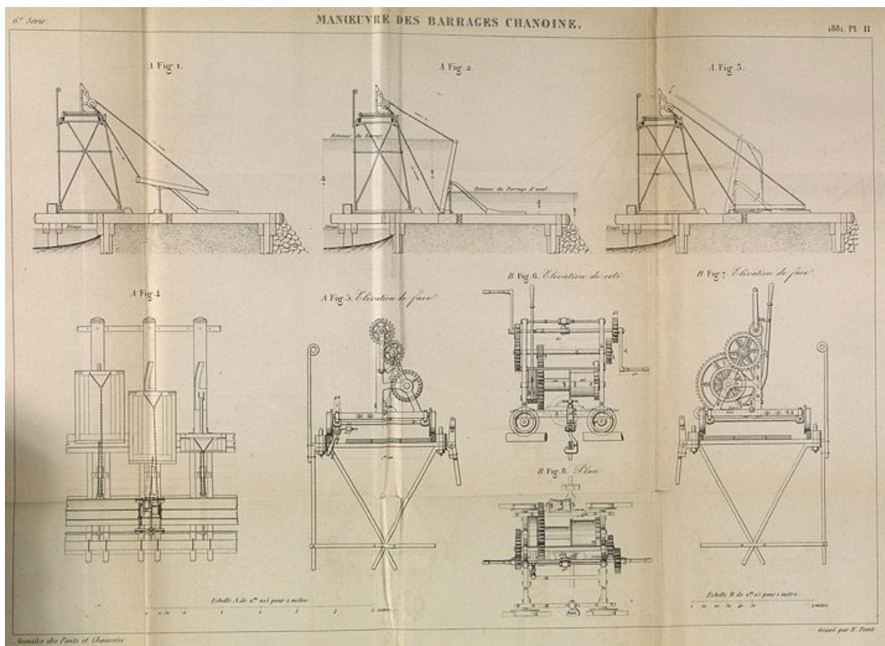
Manoeuvre des barrages Chanoine. Tiré de : Note sur la manoeuvre des barrages Chanoine / Maurice Lévy. In Annales des Ponts et Chaussées, 1er semestre 1881, n° 23, pl. 11.
