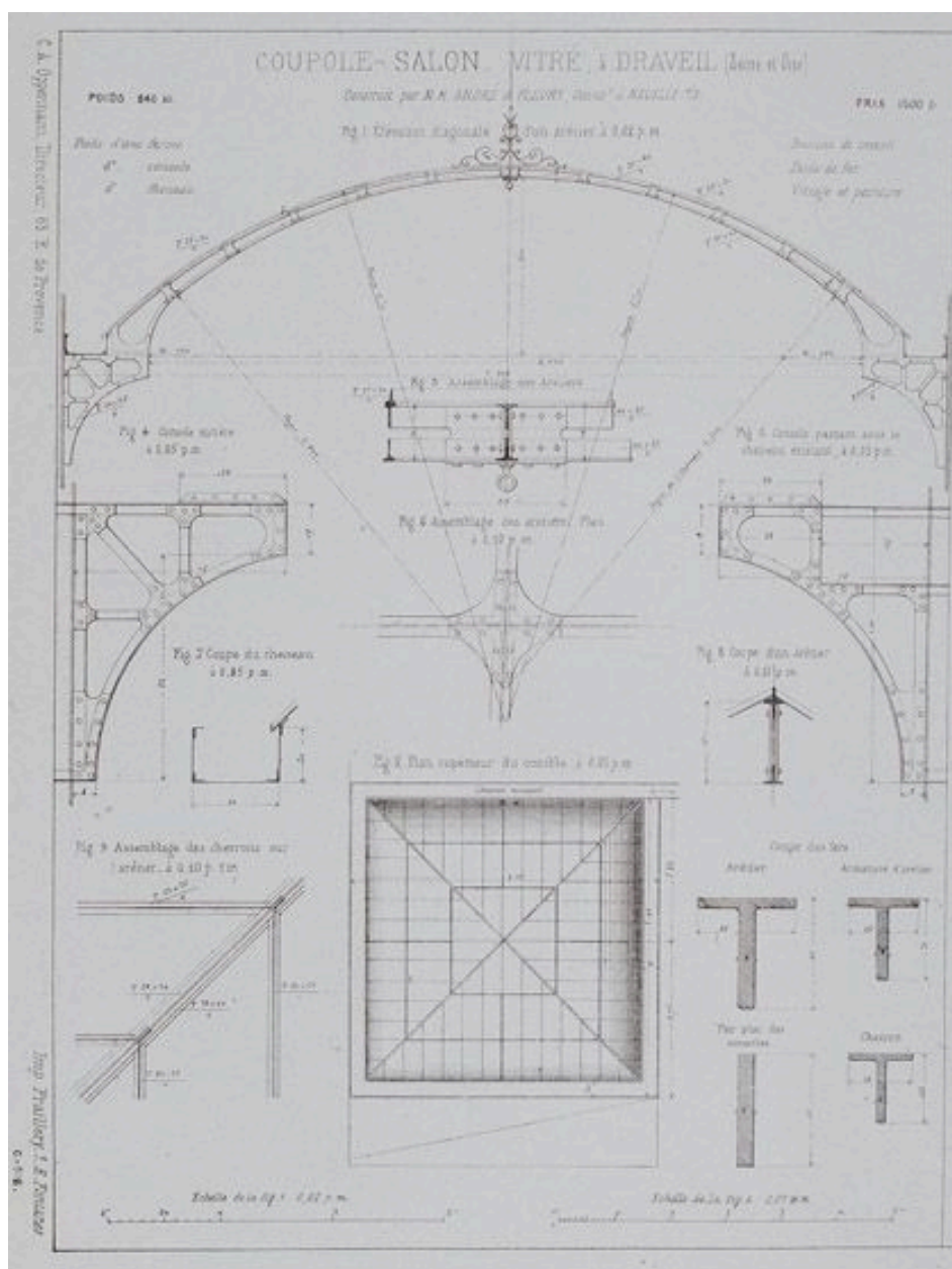
Plan, coupe, élévation, détail de la coupole du salon vitré de jardin (accolé à la façade ouest des dépendances), édifié par André et Fleury, constructeurs à Neuilly-sur-Seine. Tiré de : Nouvelles annales de la construction, 1873, col. 77-78. (BHVP, Per F° 121)
