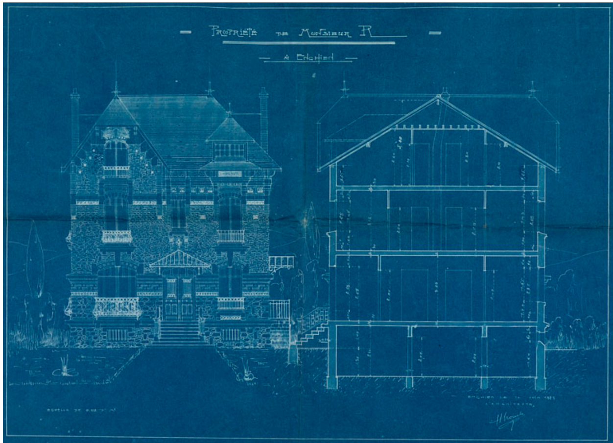
Élévation et coupe d'une maison construite pour monsieur "R", en 1923 (non localisée). (AM Enghien-les-Bains, Fonds des autorisations de permis de construire)
