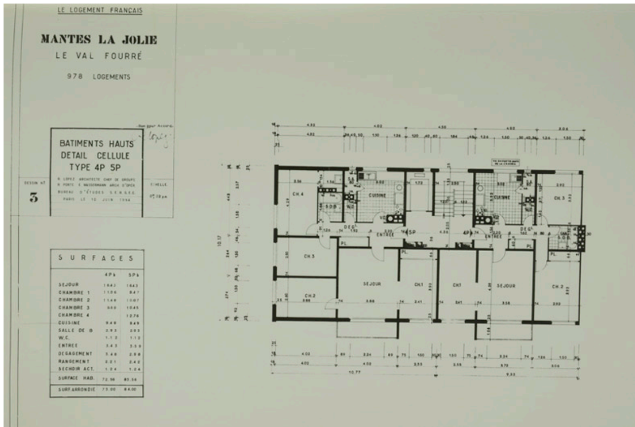
Quartier 1, des Ecrivains. Plan des bâtiments de huit étages, cellules 4 pièces et 5 pièces. (Archives Nationales, Direction de l'Habitat et de la Construction, 19840091/58-59)
