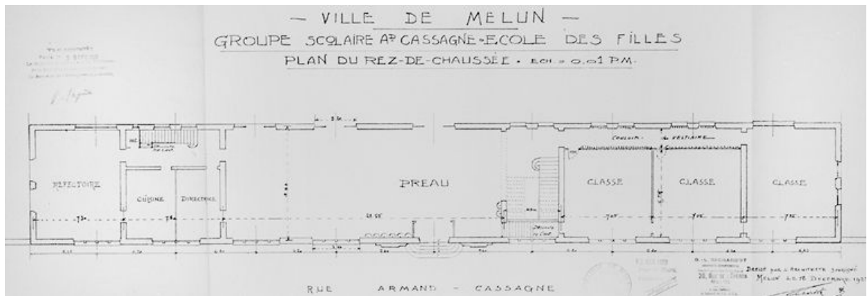
Ecole des filles : plan du rez-de-chaussée. Ech 1 : 100. Papier (tirage d'architecte), 12 décembre 1922. (AM Melun. 1 Fi 724)
