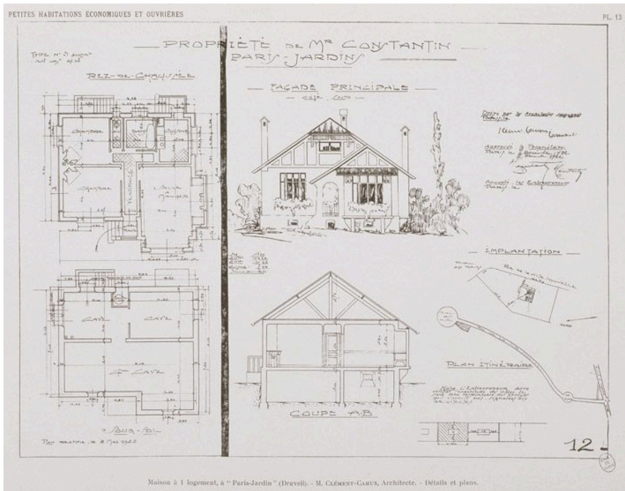
Élévation, coupe et plans du pavillon construit, pour M. Constantin. Plans, 7 décembre 1922. Tiré de : Petites habitations économiques et ouvrières./ Hector Saint-Sauveur. Paris : Ch. Massin et Cie, [192?]. (BHVP, 94066)
