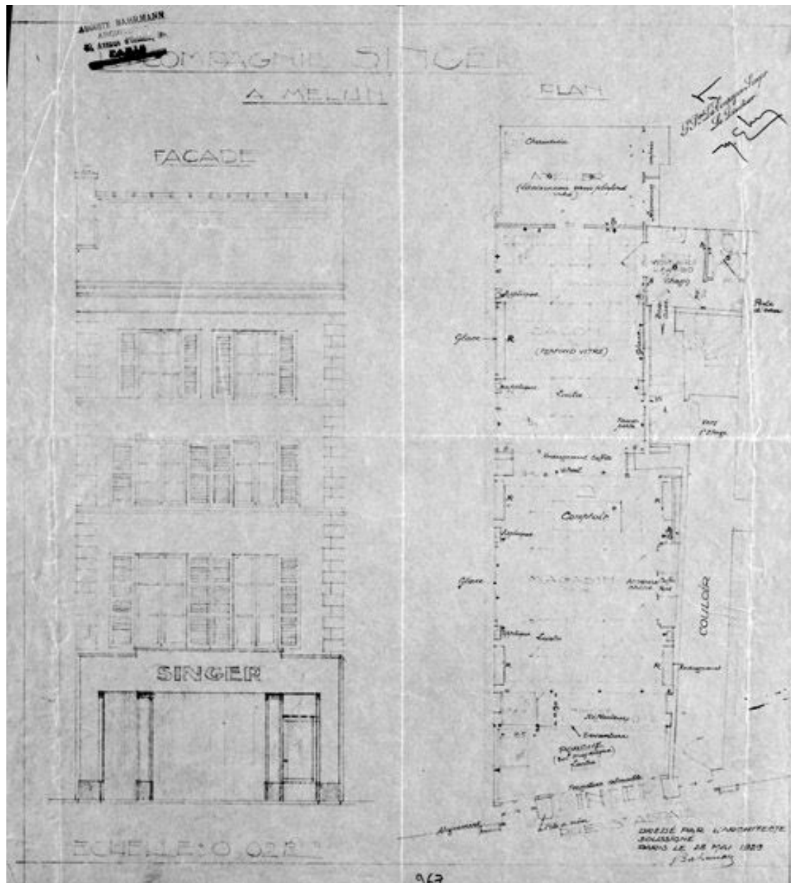
Plan et façade de l'immeuble, 8 rue Saint-Aspais, abritant au rez-de-chaussée le magasin Singer. Tirage d'architecte, 1929 (8 mai). (AM Melun. 1 Fi 967)
