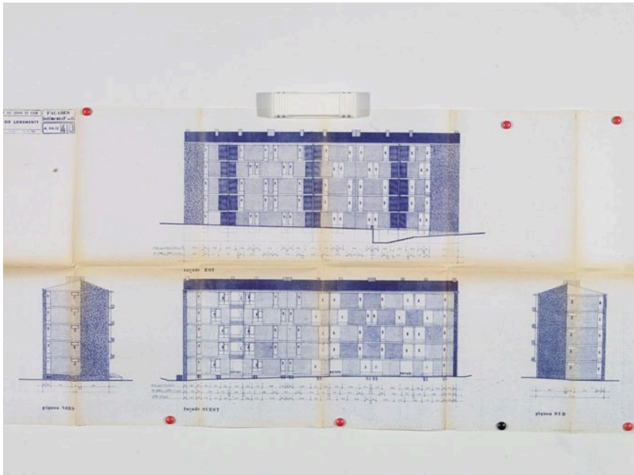
Deuxième tranche de 60 logements : plan des façades et pignons des bâtiments F et G (4 étages carrés), 24 juillet 1964. (AD Essonne, 1502 W 1254)
