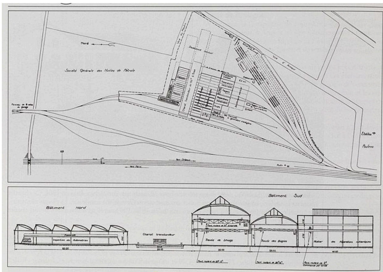
Vitry-sur-Seine. Plan et coupe des ateliers de réparation ferroviaires de la gare des Ardoines. Tiré de : Le chemin de fer Paris Orléans/J.-P. Vergez-Larrouy. Paris : la Vie du Rail, la Régordane, 1997.
