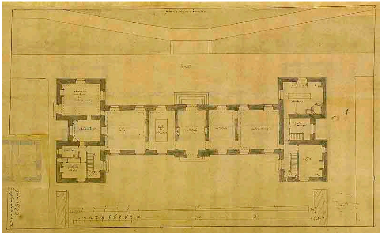
Plan du rez-de-chaussée du château. Attribution des pièces. (Ecole nationale des ponts et chaussées, Champs-sur-Marne. Fonds Charles-François Mandar)
