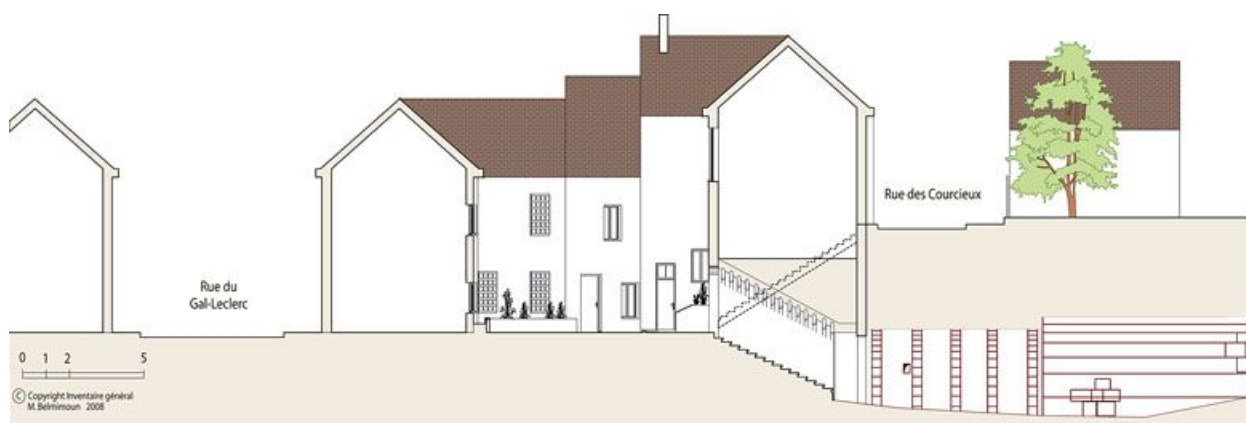
Coupe transversale de la rue du Général-Leclerc à la rue des Courcieux.
