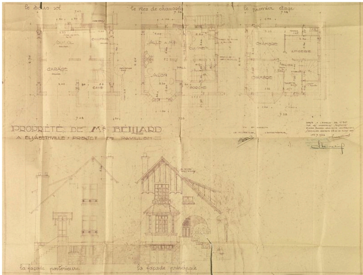
Plans de la maison de M. Beillard, architectes Eugène Boucher et S. Chevalier, 1936. (AM Aubergenville).
