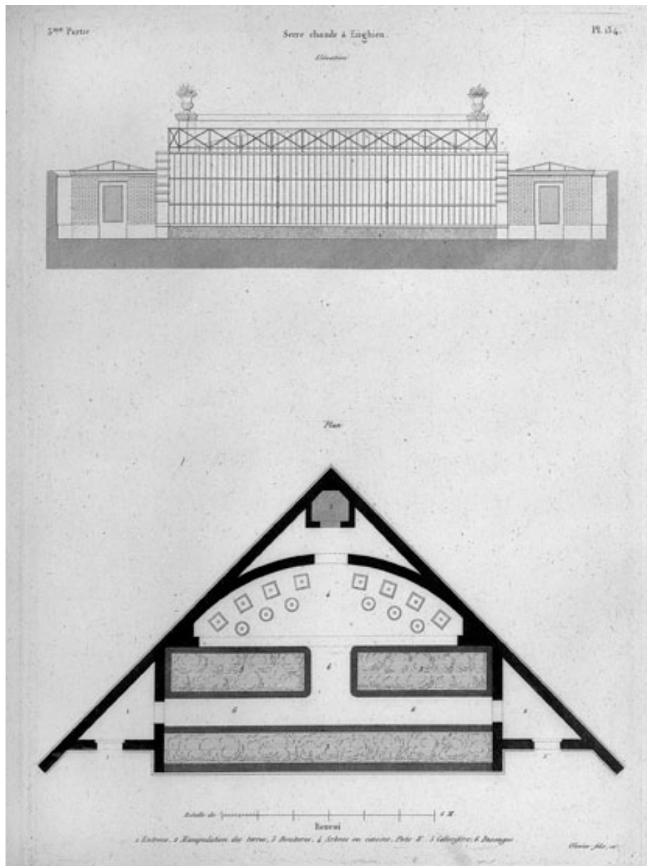
Plan et élévation d'une serre chaude. Gravure. (BHVP, in fol. 10 84)
