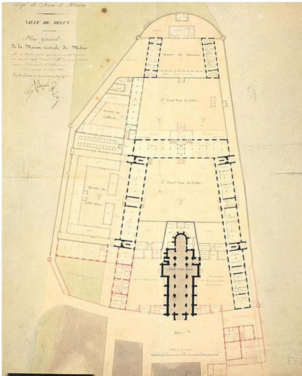
Département de Seine-et-Marne. Ville de Melun. Plan général de la maison centrale de Melun, refait sur les plans partiels approuvés et complétés de concert avec Monsieur Vallet directeur à l'effet de proposer à l'autorité supérieure l'achèvement de l'établissement.. Papier aquarellé, 1828, éch. 1/400e. (BM Melun. FF 4)
