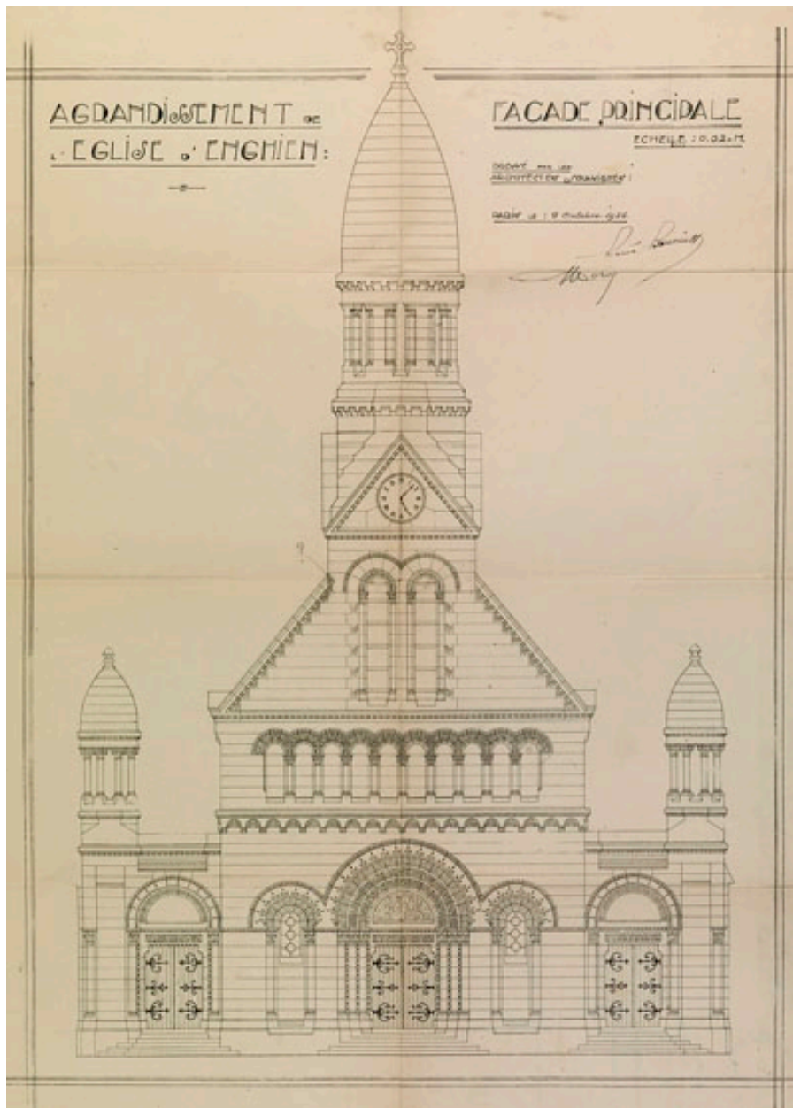
Elévation de la nouvelle façade conçue en 1926. (AM Enghien-les-Bains, M48)
