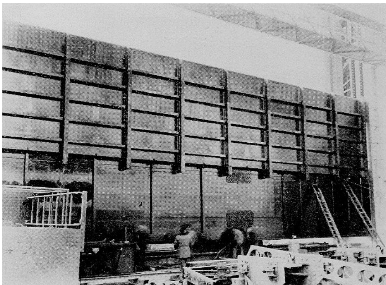
fig. 6. — Montage sur place des vannes inférieure et supérieure. Vu
