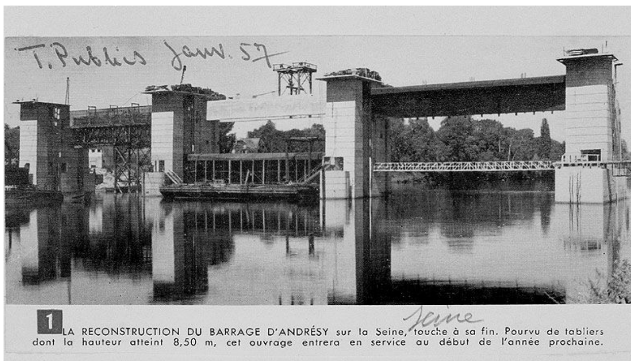
Vue du barrage en cours de construction. Photographie imprimée. Travaux publics, janvier 1957. (Musée de l'Ile-de-France).
