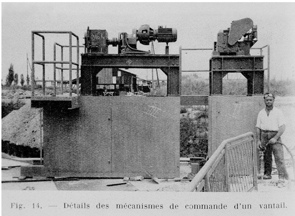
Construction du barrage : détail des mécanismes de commande d'un vantail. Photographie imprimée. Tiré de : Construction, t. XV, n° 5, mai 1960. (Musée de l'Île-de-France).
