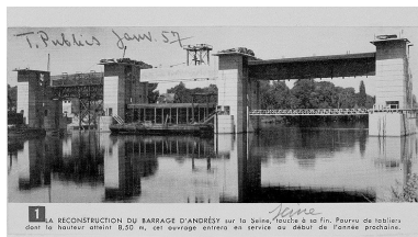
Vue du barrage en cours de construction. Photographie imprimée. Travaux publics, janvier 1957. (Musée de l'Ile-de-France). Autr. Louis Rémy Sabattier IVR11_20027800579XB
