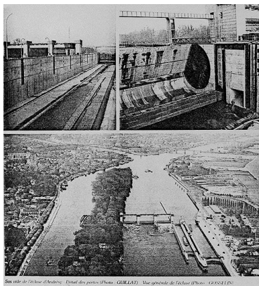
Vue générale de l' écluse et détails du sas vide et des portes. Photographie imprimée. Tiré de : L'Eclusier, novembre 1986. (Musée de l'Ile-de-France). Autr. Louis Rémy Sabattier IVR11_20027800578XB
