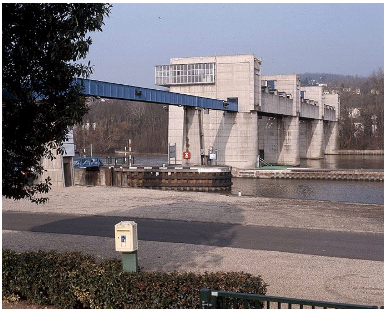
Vue arrière des cabines de manoeuvre des vannes.
