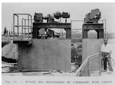
Construction du barrage : détail des mécanismes de commande d'un vantail. Photographie imprimée. Tiré de : Construction, t. XV, n° 5, mai 1960. (Musée de l'Ile-de-France). Autr. Louis Rémy Sabattier IVR11_20027800580XB
