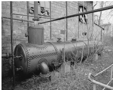
Chaudière. Photographie. (AD Seine-Saint-Denis. A NB 92) IVR11_20029300104NUC
