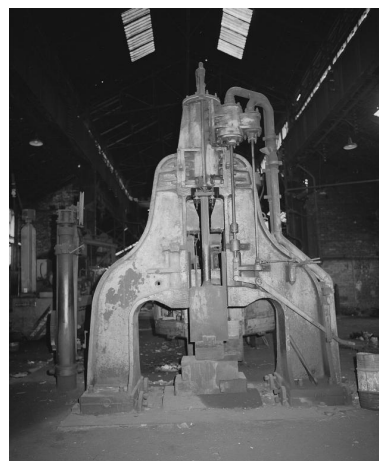
Forge presse. Photographie. (AD Seine-Saint-Denis. A NB 92) IVR11_20029300108NUC
