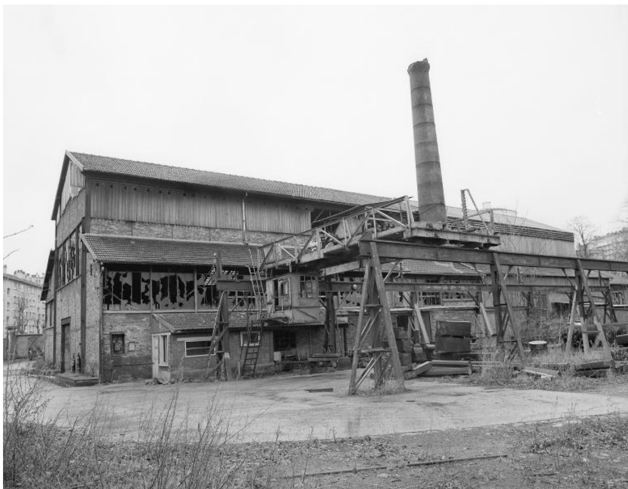
Le bâtiment de forgeage et le pont roulant. Photographie. (AD Seine-Saint-Denis. A NB 92)
