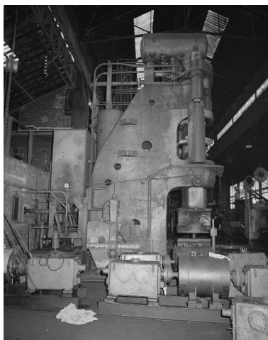
Presse. Photographie. (AD Seine-Saint-Denis. A NB 92) IVR11_20029300113NUC
