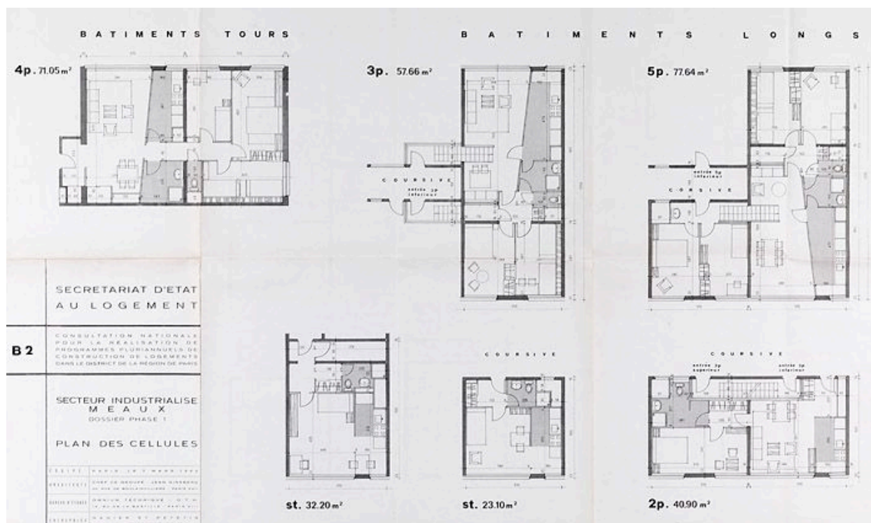
La Pierre-Collinet. Plan des logements des barres et des tours. (Cité de l'architecture et du patrimoine. fonds Ginsberg 100 boîte 408)
