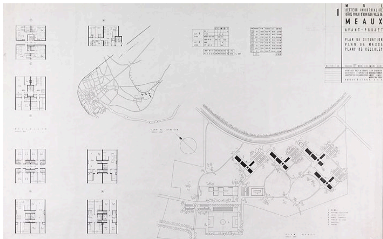
La Pierre-Collinet. Plan de situation, plan masse, plan des cellules. (Cité de l'architecture et du patrimoine, fonds Ginsberg 100 rouleau RB 1070)
