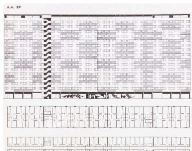
La Pierre-Collinet. Projet de façade des barres. Tiré de : "Architecture Aujourd'hui", n° 89 (Cité de l'architecture et du patrimoine) IVR11_20097701043NUC4A
