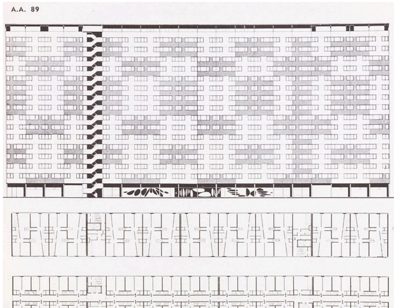
La Pierre-Collinet. Projet de façade des barres. Tiré de : "Architecture Aujourd'hui", n° 89 (Cité de l'architecture et du patrimoine)
