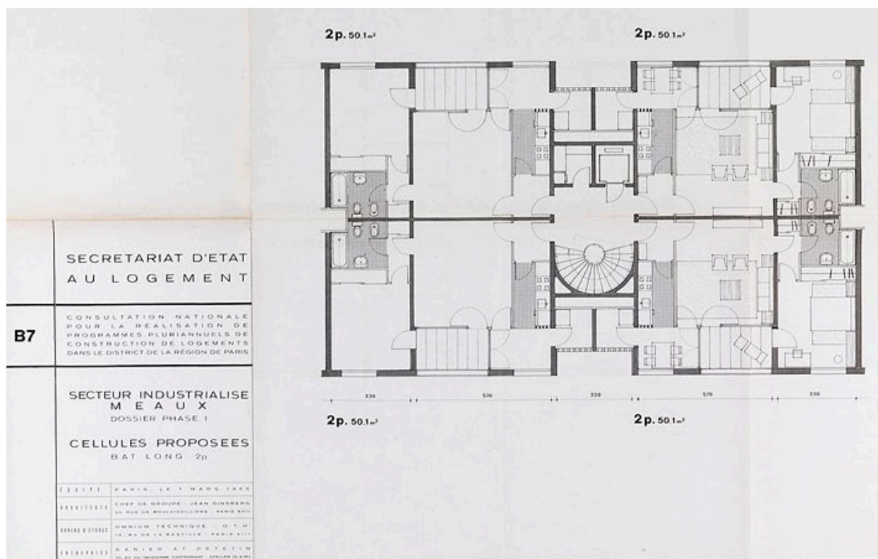
La Pierre-Collinet. Plan des logements des barres et des tours des 2 pièces. (Cité de l'architecture et du patrimoine. fonds Ginsberg 100 boîte 408)
