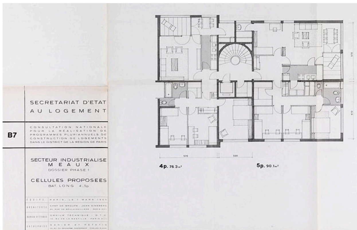
La Pierre-Collinet. Plan des logements des barres et des tours des 4 pièces et 5 pièces. (Cité de l'architecture et du patrimoine. fonds Ginsberg 100 boîte 408)
