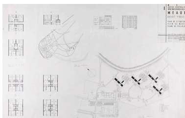
La Pierre-Collinet. Plan de situation, plan masse, plan des cellules. (Cité de l'architecture et du patrimoine. fonds Ginsberg 100 rouleau RB 1070) IVR11_20097701041NUC4A
