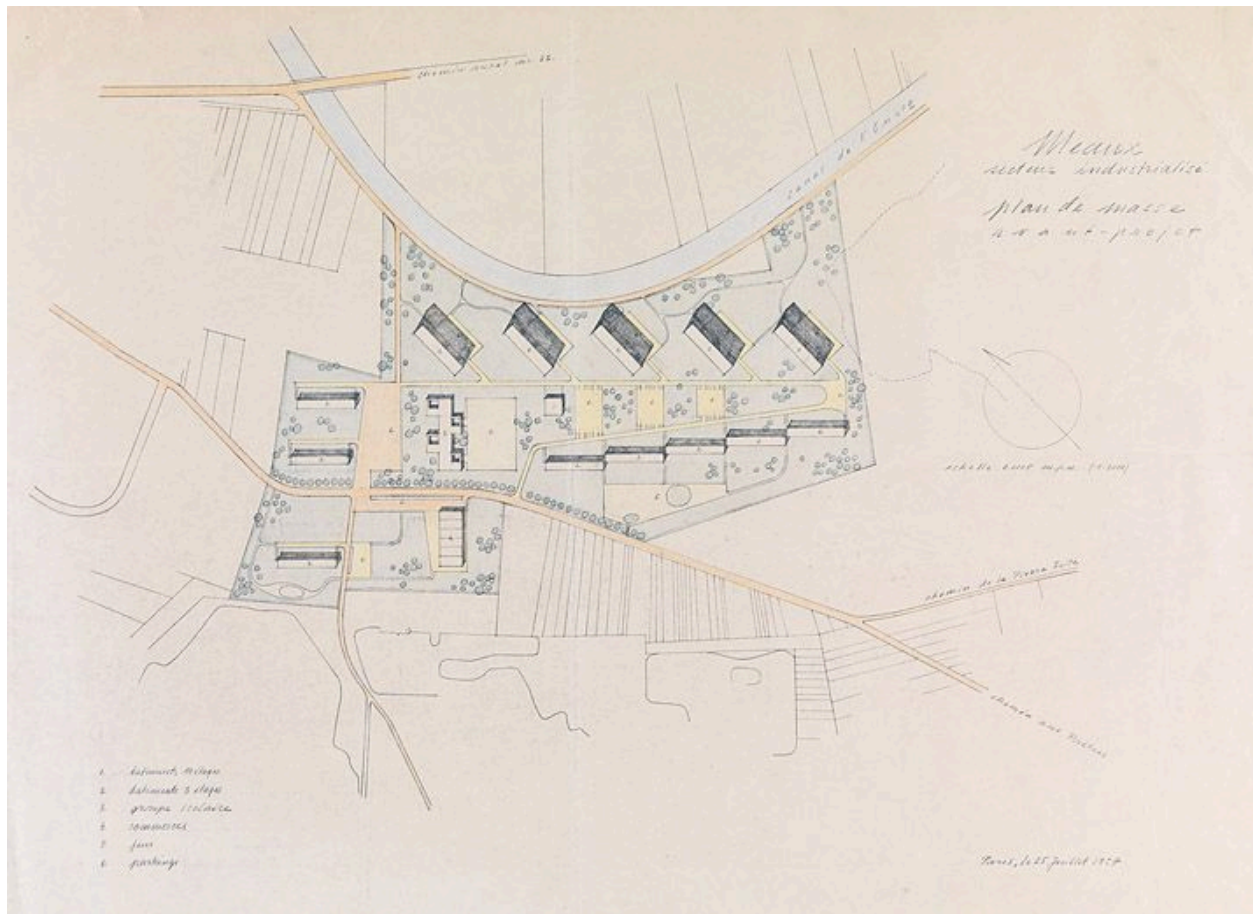
La Pierre-Collinet. Plan masse d'un premier projet. (Cité de l'architecture et du patrimoine. fonds Ginsberg 100 rouleau RB 1070)
