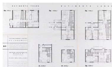
La Pierre-Collinet. Plan des logements des barres et des tours. (Cité de l'architecture et du patrimoine. fonds Ginsberg 100 boîte 408) IVR11_20097701045NUC4A
