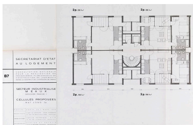
La Pierre-Collinet. Plan des logements des barres et des tours des 2 pièces. (Cité de
