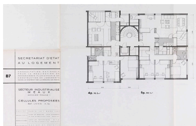
La Pierre-Collinet. Plan des logements des barres et des tours des 4 pièces et 5 pièces. (Cité de
