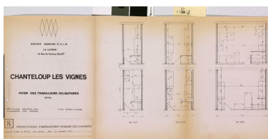
La Noé. Société anonyme d'HLM La Lutèce. Chanteloup les Vignes, foyer des travailleurs célibataires, 600 lits. Proposition d'aménagement mobilier des chambres. Emile Aillaud architecte. Janvier 1972. Les travailleurs sont répartis dans des chambres individuelles (9,45 m²), chambres doubles (15,20 m²) ou chambres à trois lits (29 m²). (Cité de l'architecture et du patrimoine, Archives d'architecture du XXe siècle). Phot. Laurent Kruszyk IVR11_20087800388NUC4A
