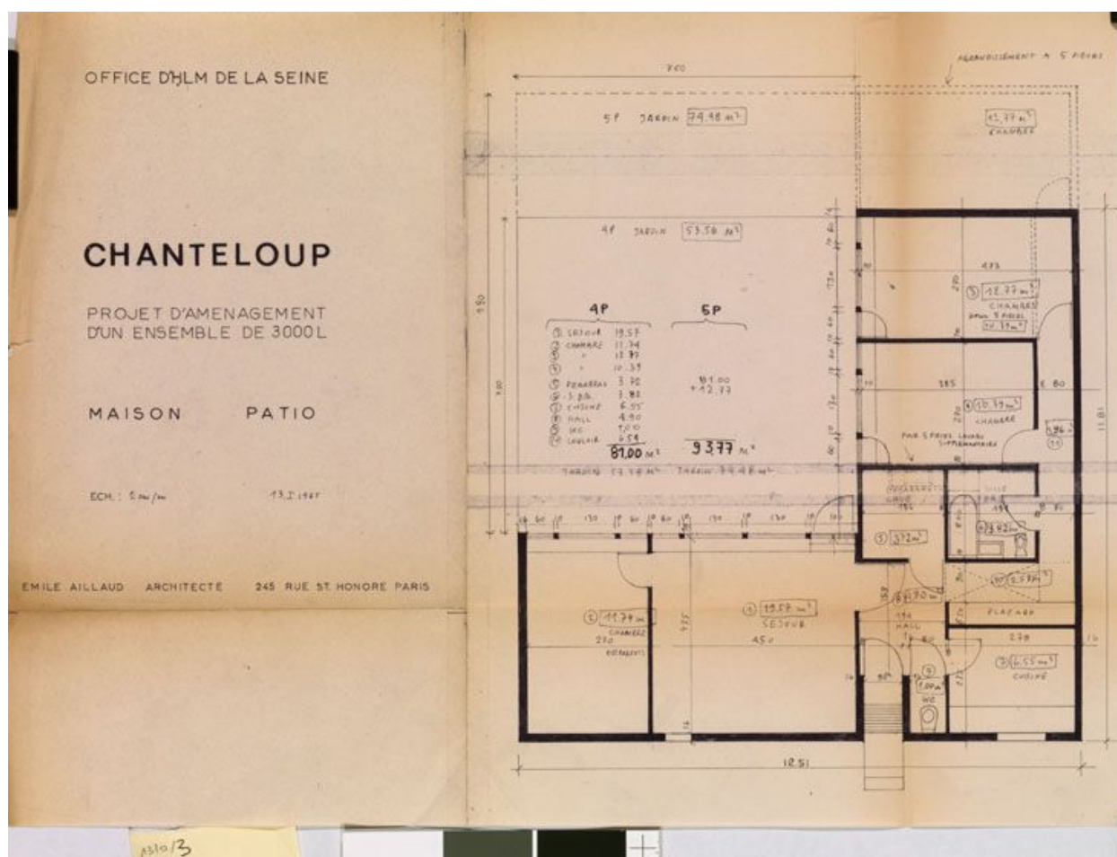
La Noé. Office d'HLM de la Seine. Chanteloup, projet d'aménagement d'un ensemble de 3000 logements. Maison patio, plan, janvier 1965, signé Emile Aillaud. (Cité de l'architecture et du patrimoine, Archives d'architecture du XXe siècle).
