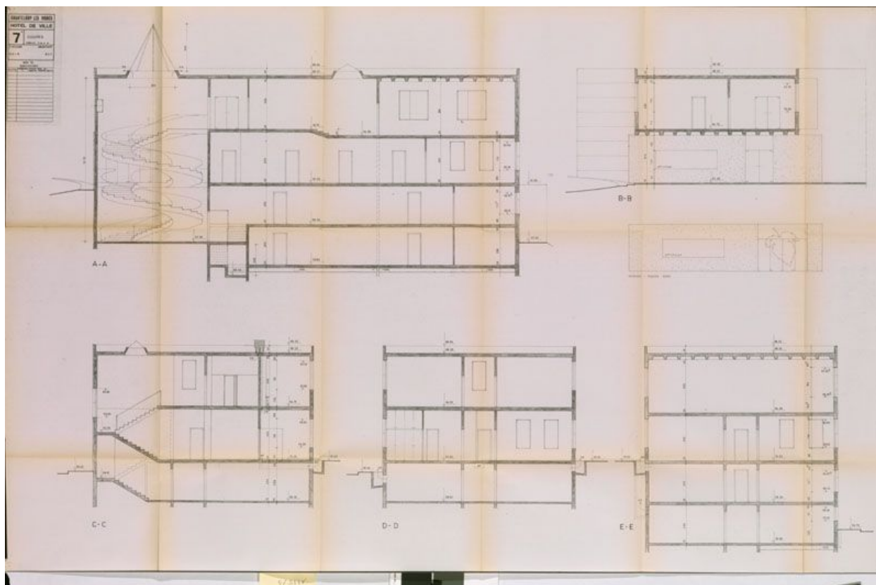
La Noé. Chanteloup les Vignes, hôtel de ville. Coupes, 1974. Emile Aillaud architecte. Le bâtiment n'a pas été construit. (Cité de l'architecture et du patrimoine, Archives d'architecture du XXe siècle).
