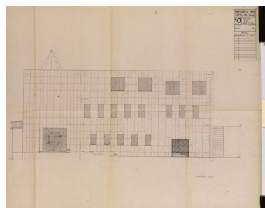
La Noé. Chanteloup les Vignes, hôtel de ville. Façade sud, 1974. Emile Aillaud architecte. Le bâtiment n'a pas été construit. Les façades étaient prévues recouvertes de marbre blanc. (Cité de l'architecture
