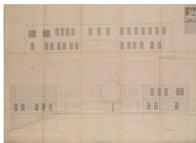
La Noé. Chanteloup les Vignes, hôtel de ville. Façade est, 1974. Emile Aillaud architecte. Le bâtiment n'a pas été construit. Les façades étaient prévues recouvertes de marbre blanc. (Cité de l'architecture
