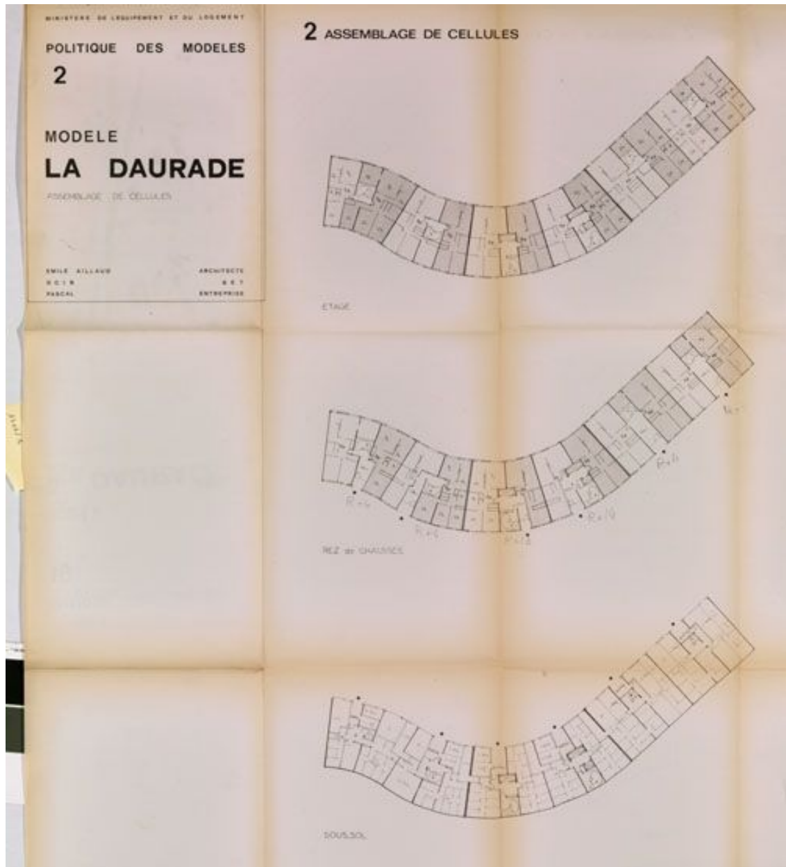
La Noé. Ministère de l'équipement et du logement, Politique des modèles. Modèle La Daurade, assemblage des cellules. Emile Aillaud, architecte. OCIB, BET. Pascal, entreprise. S. d. (les pièces écrites du dossier sont datées d'octobre 1972). (Cité de l'architecture et du patrimoine, Archives d'architecture du XXe siècle).
