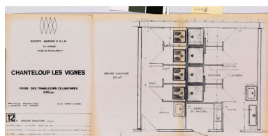
La Noé. Société anonyme d'HLM La Lutèce. Chanteloup les Vignes, foyer des travailleurs célibataires, 249 chambres. Plan d'un groupe sanitaire en étage. Emile Aillaud architecte. Janvier/octobre 1972. Le cartouche indique les modificatifs successifs, dont la dernière : suppression des lavabos, pour ne conserver qu'un bac à laver et un lavabo pour quatre douches. (Cité de l'architecture et du patrimoine, Archives d'architecture du XXe siècle). Phot. Laurent Kruszyk IVR11_20087800387NUC4A
