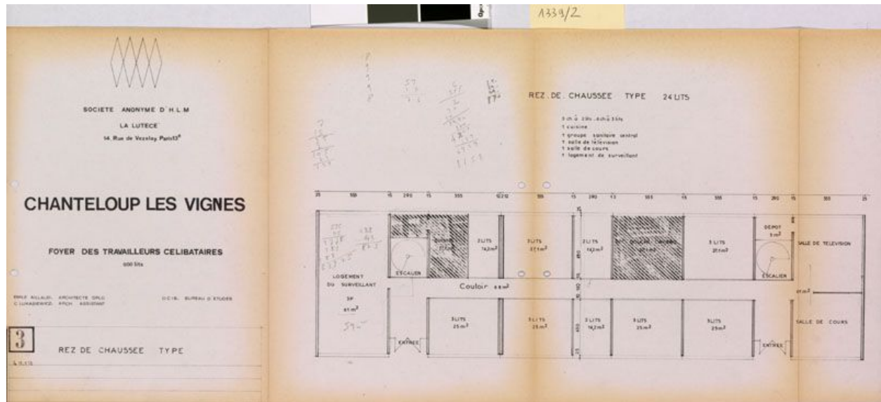
La Noé. Société anonyme d'HLM La Lutèce. Chanteloup les Vignes, foyer des travailleurs célibataires, 600 lits. Plan d'un rez-de-chaussée type. Emile Aillaud architecte. janvier 1972. (Cité de l'architecture et du patrimoine, Archives d'architecture du XXe siècle).
