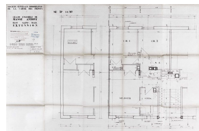
Plan d'un logement de 3 pièces réalisé le 30 avril 1959 par les architectes Sonrel, Duthilleul et Mikaelian. Plan, échelle 1/20, 1959. (AD Essonne, 1153W 331) Autr. Pierre (architecte) Sonrel, Autr. Jean (architecte) Duthilleul, Autr. B. (architecte). Mikaelian IVR11_20109100126NUC4A
