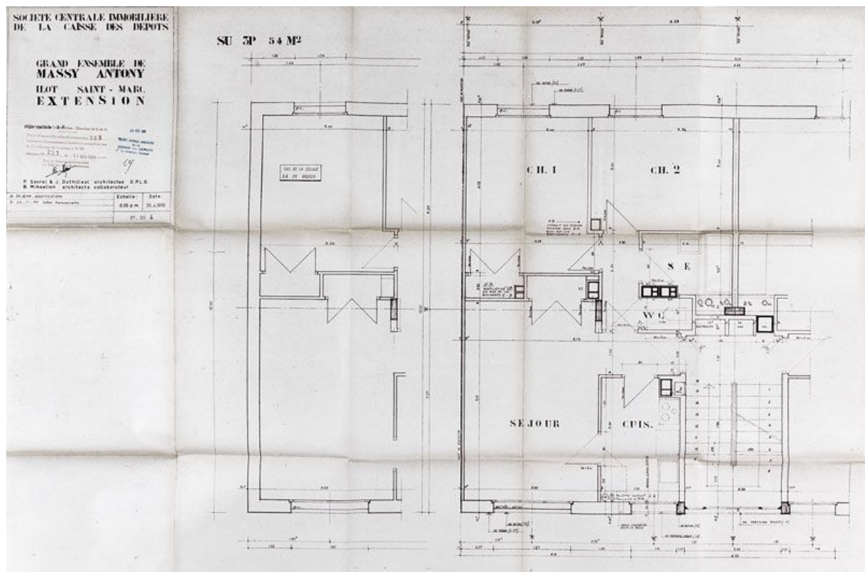
Plan d'un logement de 3 pièces réalisé le 30 avril 1959 par les architectes Sonrel, Duthilleul et Mikaelian. Plan, échelle 1/20, 1959. (AD Essonne, 1153W 331)
