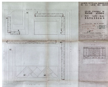
Plan de répartition des rez-de-chaussée réalisé le 17 août 1959 par les architectes Sonrel, Duthilleul et Mikaelian. Plan, échelle 1/500, 1959. (AD Essonne, 1153W 331) Autr. Pierre (architecte) Sonrel, Autr. Jean (architecte) Duthilleul, Autr. B. (architecte). Mikaelian IVR11_20109100125NUC4A
