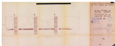
Plan masse des trois barres R+16 situées rue des Canadiens. (AM Massy, 7 T 199) IVR11_20119100153NUC4A
