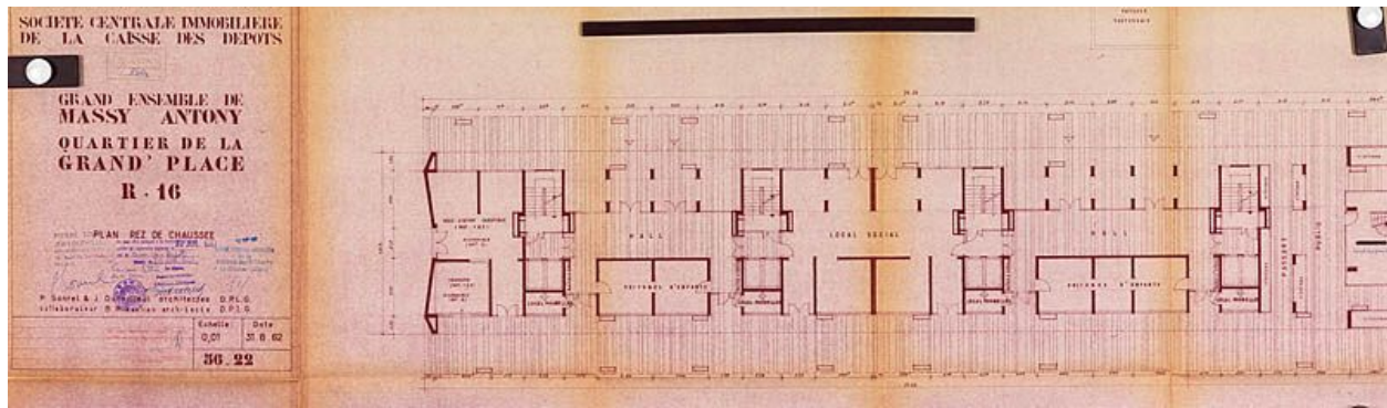
Plan de rez-de-chaussée d'une barre R+16, 31 août 1962. (AM Massy, 7 T 199)
