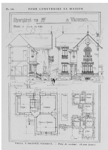
Élévation, coupe et plans des niveaux d'un pavillon. Tiré de : Pour construire sa maison. Recueil de constructions édifiées d'après les plans et devis de M. Bourniquel, architecte-expert / Bourniquel. Paris : Garnier Fr, [1918]. (BHVP, 116028) Autr. Bourniquel (architecte) IVR11_20069100182X
