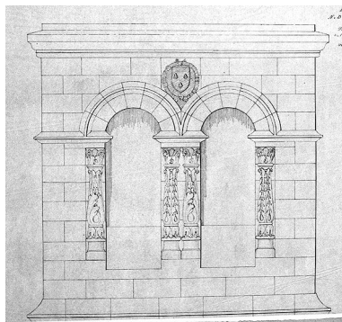
La tour sud : élévation ouest, partie supérieure. Encre sur calque, 19e siècle. (BM Melun. HH 7) Phot. Philippe Ayrault, Autr. C. Guillaume IVR11_20027701108X
