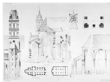
Plans, coupes, élévations. Tiré de : L'Encyclopédie d'architecture, 1890-191. (BNF, Département des estampes. Topo Va Seine-et-Marne) Phot. Département des Estampes (reproduction) Bibliothèque nationale de France, Autr. E Bérard IVR11_20057700361Z
