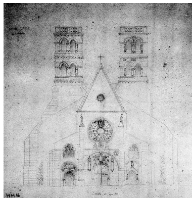
Plan et élévation de la collégiale avant la restauration de Millet. Papier aquarellé. (Musée municipal de Melun. inv. 970.17.2)
