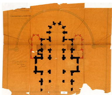
Eglise Notre-Dame : projet de construction des sacristies. Plan. Calque, encre noire et rouge, 1868. (AM Melun. 1 Fi 2099) Phot. Archives municipales de Melun (reproduction), Autr. Buval (architecte de la ville) IVR11_20047700523NUCA
