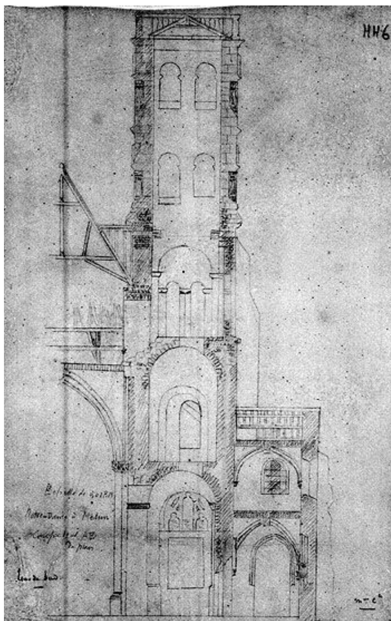
Coupe transversale sur la tour sud. éch. 0.01 p.m. Crayon sur calque, 19e siècle. (BM Melun. HH 6)
