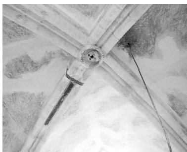
Voûte de la nef, vue depuis un échaffaudage en 2005. L'ogive a été confortée par un élément métallique. Phot. Stéphane Asseline IVR11_20057700277X
