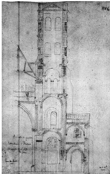
Coupe transversale sur la tour sud. éch. 0.01 p.m. Crayon sur calque, 19e siècle. (BM Melun. HH 6) Phot. Philippe Ayrault, Autr. C. Guillaume IVR11_20027701107X
