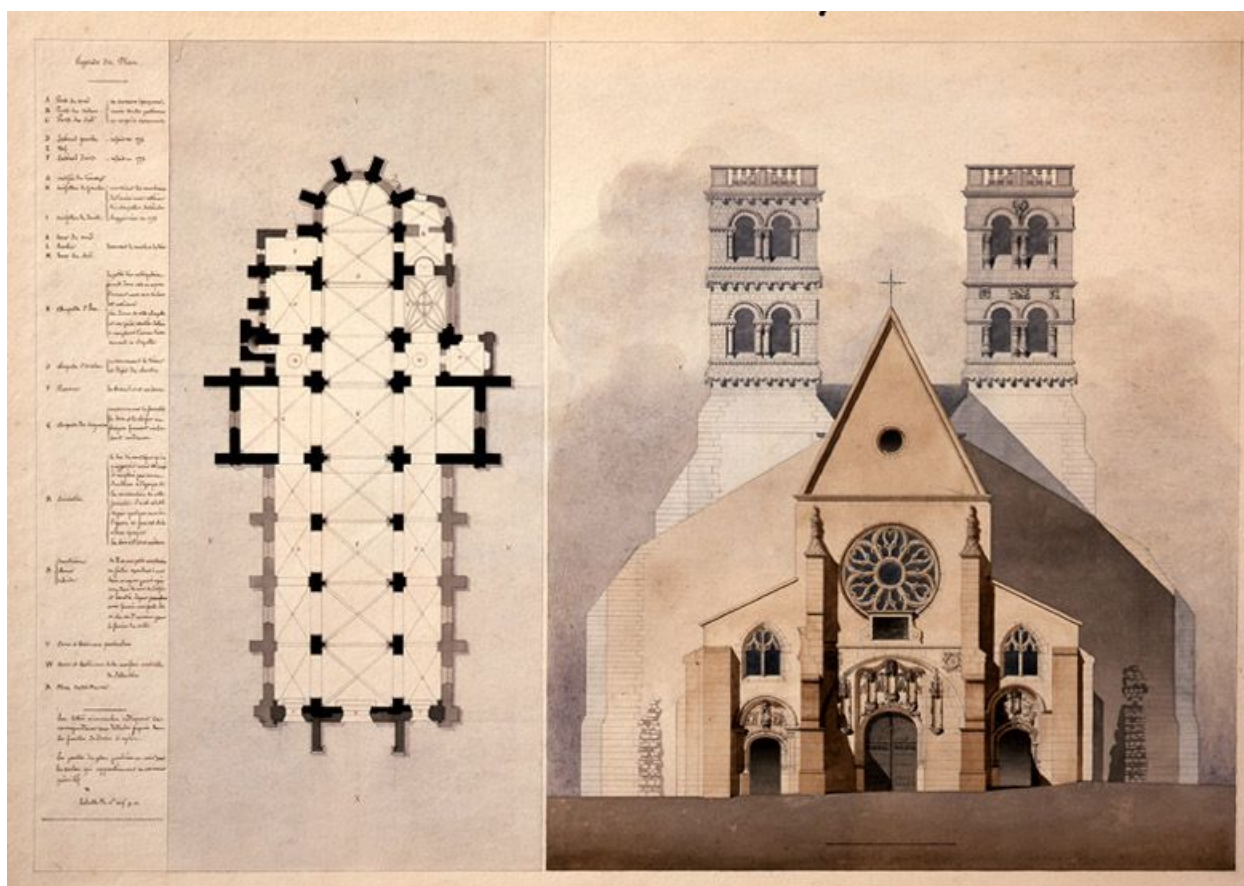
Plan et élévation de la collégiale avant la restauration de Millet. Papier aquarellé. (Musée municipal de Melun. inv. 970.17.2)
