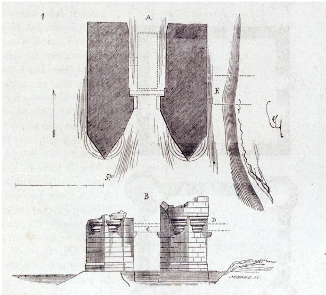
Relevé des deux piles du moulin datant du Moyen Age, publié par Viollet-le-Duc environ trente ans après leur disparition. Gravure. Tiré de : Dictionnaire raisonné de l'architecture française du XIe au XVIe siècle / E. Viollet-Le-Duc, article moulin. Paris, 1868. (BM Melun. 8° 311)
