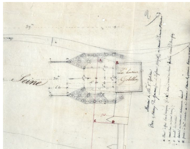
Plan des piles du moulin, 28 mars 1836. (AD Seine-et-Marne. 3 S 115) Phot. Philippe Ayraut, Autr. J.J. (architecte de la ville) Gilson IVR11_20067700375XA
