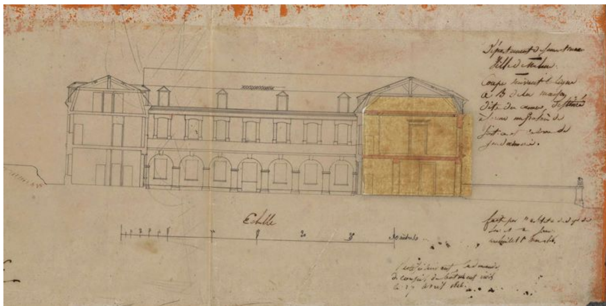
« Coupe sur les ailes en retour et élévation sur le cloître », 11 mars 1816. (AD Seine-et-Marne. 4 N 94)
