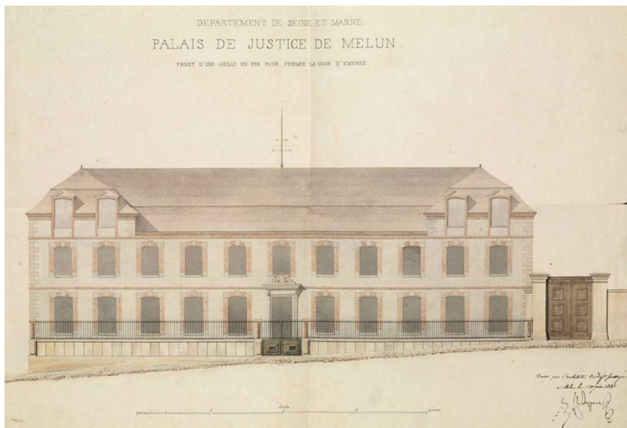
« Palais de justice de Melun. Projet d'une grille en fer pour fermer la cour d'entrée », 10 juin 1841. (AD Seine-et-Marne. 4 N 95)
