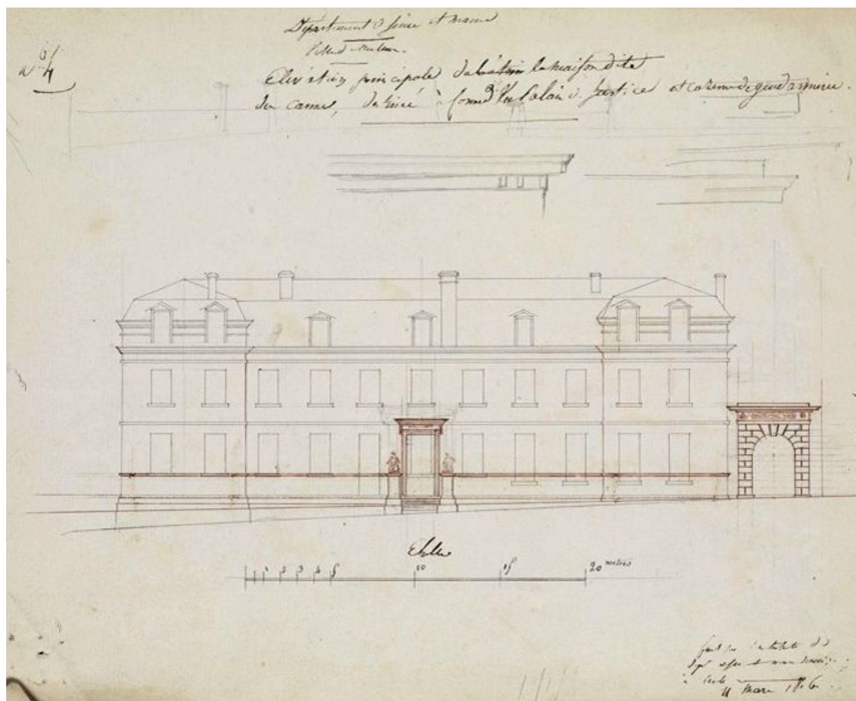
« Elévation principale de la maison dite des Carmes, destinée à former un palais de justice et caserne de gendarmerie », 11 mars 1816. (AD Seine-et-Marne. 4 N 94)
