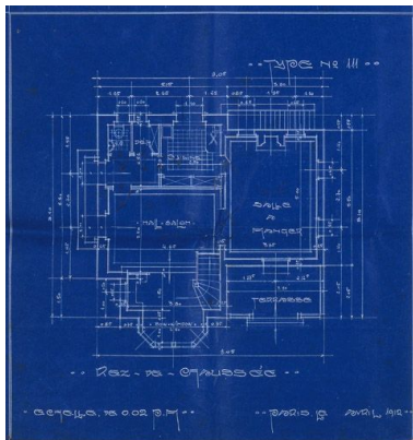
Maison du type 111 : plan du rez-de-chaussée. (Société coopérative ""Paris-Jardins"" de Draveil, dossier 179) Phot. Philippe , Autr. Jean (architecte) Walter IVR11_20069100929XA
