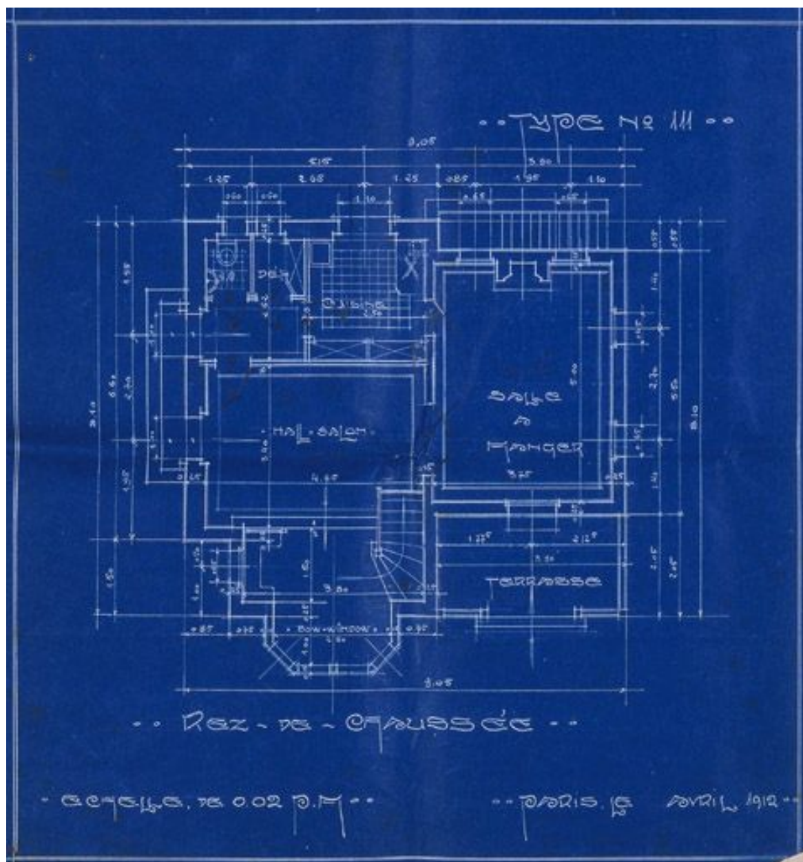
Maison du type 111 : plan du rez-de-chaussée. (Société coopérative ""Paris-Jardins"" de Draveil, dossier 179)
