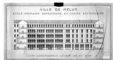
Suite du projet précédent (Doc. 5) : coupe longitudinale. Papier, s.d. (vers 1930). (AM Melun. 1 Fi 1639) Phot. Archives municipales de Melun (reproduction), Autr. Félix (architecte). Boutron IVR11_20047700489NUC
