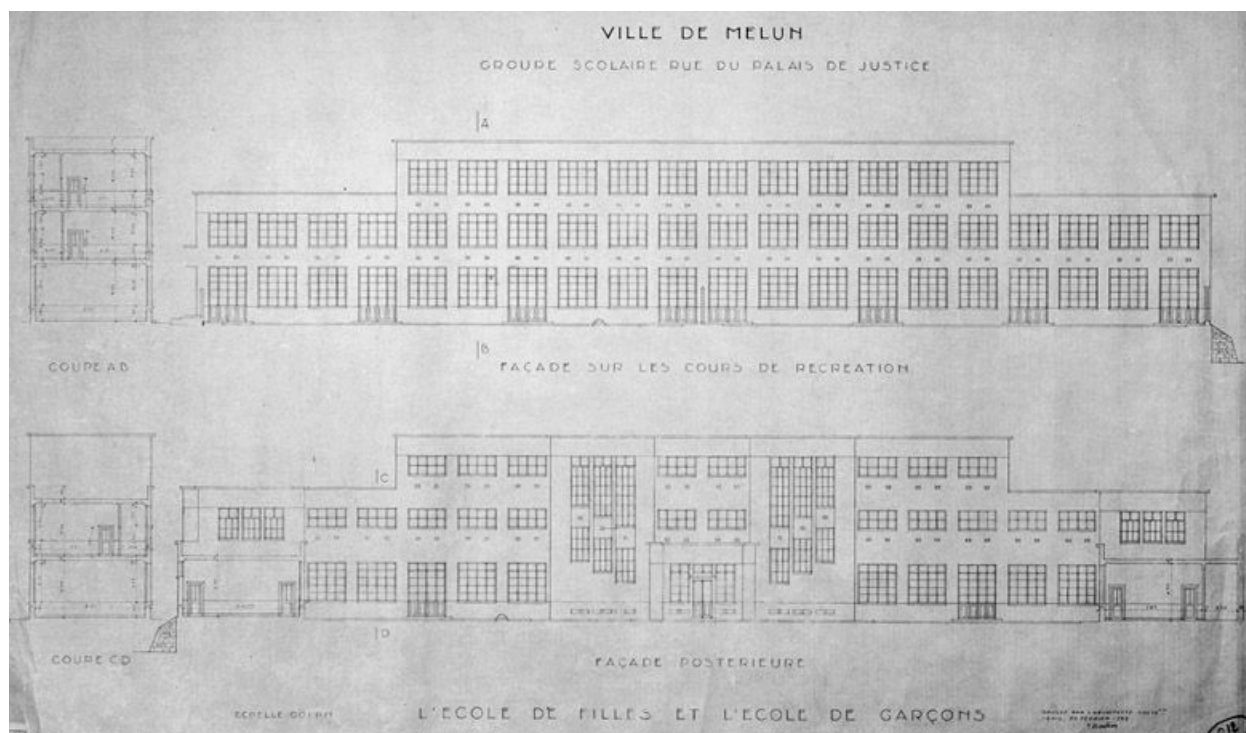
Projet finalement réalisé : élévations sud et nord de l'école primaire. Tirage d'architecte, 1932 (20 février). (AM Melun. 1 Fi 1278)
