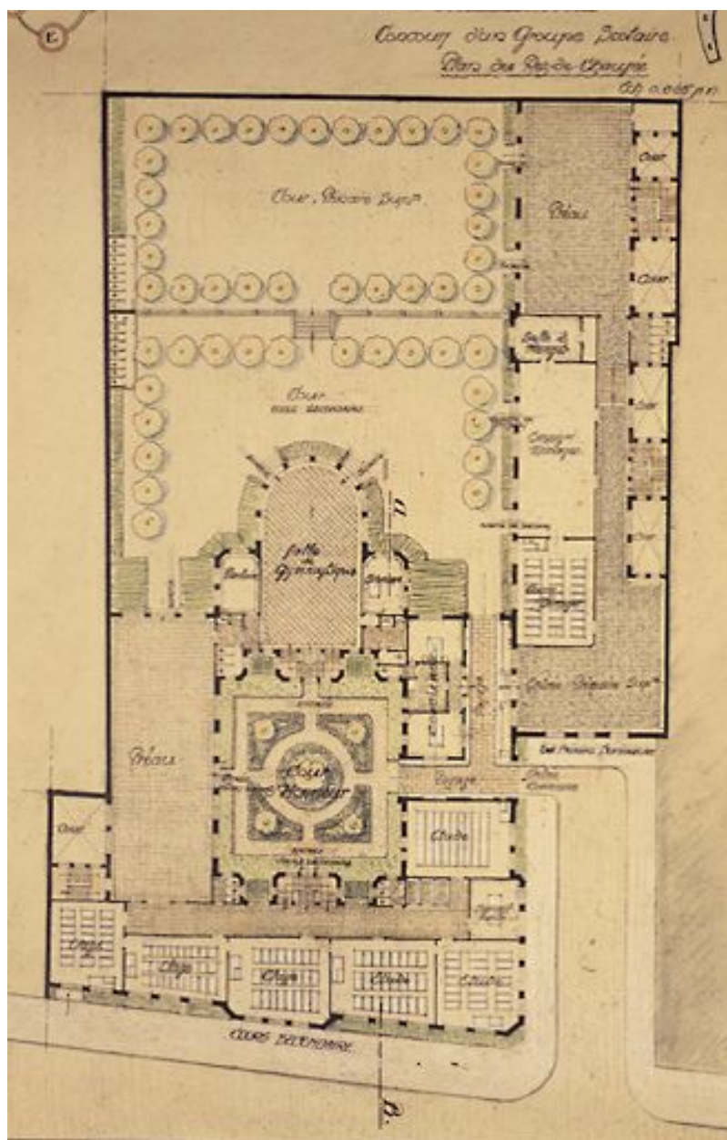
Ville de Melun. Concours d'un groupe scolaire. Plan du rez-de-chaussée. Projet non réalisé pour le groupe scolaire Pasteur, devise : fer à cheval (voir les Doc.2 et 3). Papier aquarellé, s.d. (vers 1930). (AM Melun. 1 Fi 846)
