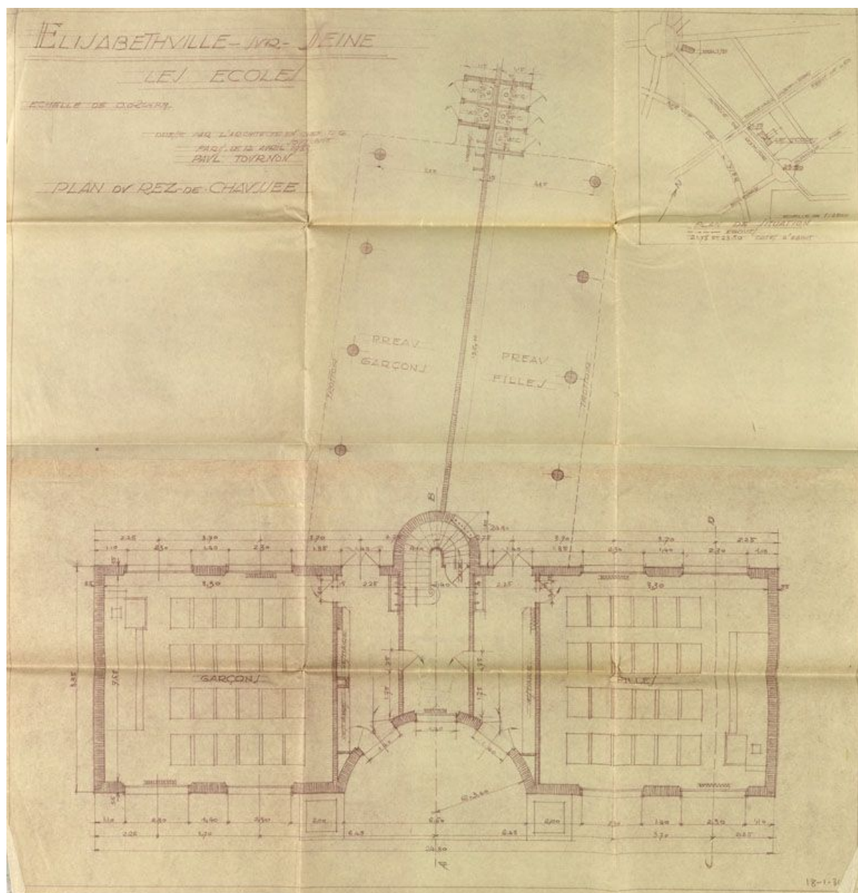
Plan masse de construction de l'Ecole de la Reine Astrid. Tirage, 1929. (AM Aubergenville).
