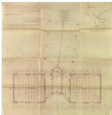
Plan masse de construction de l'Ecole de la Reine Astrid. Tirage, 1929. (AM Aubergenville). Phot. Laurent Kruszyk IVR11_20137800185NUC4A
