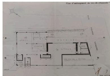
PLan d'aménagement du rez de chaussée, extrait du permis de construire. Phot. Hervé, Michel, Marie Baley IVR11_20169200293NUC4A
