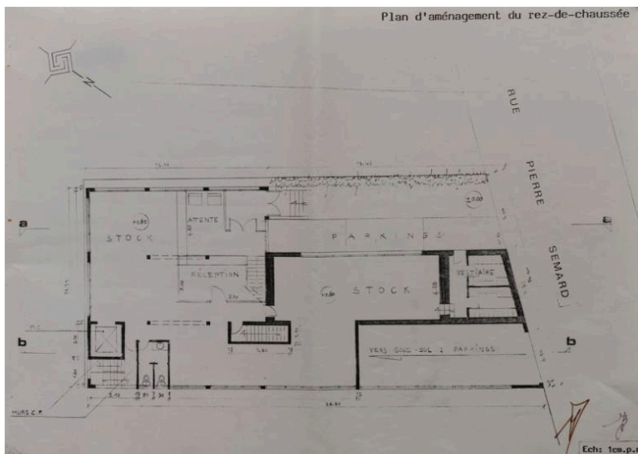
Plan d'aménagement du rez de chaussée, extrait du permis de construire.
