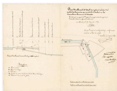
Plan et coupe du moulin des tanneries en 1839. (AD78 7s 285) IVR11_20187800003NUC4A
