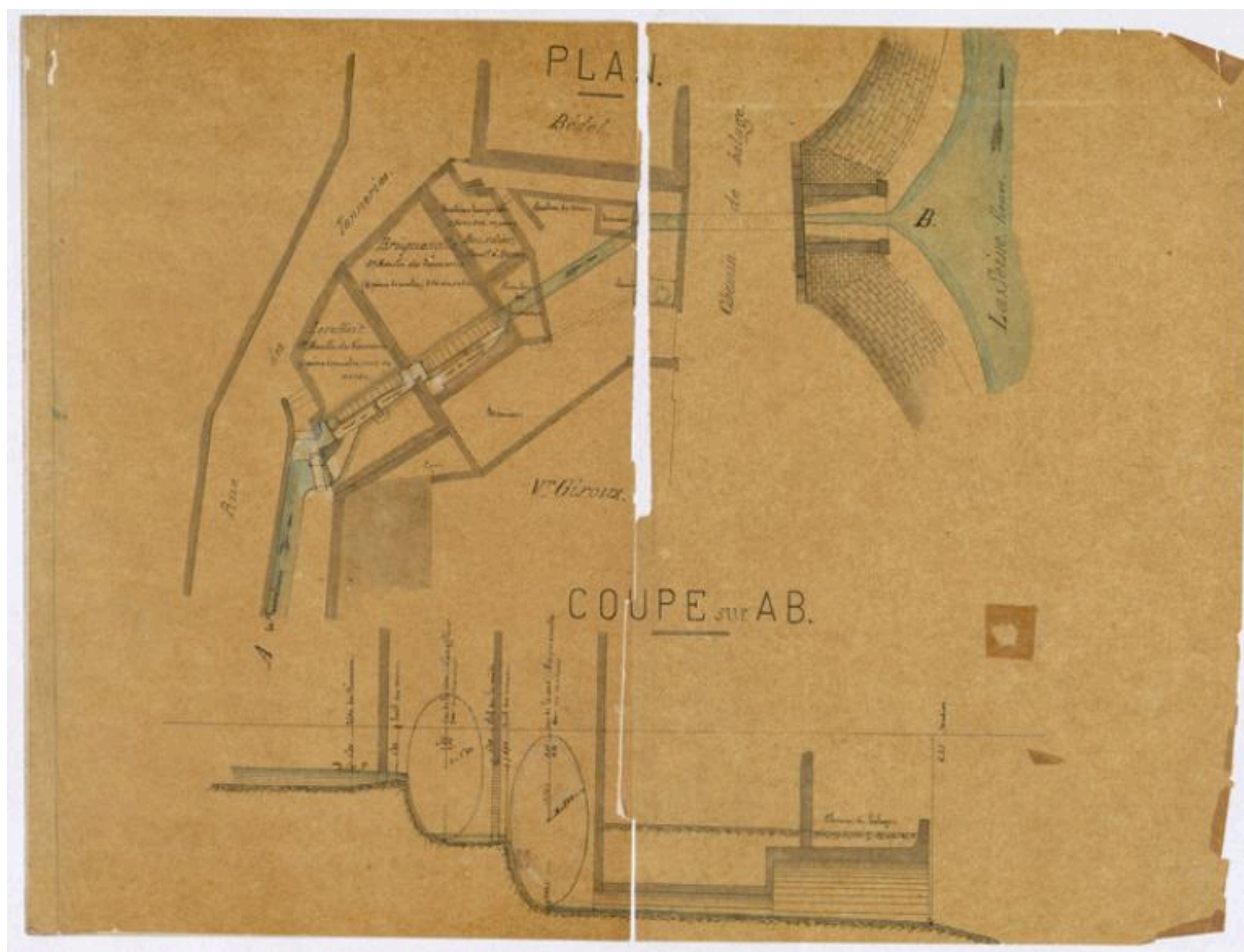
Les deux moulins des tanneries en 1875. Ils appartiennent à M. Lereffait pour le premier et à M. Briquenolle pour le deuxième. (AD 78 7S 285).
