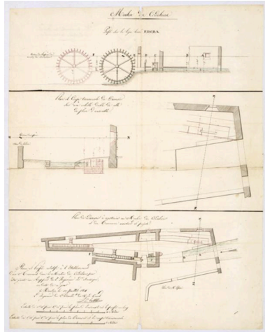
Le nouveau moulin des Cordeliers, plan et coupes.1821 (AD78 7s 285) IVR11_20187800006NUC4A
