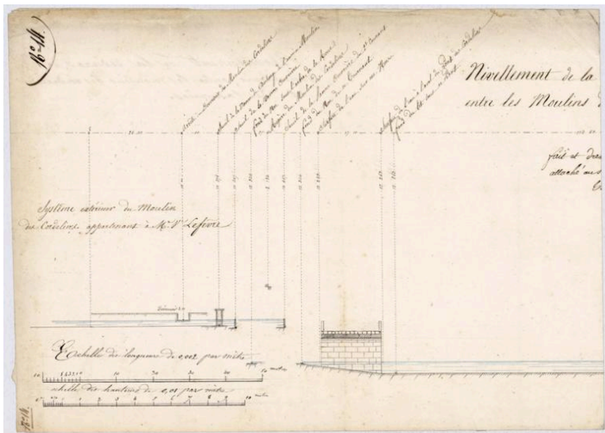
Nivellement de la Vaucouleurs en 1830. Partie gauche. (AD78 7s 285)
