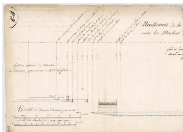
Nivellement de la Vaucouleurs en 1830. Partie gauche. (AD78 7s 285) IVR11_20187800014NUC4A
