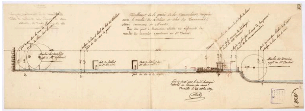
Nivellement de la Vaucouleurs entre le moulin des Cordeliers et le moulin des Tanneries. 1839. (AD78 7s 285)
