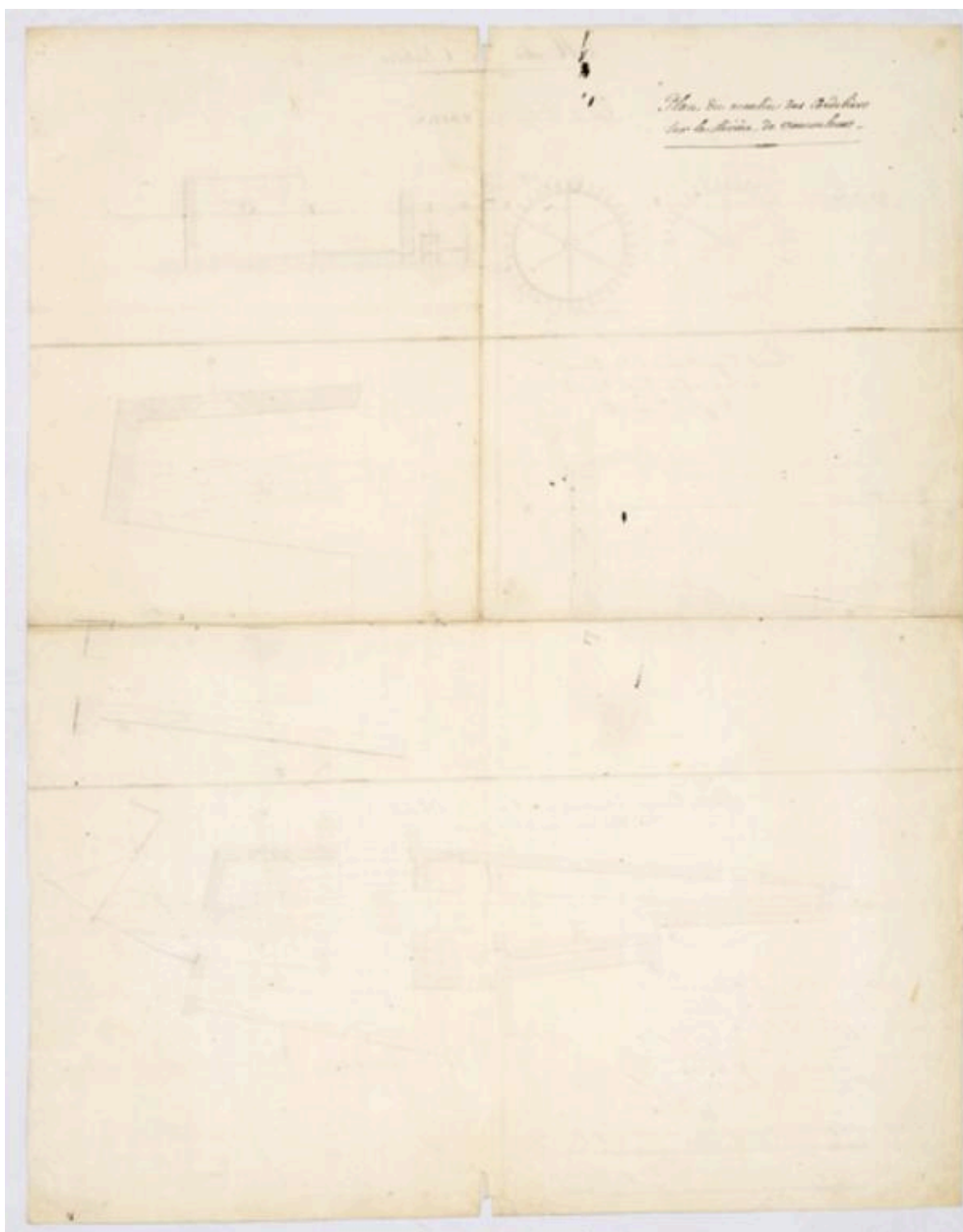
Le nouveau moulin des Cordeliers, plan et coupes.1821. Verso. (AD78 7s 285)
