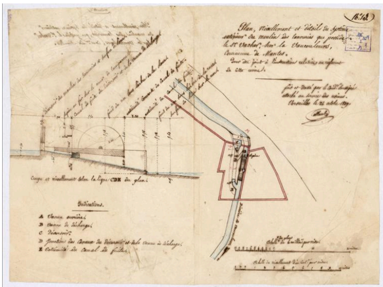
Plan du moulin des Tanneries en 1839. (AD78 7s 285)
