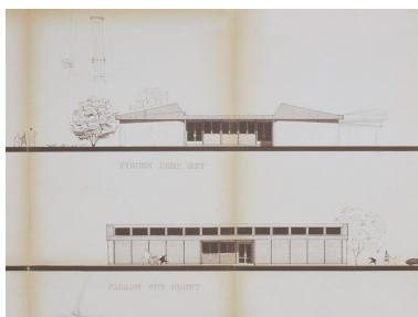
Projet Geep industrie, détail de la façade sud-ouest et du pignon nord-est. (AM Vigneux-sur-Seine, 1 M 122) Autr. Paul (architecte, urbaniste) Chemetov, Autr. Jean (architecte) Deroche IVR11_20079101171XA
