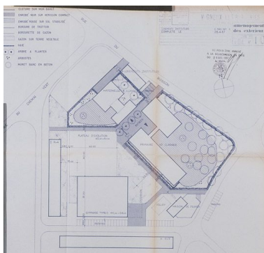
Plan d'aménagement des extérieurs, dressé par P. Chemetov et J. Deroche, 27 février 1967. (AM Vigneux-sur-Seine, 1 M 119) Autr. Paul (architecte, urbaniste) Chemetov, Autr. J. (architecte) Deroche IVR11_20079101165XA
