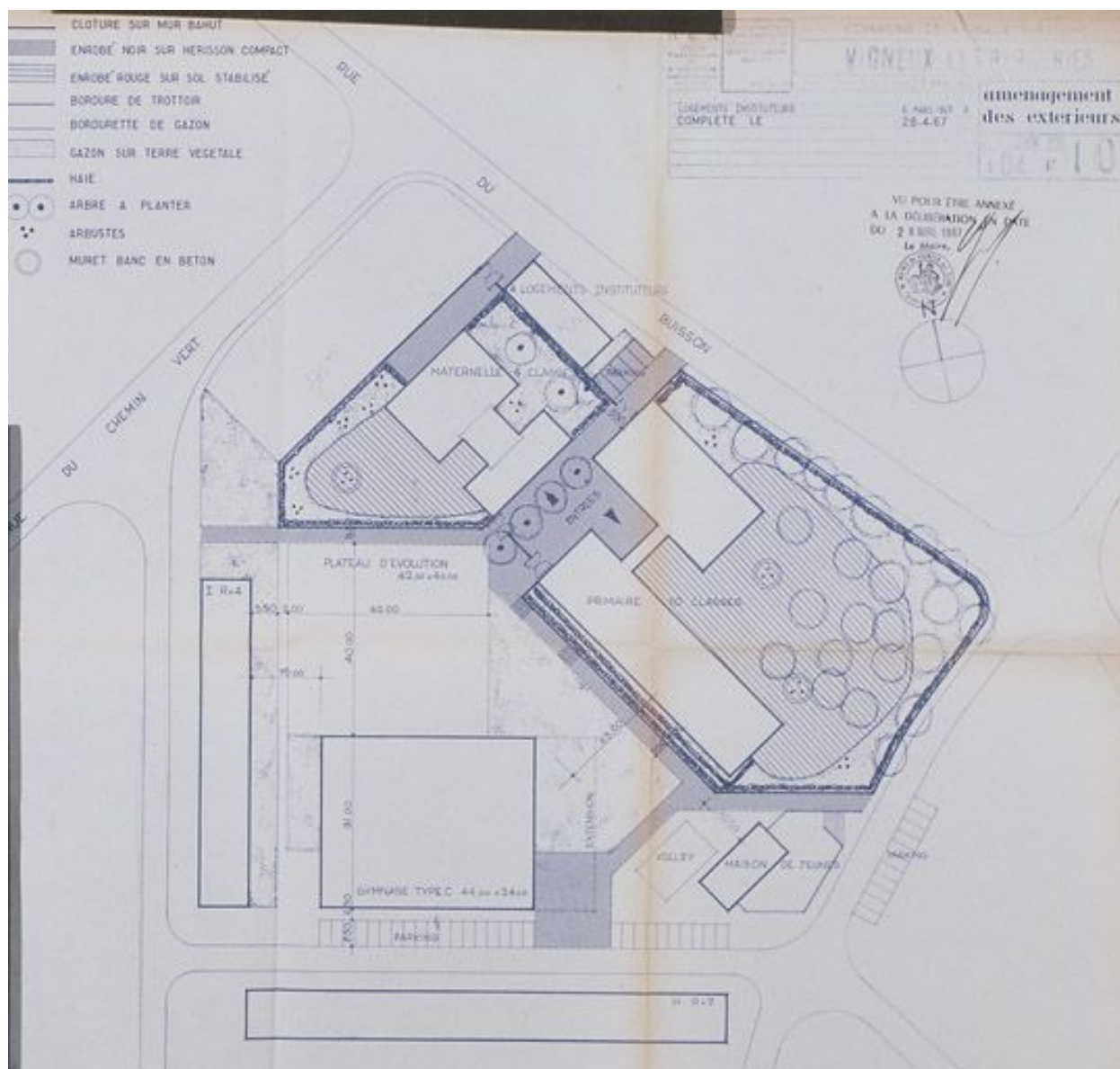
Plan d'aménagement des extérieurs, dressé par P. Chemetov et J. Deroche, 27 février 1967. (AM Vigneux-sur-Seine, 1 M 119)
