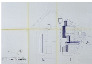
Groupe scolaire Louise-Michel : plan-masse, dressé par P. Chemetov et J. Deroche, 13 novembre 1965. (AM Vigneux-sur-Seine, 1 M 119) IVR11_20079101167XA
