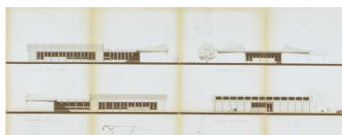
Projet Geep industrie, façades nord-ouest, sud-est, sud-ouest et du pignon nord-est. (AM Vigneux-sur-Seine, 1 M 122) Autr. Paul (architecte, urbaniste) Chemetov, Autr. Jean (architecte) Deroche IVR11_20079101173XA
