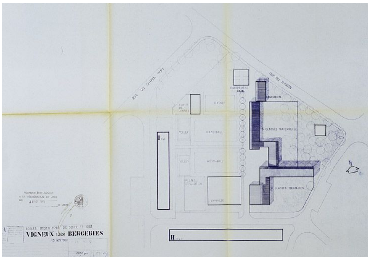
Groupe scolaire Louise-Michel : plan-masse, dressé par P. Chemetov et J. Deroche, 13 novembre 1965. (AM Vigneux-sur-Seine, 1 M 119)
