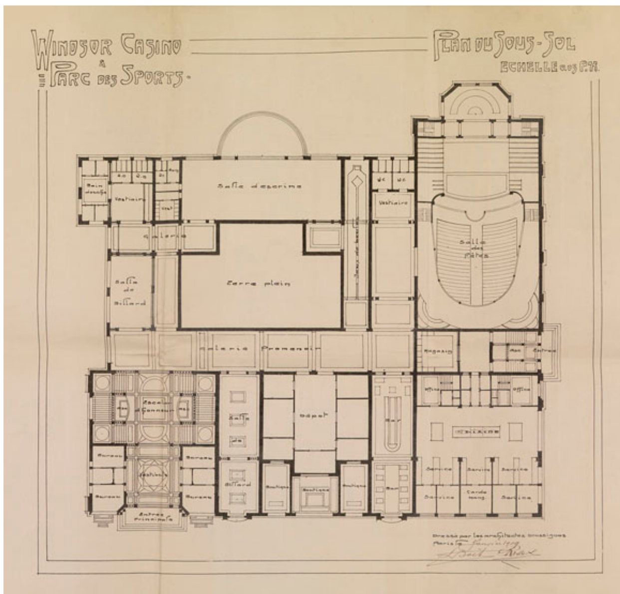
Plan du sous-sol du casino, 1909. (AM Enghien-les-Bains, Fonds des autorisations de permis de construire)
