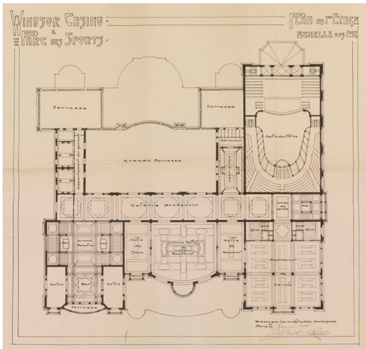
Plan du premier étage, 1909. (AM Enghien-les-Bains, Fonds des autorisations de permis de construire)
