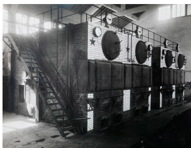
Les chaudières. (Archives de l'Assistance publique, 3 Fi 3/20) Autr. Indus-Photos Demeure J. IVR11_20089100137NUC4AB
