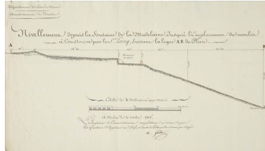
Profil annexé à la demande d'installation d'un moulin formulée par François Lecoq, en 1815. (AD Seine-et-Marne, 3S97/1) Repro. Yvan Bourhis IVR11_20097701589NUC2A
