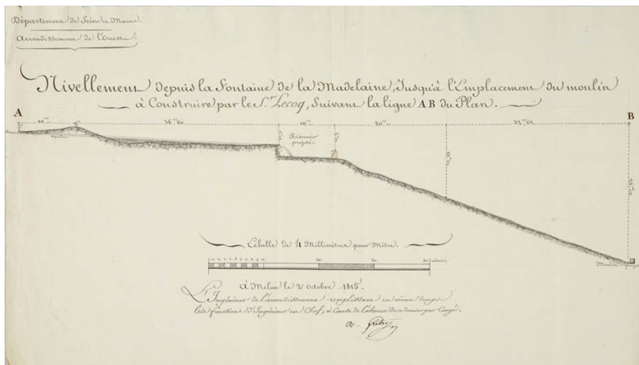
Profil annexé à la demande d'installation d'un moulin formulée par François Lecoq, en 1815. (AD Seine-et-Marne, 3S97/1)
