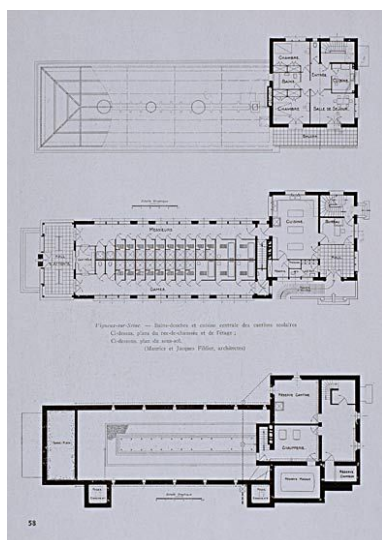
Plans des différents niveaux. (AD Essonne) IVR11_20059101673XA
