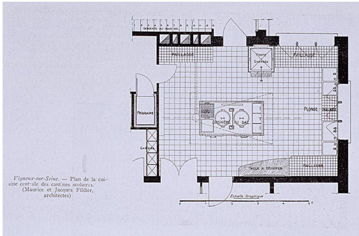
Plan de la cuisine. (AD Essonne)
