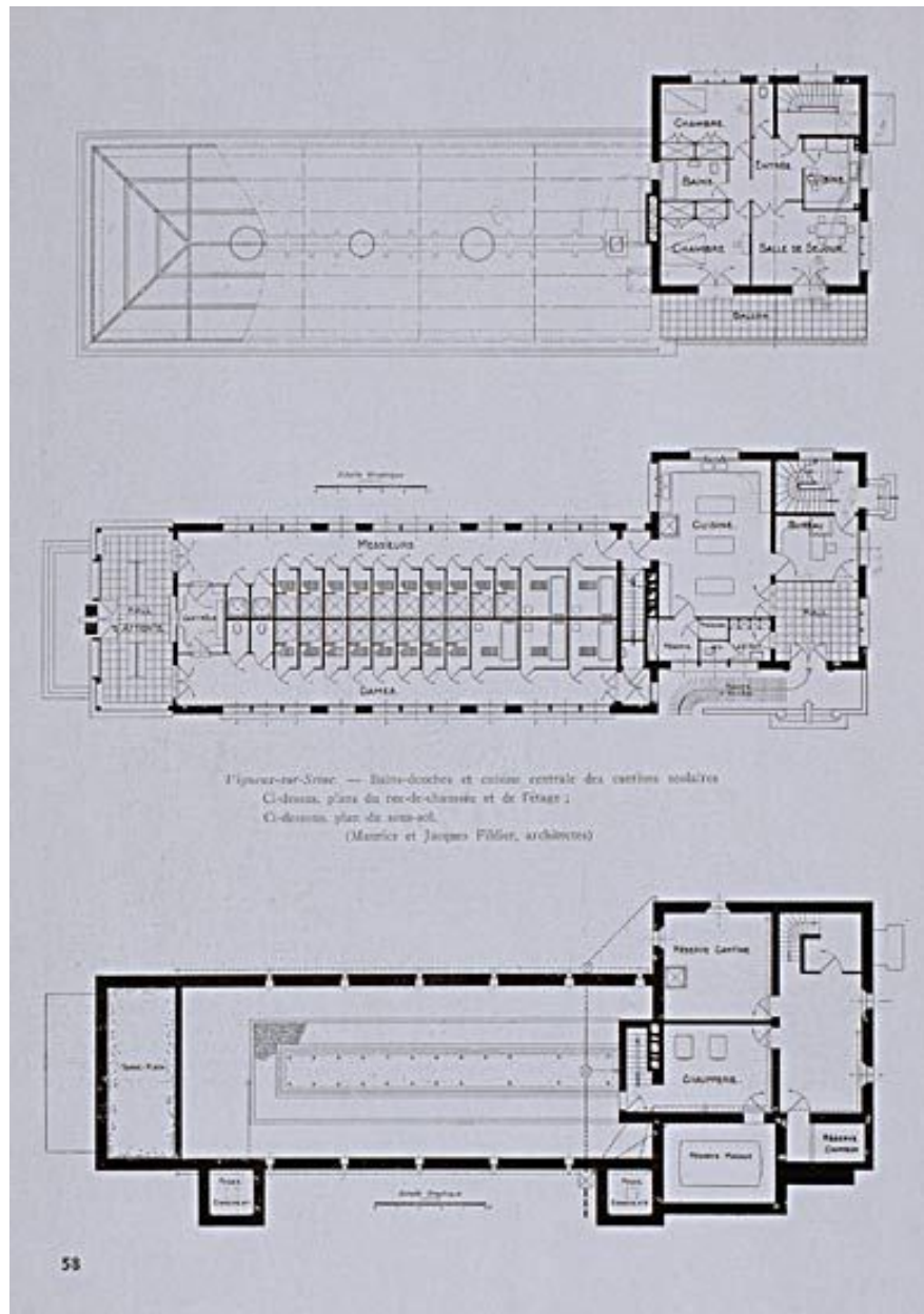
Plans des différents niveaux. (AD Essonne)
