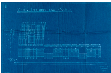
Projet d'élévation de façade, 1927. (AM Enghien-les-Bains, M14) Phot. Jean-Bernard Vialles, Autr. Henri (architecte) Moreels IVR11_20099500096NUC4A
