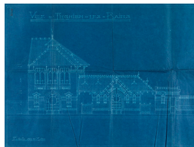
Second projet d'élévation de façade, 1927. (AM Enghien-les-Bains, M14) Phot. Jean-Bernard Vialles, Autr. Henri (architecte) Moreels IVR11_20099500095NUC4A
