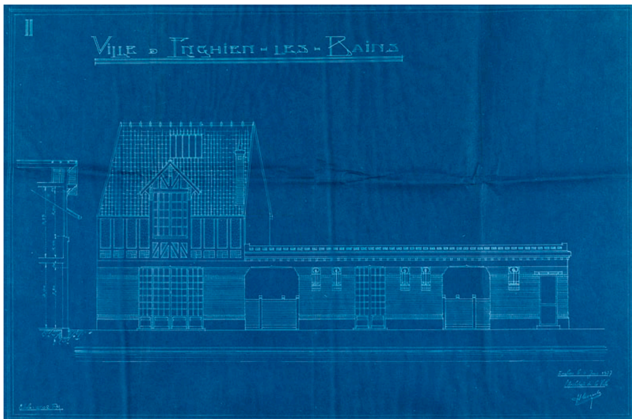
Projet d'élévation de façade, 1927. (AM Enghien-les-Bains, M14)
