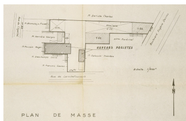
Plan accompagnant une demande de permis de construire : "Projet de construction de 2 hangars préfabriqués", plan-masse, 1962 (Ville des Lilas, Permis de construire 1961-3). IVR11_20059300420XA
