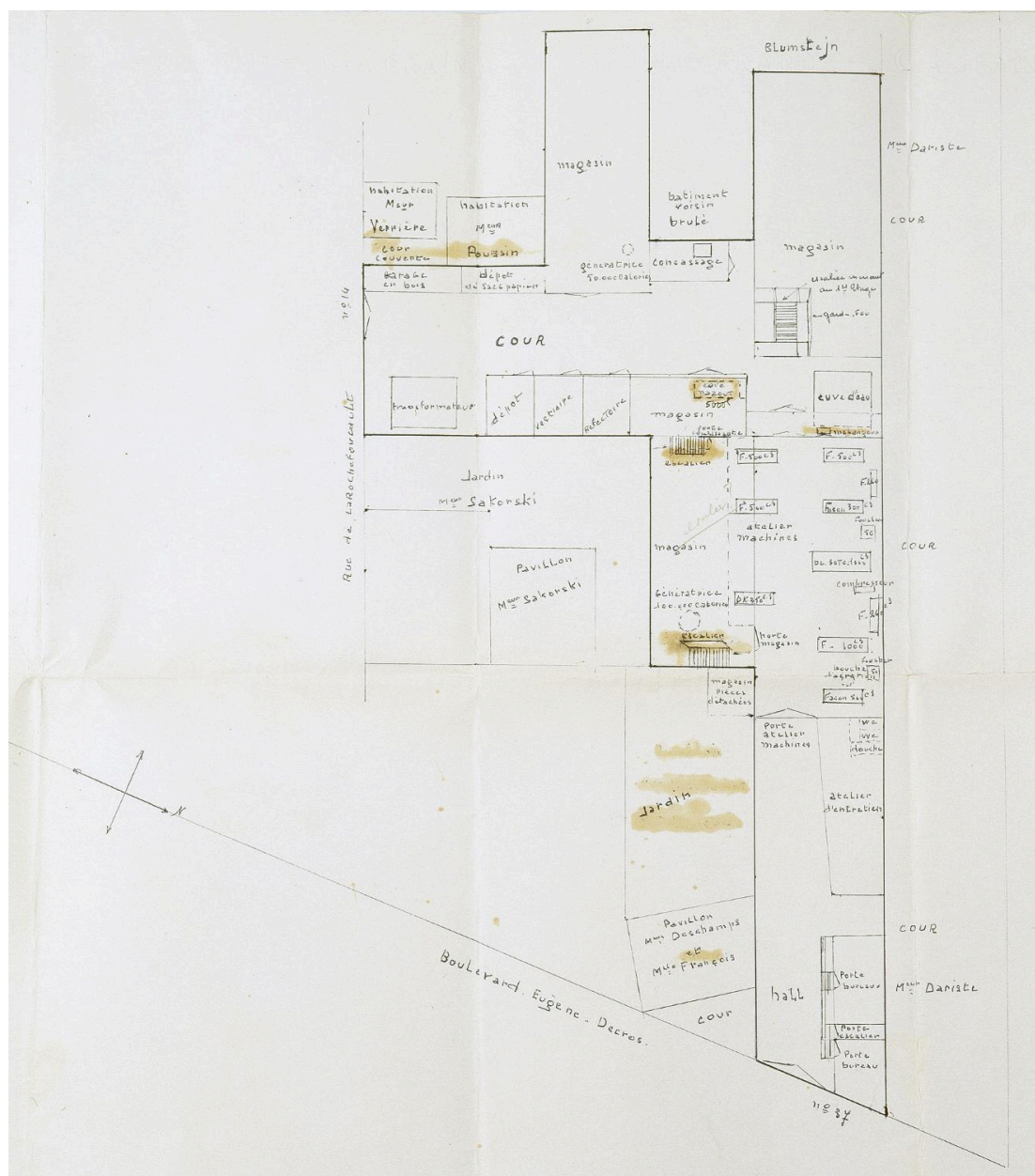
Plan-masse indiquant la fonction des ateliers, 1966 (AD93 1322 W 261).
