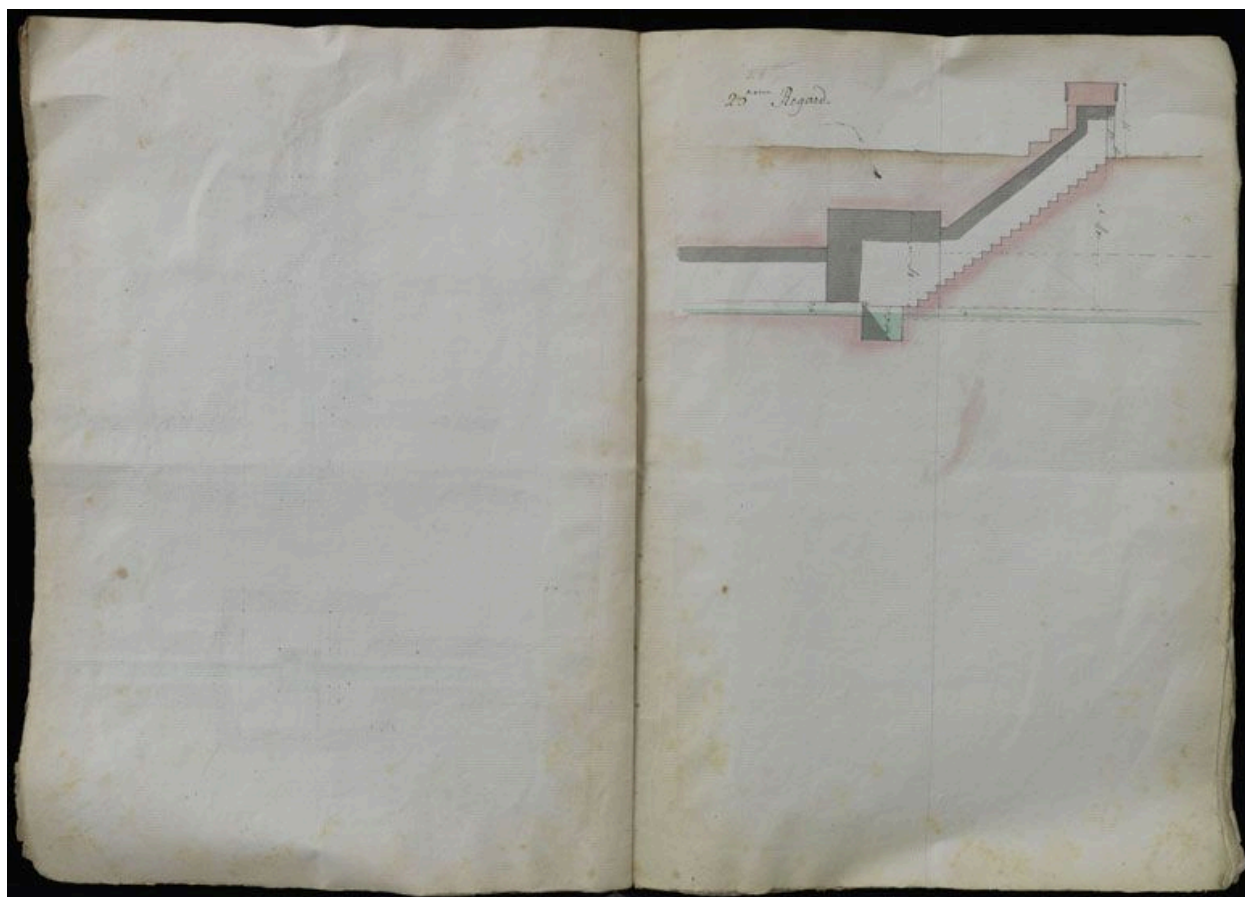
Paris 14e. Coupe du regard XXV. Plans, 1765-1789. (Bibliothèque de l'Ecole de Nationale des Ponts et Chaussées, Ms.2567 -vol 2)
