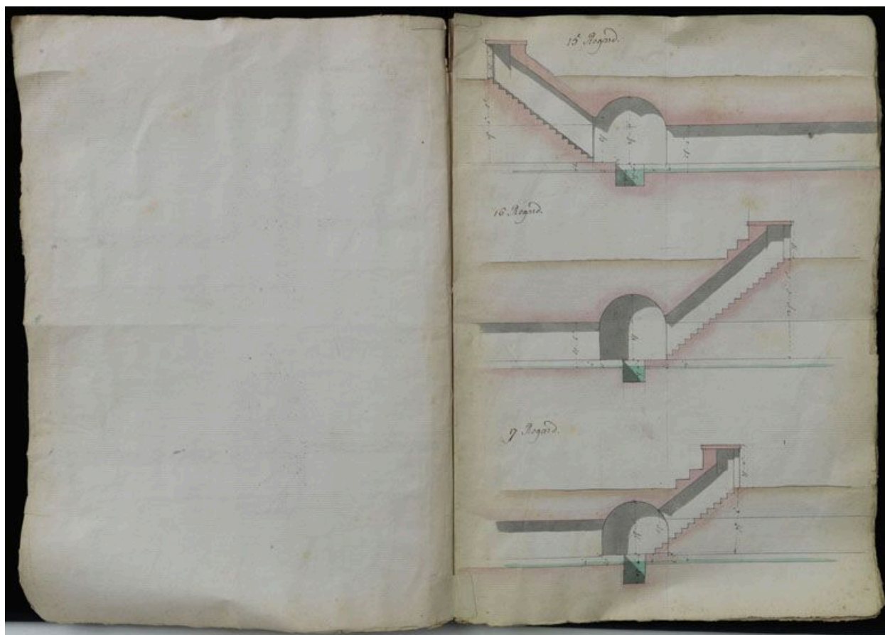
Arcueil. Coupes des regards XV, XVI et XVII. Plans, 1765-1789. (Bibliothèque de l'Ecole de Nationale des Ponts et Chaussées, Ms.2567 -vol 2)
