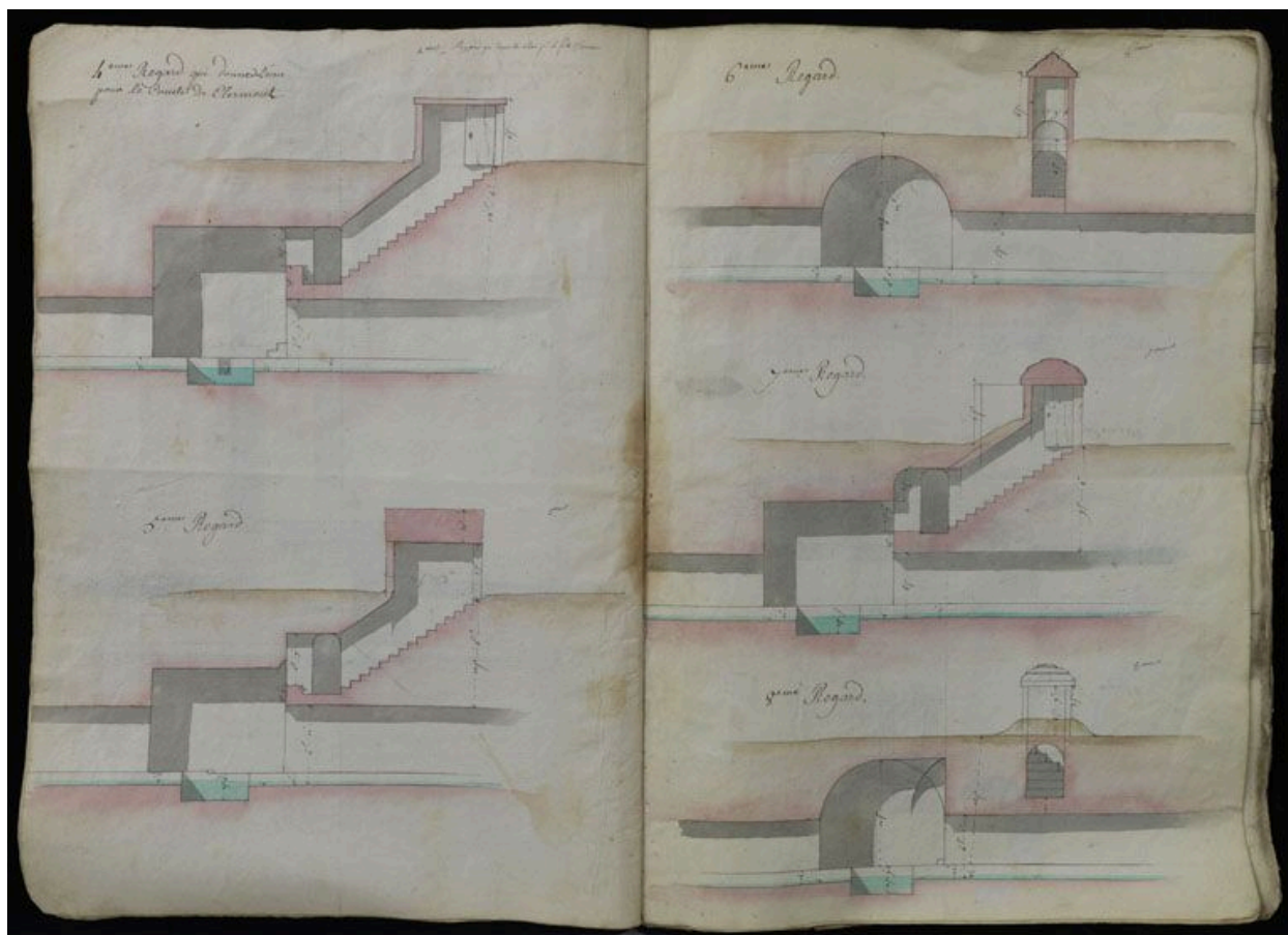
Fresnes, Haÿ-les-Roses (L'). Coupes des regards IV, V, VI, VII et VIII . Plans, 1765-1789. (Bibliothèque de l'Ecole de Nationale des Ponts et Chaussées, Ms.2567 -vol 2)
