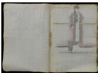
Fresnes. Coupe du regard III. Plans, 1765-1789. (Bibliothèque de l'Ecole de Nationale des Ponts et Chaussées, Ms.2567 -vol 2) Phot. Laurent Kruszyk IVR11_20129400261NUC4A
