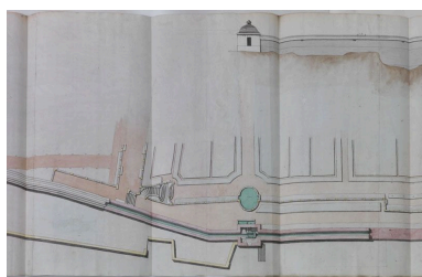
Arcueil. Coupe et plan de la concession d'eau à Arcueil partant du regard XIII desservant un bassin et une fontainer (18e siècle). (Bibliothèque de l'Ecole de Nationale des Ponts et Chaussées, Ms.2783) Phot. Laurent Kruszyk IVR11_20129400253NUC4A
