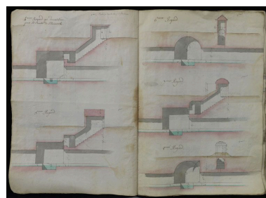
Fresnes, Haÿ-les-Roses (L'). Coupes des regards IV, V, VI, VII et VIII. Plans, 1765-1789. (Bibliothèque de l'Ecole de Nationale des Ponts et Chaussées, Ms.2567 -vol 2) Phot. Laurent Kruszyk IVR11_20129400262NUC4A
