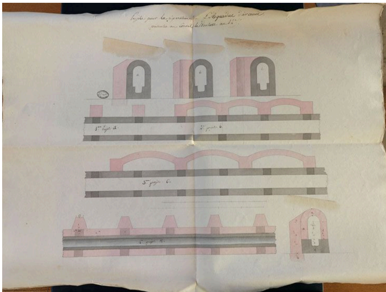
Arcueil. Coupe de la galerie pour réparation fin XVIIe siècle début XIXe siècle. (AN, F/13/1004)
