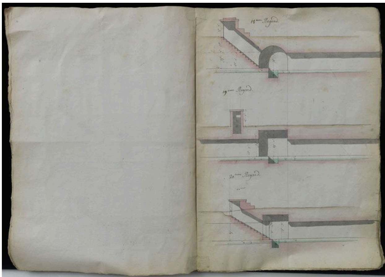
Arcueil, Gentilly. Coupes des regards XVIII, XIX et XX. Plans, 1765-1789. (Bibliothèque de l'Ecole de Nationale des Ponts et Chaussées, Ms.2567 -vol 2)
