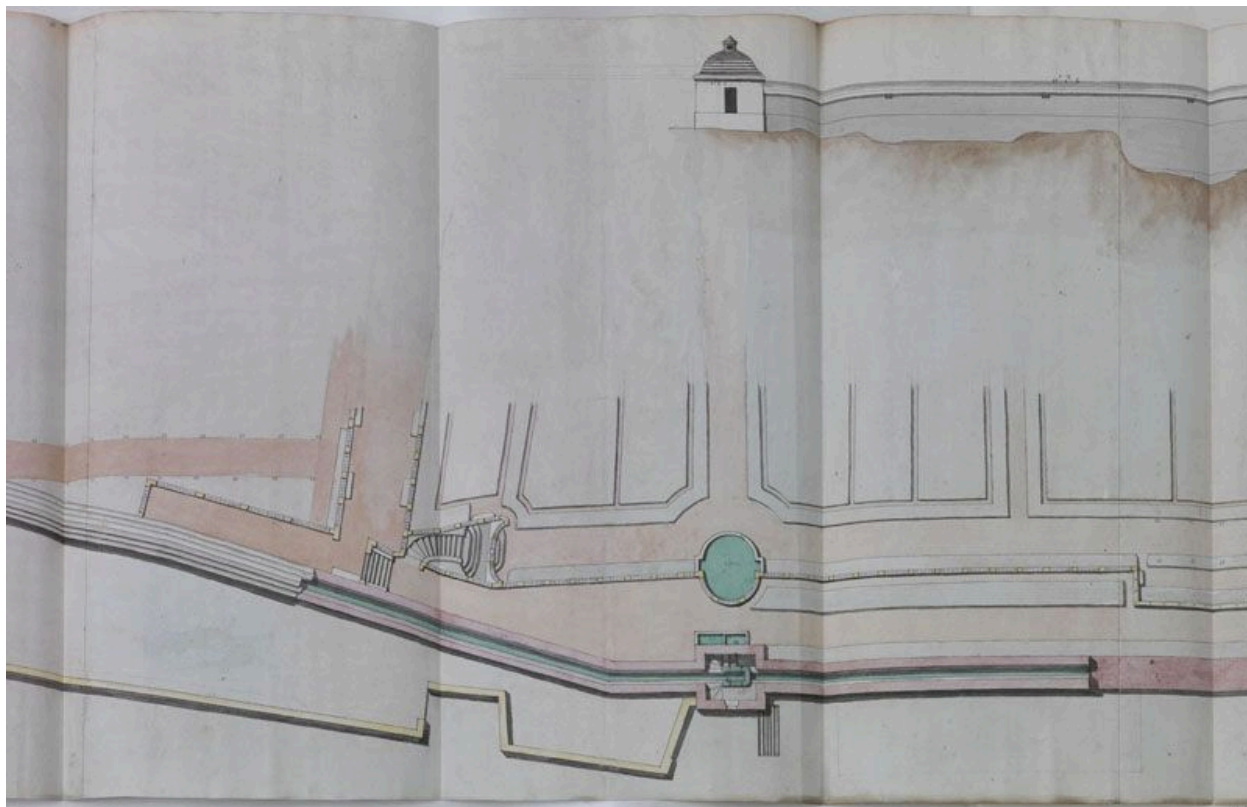
Arcueil. Coupe et plan de la concession d'eau à Arcueil partant du regard XIII desservant un bassin et une fontainer (18e siècle). (Bibliothèque de l'Ecole de Nationale des Ponts et Chaussées, Ms.2783)
