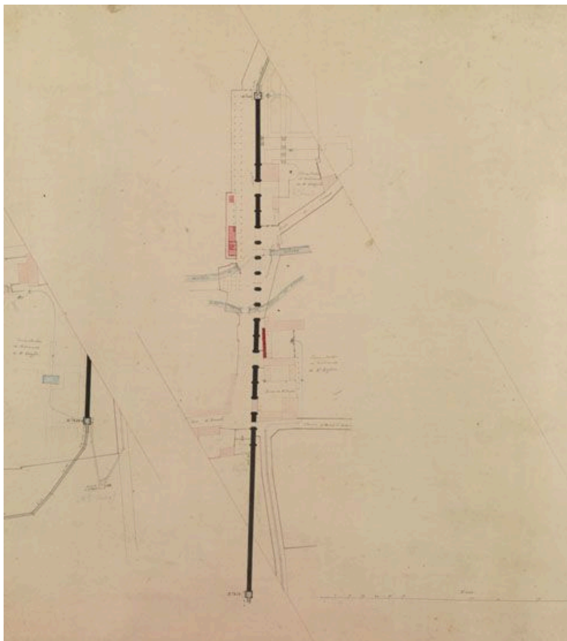
Arcueil, Cachan. Plan détaillé de l'aqueduc Médicis vers 1860 : Pont-aqueduc d'Arcueil-Cachan. (Archives de Paris, Plan n°2522)
