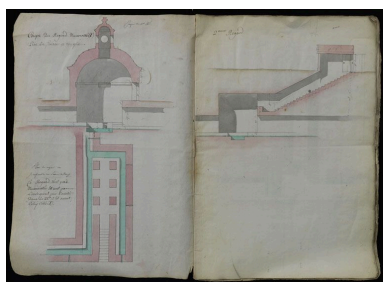
Rungis. Coupe des regards I et II ainsi que du regard des sources. Plans, 1765-1789. (Bibliothèque de l'Ecole de Nationale des Ponts et Chaussées, Ms.2567 -vol 2) Phot. Laurent Kruszyk IVR11_20129400260NUC4A
