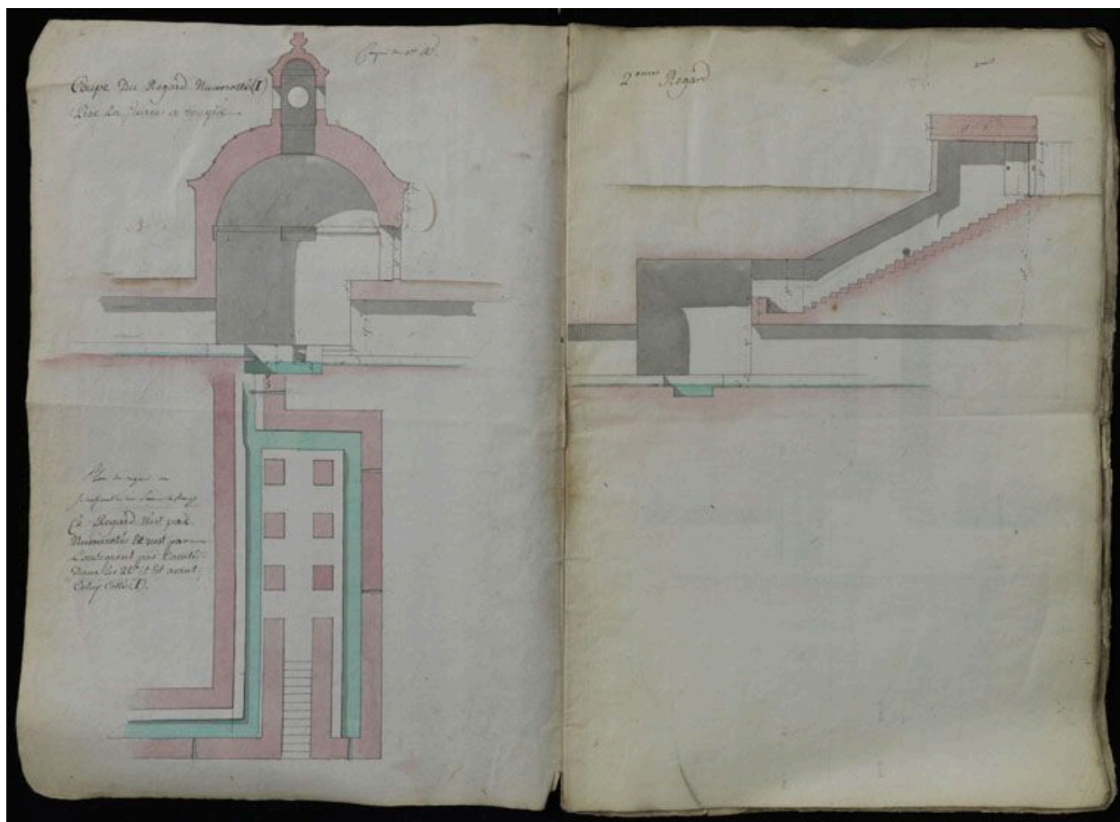
Rungis. Coupe des regards I et II ainsi que du regard des sources. Plans, 1765-1789. (Bibliothèque de l'Ecole de Nationale des Ponts et Chaussées, Ms.2567 -vol 2)
