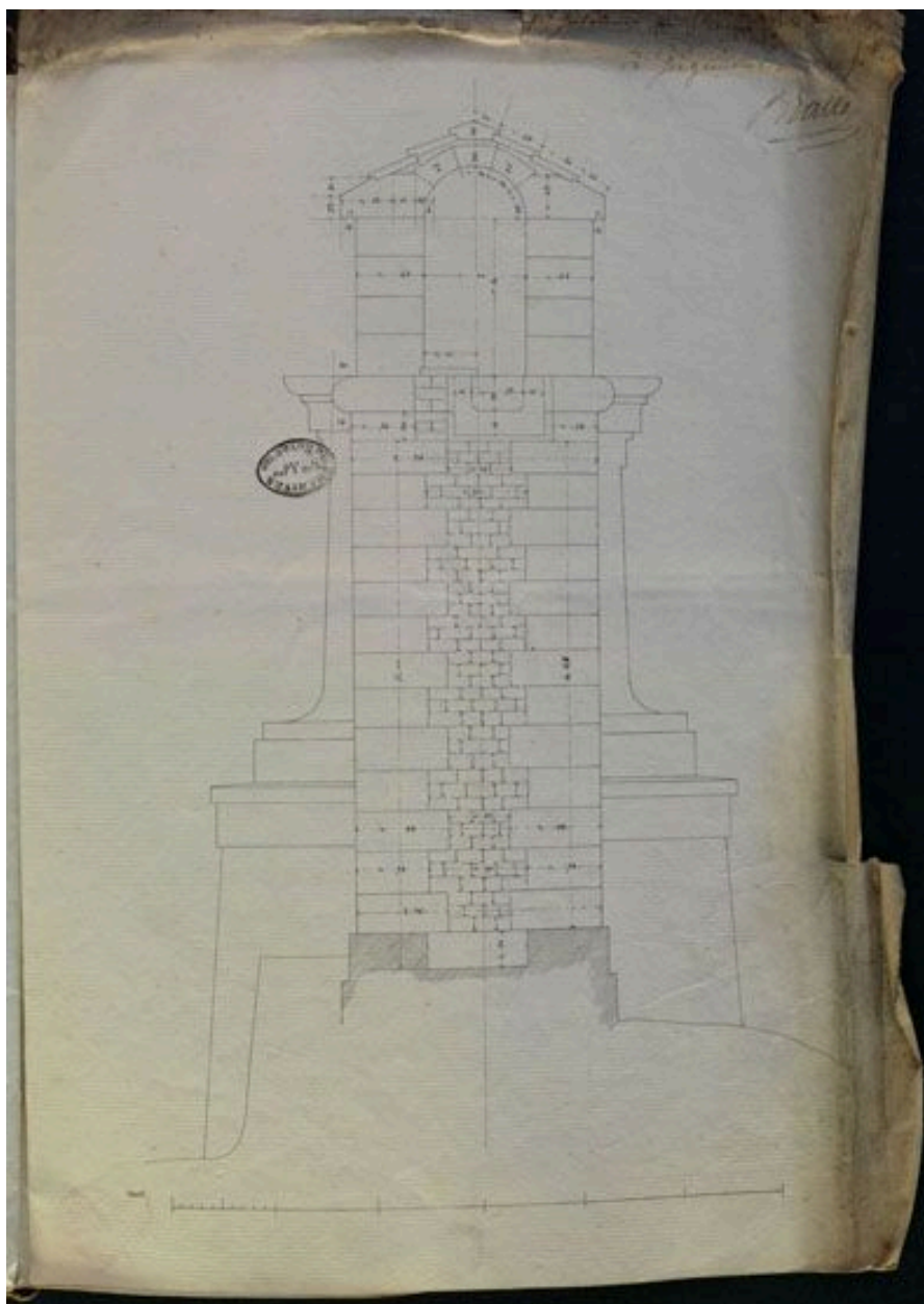
Arcueil. Elevation du pont-aqueduc au XIXe siècle. (AN, F/13/1004)
