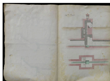
Paris 14e. Coupe et plan du regard XXIV. Plans, 1765-1789. (Bibliothèque de l'Ecole de Nationale des Ponts et Chaussées, Ms.2567 -vol 2) Phot. Laurent Kruszyk IVR11_20127501483NUC4A
