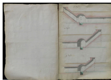
Arcueil. Coupes des regards XV, XVI et XVII. Plans, 1765-1789. (Bibliothèque de l'Ecole de Nationale des Ponts et Chaussées, Ms.2567 -vol 2) Phot. Laurent Kruszyk IVR11_20129400265NUC4A
