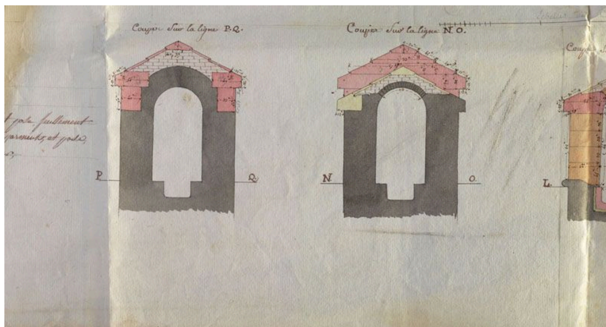
Arcueil. Coupe de la galerie pour réparation fin XVIIe siècle début XIXe siècle. (AN, F/13/1004)
