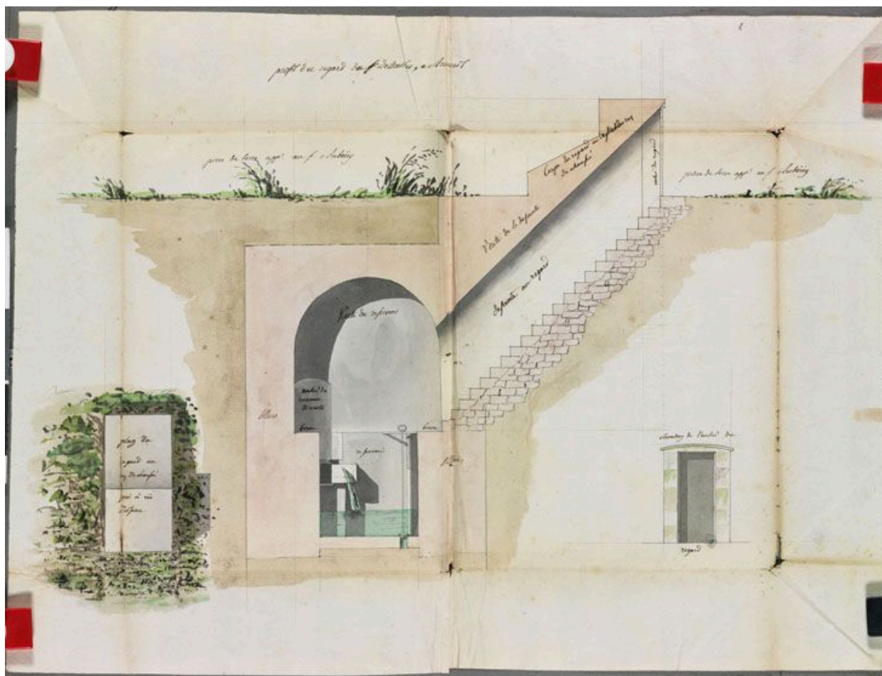
Arcueil. Coupe d'un regard de concession. (AN, O/1/1599)
