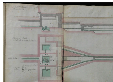
Paris 14e. Plan et coupe du regard XXVI : galerie d'arrivée, bassins de
