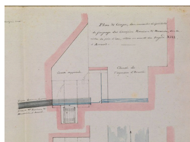
Arcueil. Coupe d'un regard de concession, en amont du regard XIII à Arcueil. (Archives de Paris, VO3-137)
