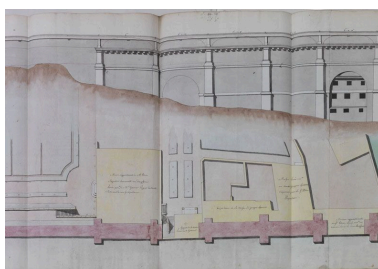
Arcueil. Elévation et plan du pont-aqueduc d'Arcueil avec les noms des propriétés jouxtant l'édifice (18e siècle). (Bibliothèque de l'Ecole de Nationale des Ponts et Chaussées, Ms.2783) Phot. Laurent Kruszyk IVR11_20129400254NUC4A
