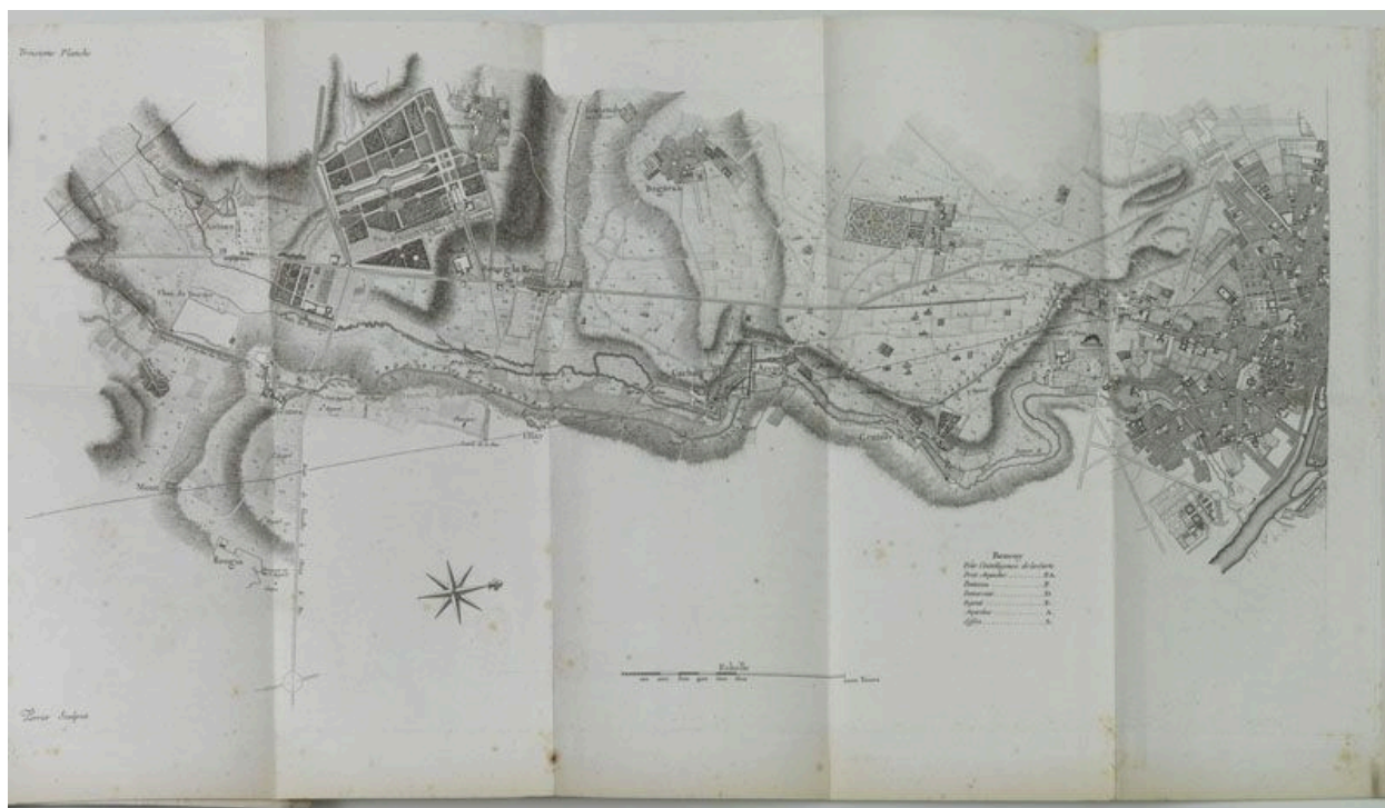
Planche représentant le projet de détournement des eaux de l'Yvette et de la Bièvre pour amener l'eau à Paris . Plans, 1765-1789. (Bibliothèque de l'Ecole de Nationale des Ponts et Chaussées, Ms.2567 )
