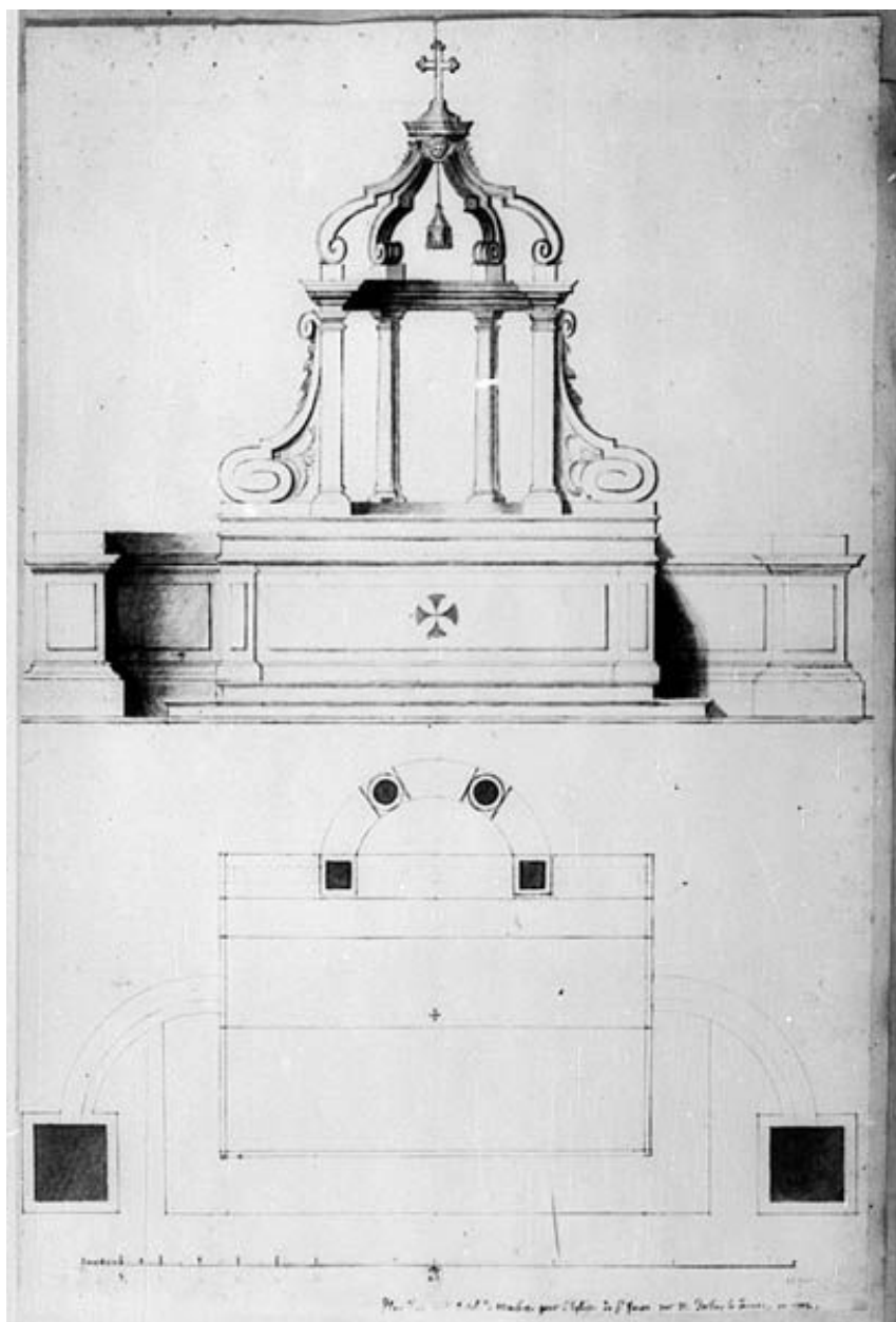
Plan d'un petit autel de marbre pour l'église de St Faron par M. d'Orbay le Jeune en 1702." Dessin, 18e s. (BNF. Département des estampes, TopoVa Seine-et-Marne, H 156277-156283)
