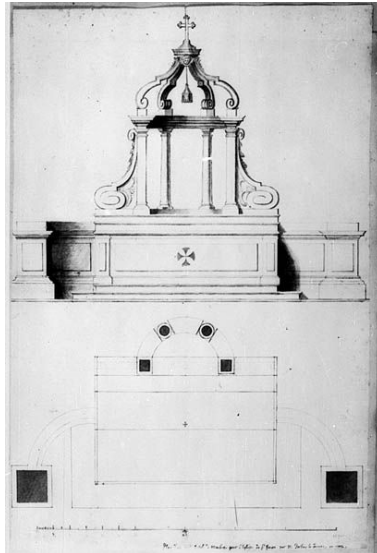
Plan d'un petit autel de marbre pour l'église de St Faron par M. d'Orbay le Jeune en 1702." Dessin, 18e s. (BNF. Département des estampes, TopoVa Seine-et-Marne, H 156277-156283) Phot. Bibliothèque nationale de France IVR11_19807700105Z
