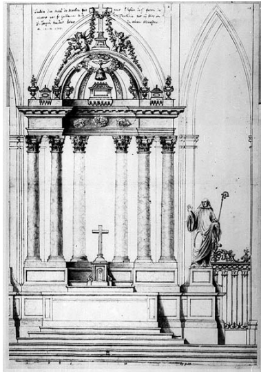
Dessain d'un autel de marbre fait pour l'église de St Faron lès Meaux par frère Guillaume de la Tremblaie, par les soins de D. Jacques Houdart, prieur du même monastère, en janvier 1703." Dessin, 18e s. (BNF. Département des estampes, TopoVa Seine-et-Marne, H 156277-156283) Phot. Bibliothèque nationale de France IVR11_19807700104Z
