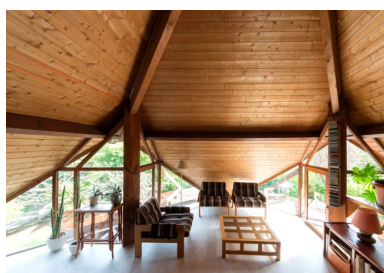
Vue générale de la mezzanine au-dessus de l'espace de séjour. Phot. Laurent Kruszyk IVR11_20179100037NUC4A
