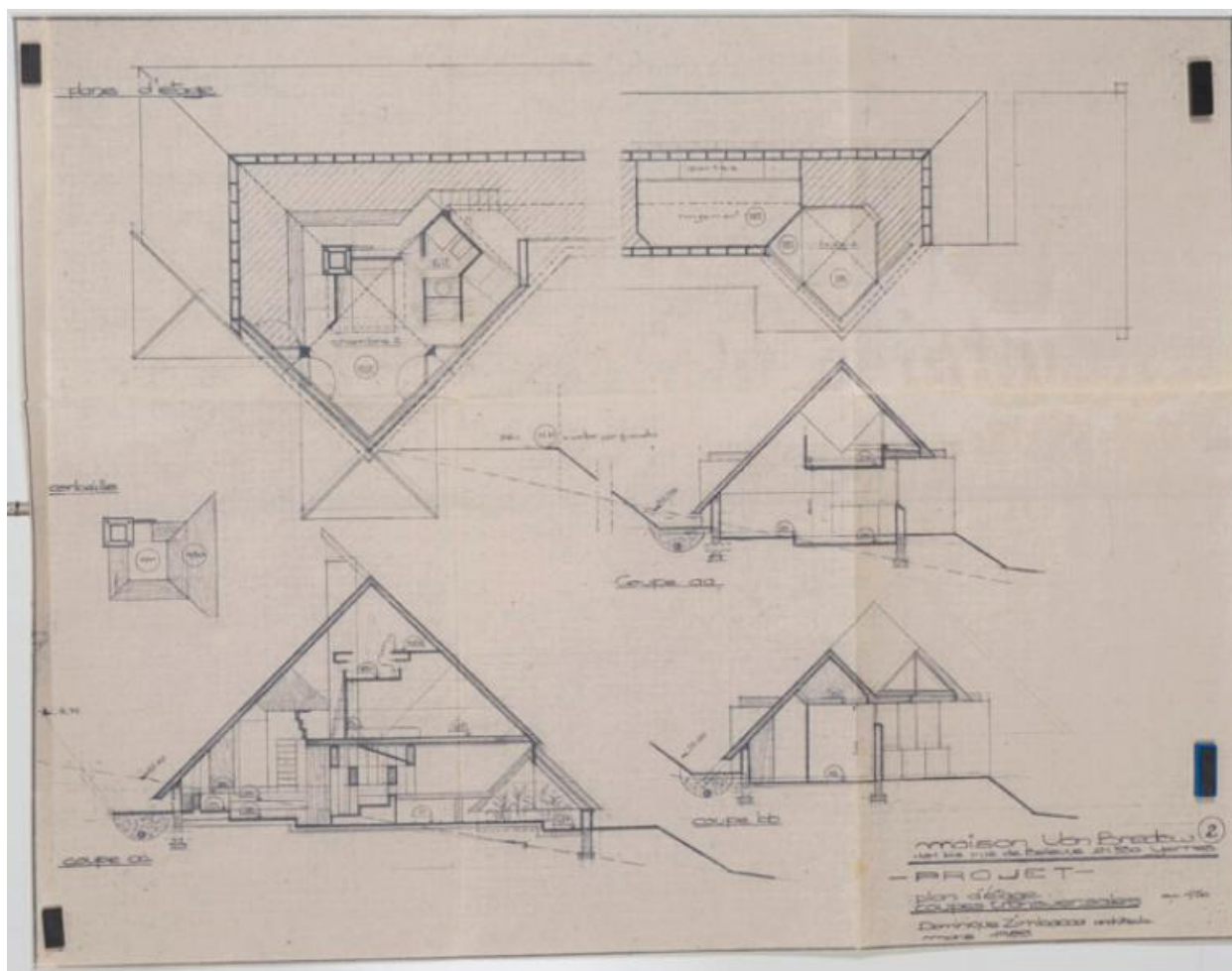
Plan d'étages-coupes transversales.
