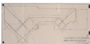
Plan de couverture. Autr. Jean-Pierre, Raymond Zimbacca IVR11_20179100129NUC4A
