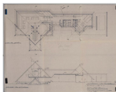
Plan rez de jardin-coupe de principe. Autr. Jean-Pierre, Raymond Zimbacca IVR11_20179100127NUC4A
