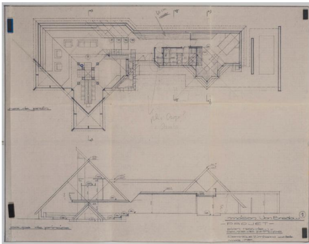
Plan rez de jardin-coupe de principe.
