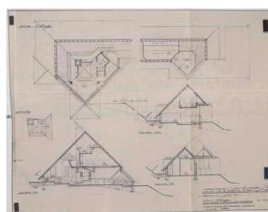
Plan d'étages-coupes transversales. Autr. Jean-Pierre, Raymond Zimbacca IVR11_20179100130NUC4A
