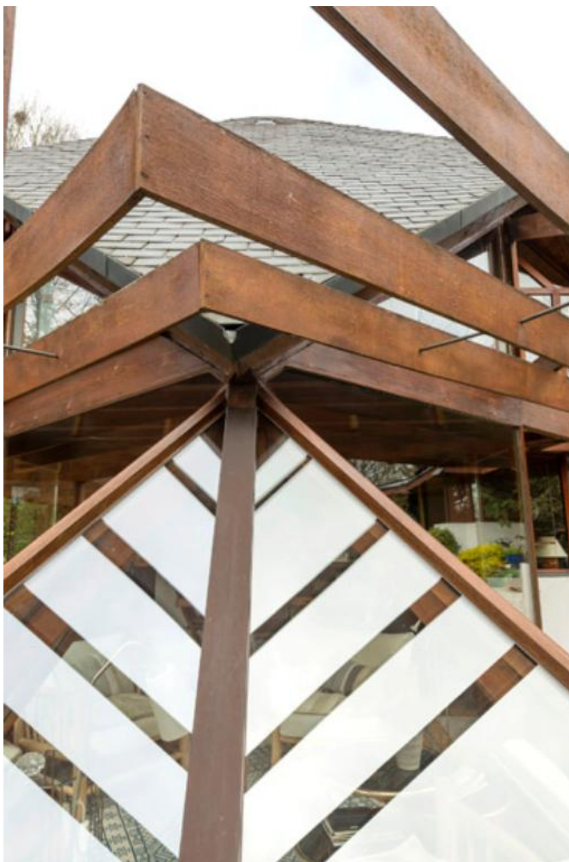
Vue de la façade principale : détail de la jonction toiture et véranda pyramiadales de l'avant-corps Ouest.
