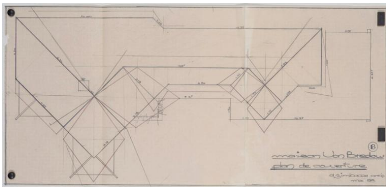
Plan de couverture.
