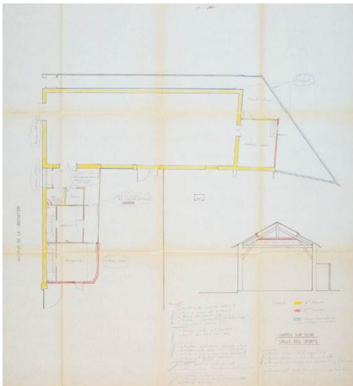
Plan et coupe des bâtiments transformés en gymnase. (AM Samois-sur-Seine, permis de construire, 1986)
