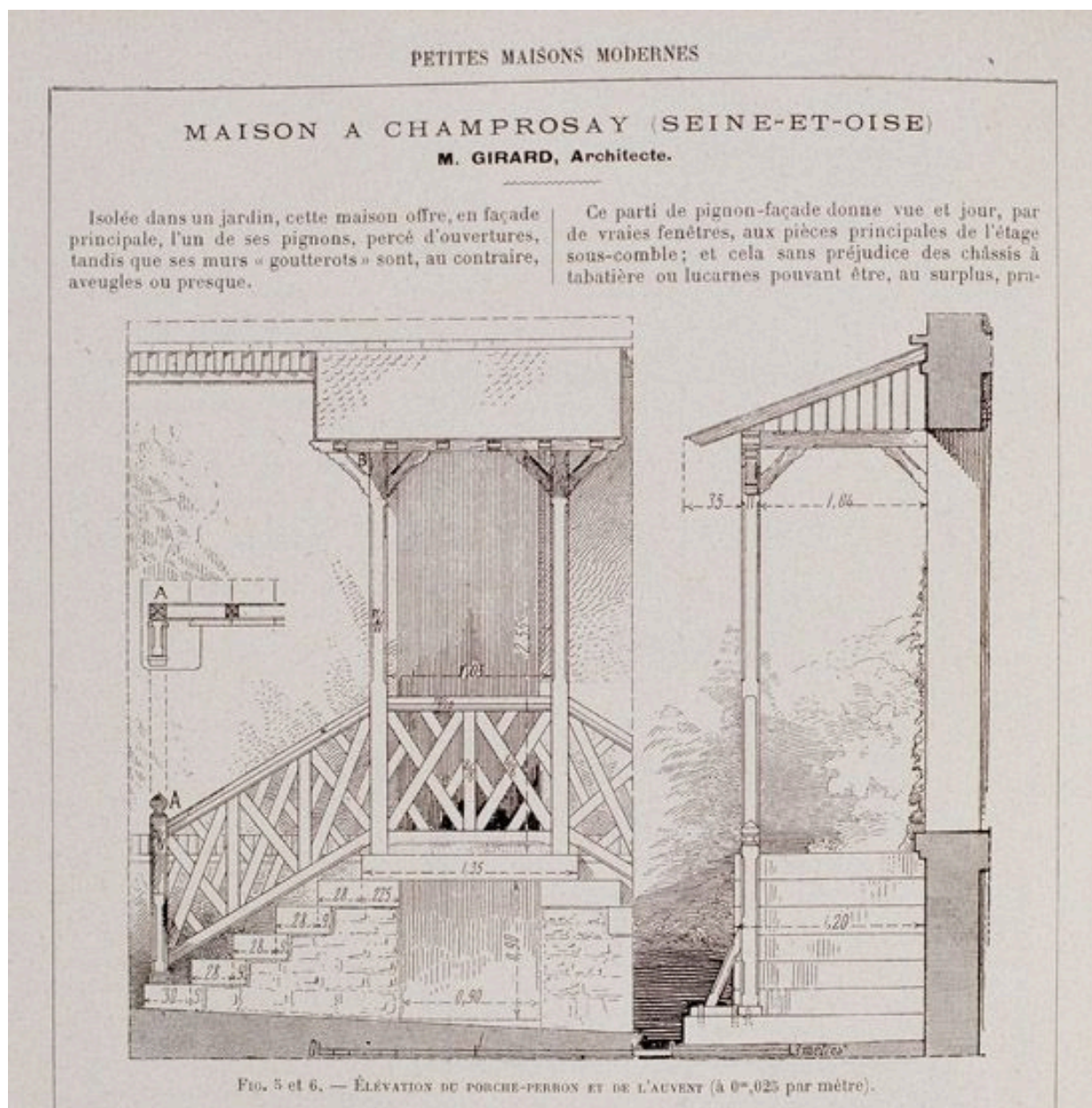
Maison à Champrosay : élévation du porche-perron et de l'auvent ; projet. (BHVP, 114691)
