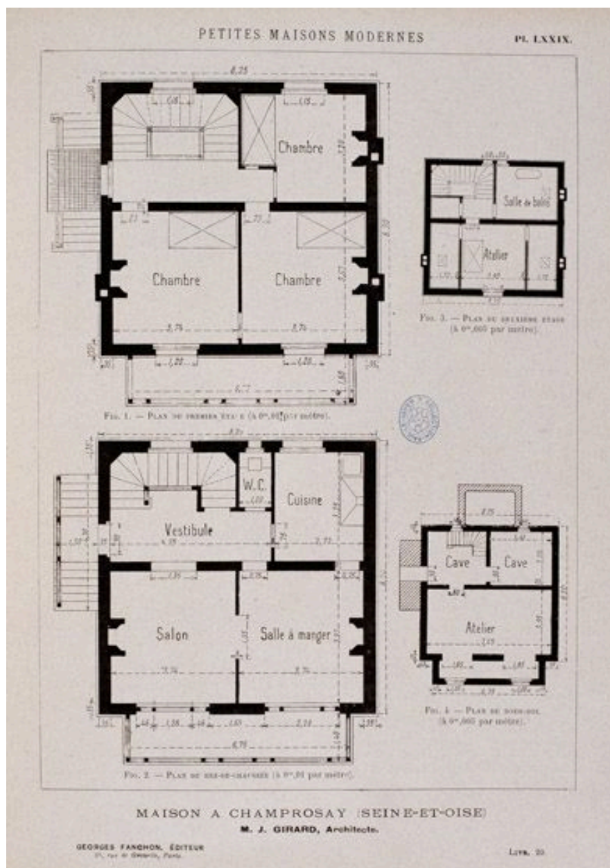
Maison à Champrosay : plans des différents niveaux ; projet. (BHVP, 114691)
