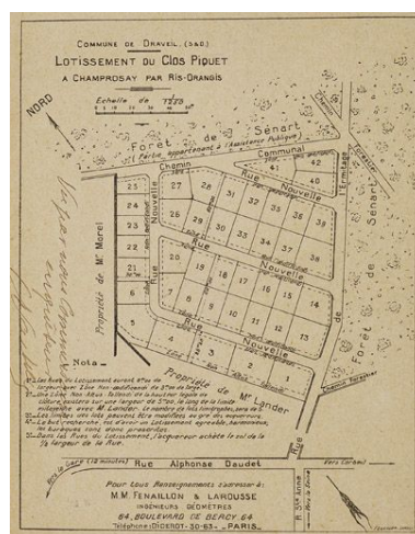
Plan parcellaire du lotissement du Clos Piquet. Ce lotissement,
