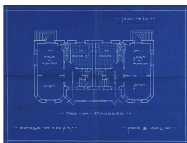
Maison double (à deux logements) du type 115 : plan du rez-de-chaussée. (Société coopérative "Paris-Jardins" de Draveil, dossier 182) Phot. Philippe Ayrault, Autr. Jean (architecte) Walter IVR11_20069100948XA
