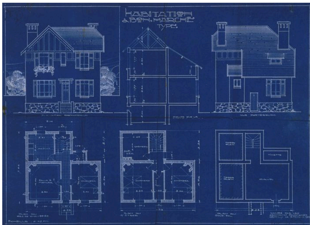
Plan d'un pavillon : élévations, coupe et niveaux. (Société coopérative ""Paris-Jardins"" de Draveil, dossier 101)
