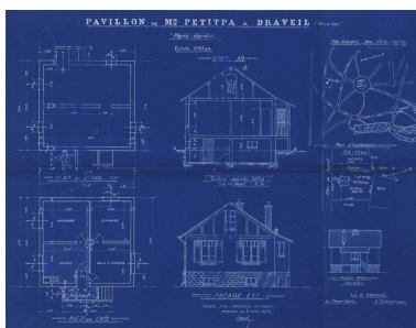
Plan de la maison construite pour M. Petipa, 16 allée des Vergers : élévations, coupe, plans du sous-sol et du rez-de-chaussée, implantation. Cette maison a été agrandie. (Société coopérative ""Paris-Jardins"" de Draveil, dossier 69) Phot. Philippe Ayrault, Autr. Louis (architecte) Martin IVR11_20069100930XA
