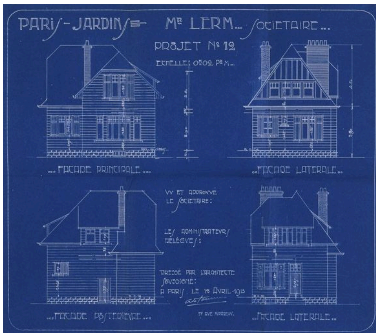
Plan de la maison de M. Lerm, 31 allée des Vergers : élévations. (Société coopérative ""Paris-Jardins"" de Draveil, dossier 16)
