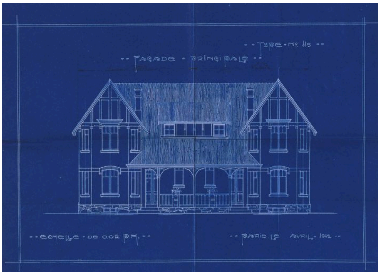
Maison double (à deux logements) du type 115 : plan de la façade principale. (Société coopérative "Paris-Jardins" de Draveil, dossier 182)
