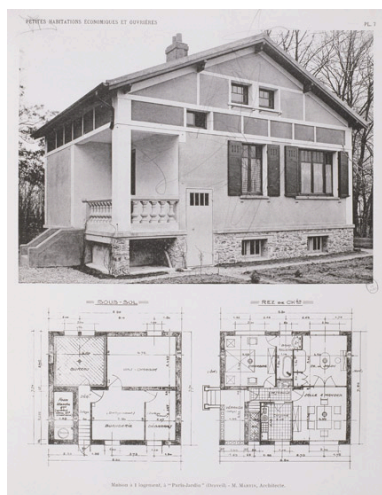
Plans des niveaux et vue d'ensemble du pavillon, allée de la Cité nouvelle. Aujourd'hui, la façade a été légèrement modifiée par un agrandissement latéral. Photographie et plans, s.d. Tiré de : Petites habitations économiques et ouvrières./ Hector Saint-Sauveur. Paris : Ch. Massin et Cie, [192?]. (BHVP, 94066) Phot. Philippe Ayrault IVR11_20069100195XAB
