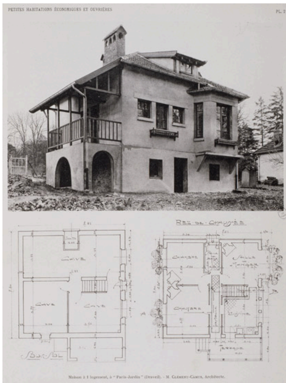
Pavillon : plans du rez-de-chaussée, du sous-sol et photographie de la façade. Tiré de : Petites habitations économiques et ouvrières./ Hector Saint-Sauveur. Paris : Ch. Massin et Cie, [192?]. (BHVP, 94066)
