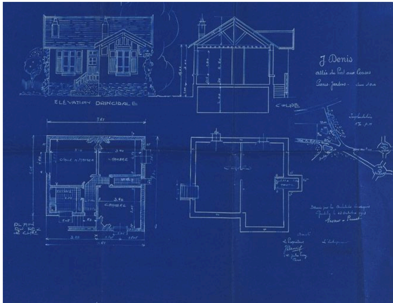
Plan de la maison construite pour le sociétaire J. Denis : élévation principale, coupe, niveaux et implantation. (Société coopérative ""Paris-Jardins"" de Draveil, dossier 101)
