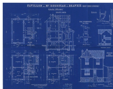
Plans de la maison de M. Rousseau, 8 allée de la Perspective : implantation, élévations, coupe et plans par niveaux. (Société coopérative ""Paris-Jardins"" de Draveil, dossier 237) Phot. Philippe Ayrault, Autr. Louis (architecte) Martin IVR11_20069100951XA
