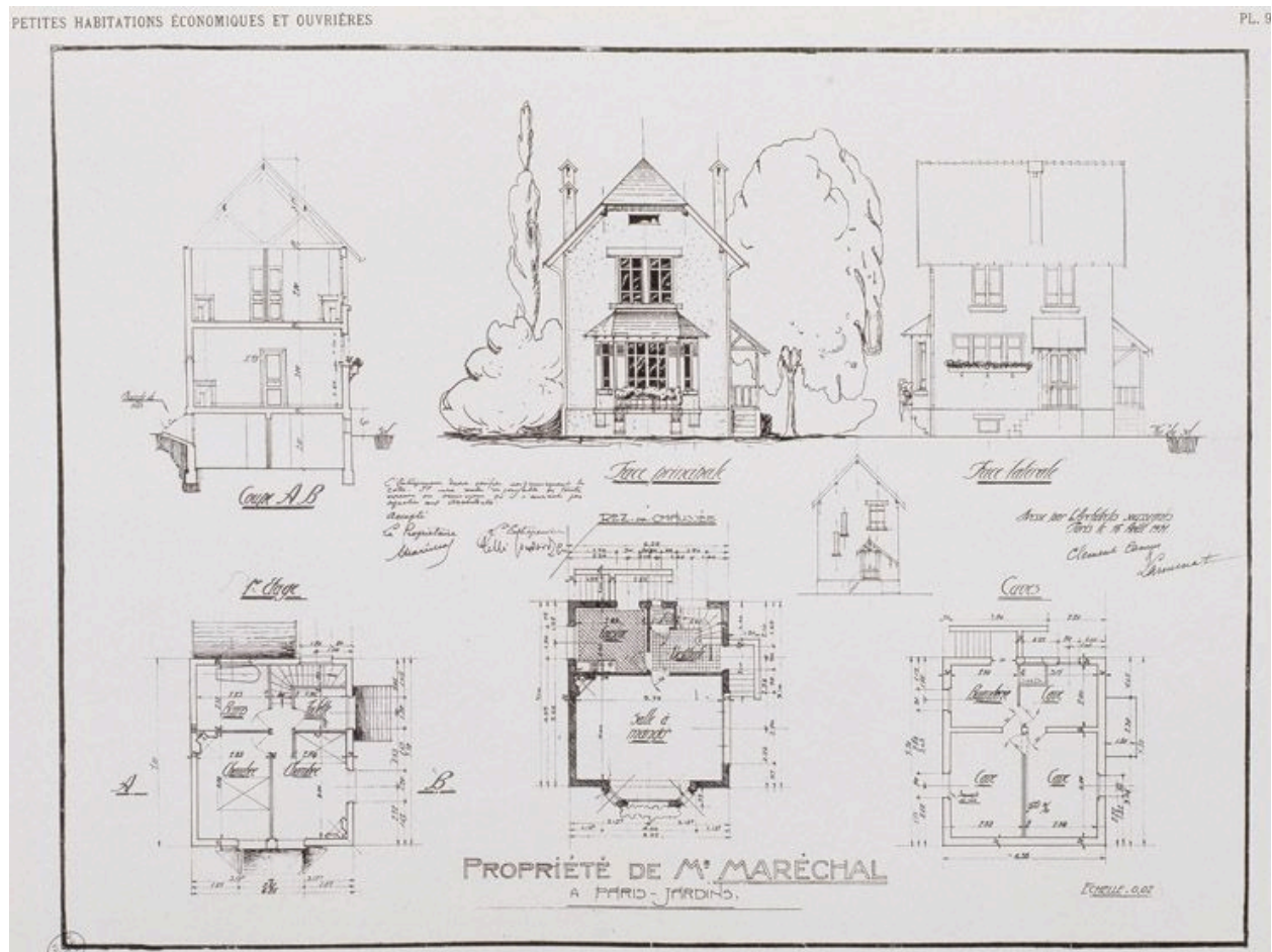
Elévations, coupe et plans d'un pavillon. Plans, 16 avril 1921. Tiré de : Petites habitations économiques et ouvrières./ Hector Saint-Sauveur. Paris : Ch. Massin et Cie, [192?]. (BHVP, 94066)
