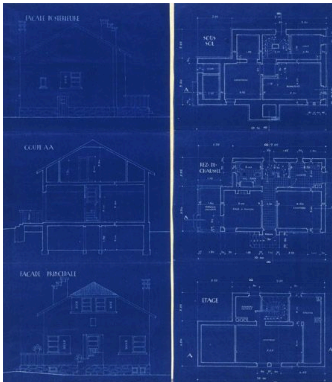
Plan d'une maison projetée : élévations, coupe, niveaux. (Société coopérative ""Paris-Jardins"" de Draveil)
