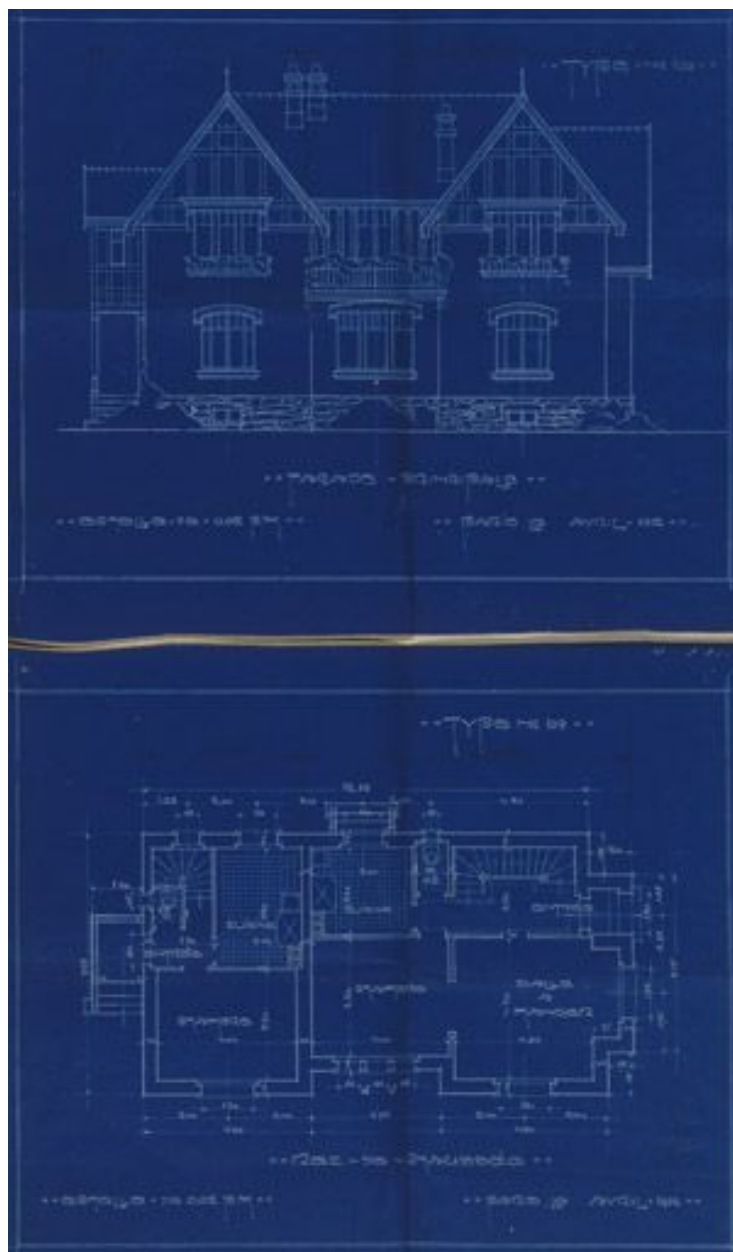
Plan de la maison double du type 109 : élévation principale et plan de distribution. (Société coopérative ""Paris-Jardins"" de Draveil, dossier 176)
