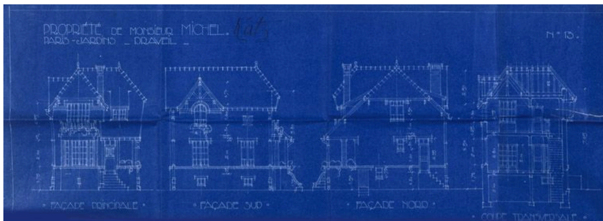
Plan de la maison de M. Michel : élévations et coupe transversale ; s. d. (Société coopérative ""Paris-Jardins"" de Draveil, dossier 281)
