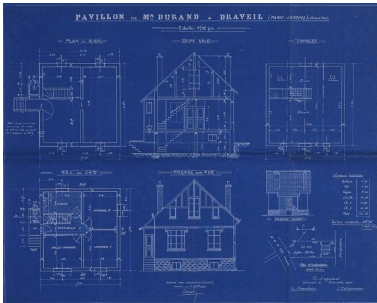
Plans de la maison de M. Durand : implantation, élévations, coupe et plans par niveaux. (Société coopérative ""Paris-Jardins"" de Draveil, dossier 229)
