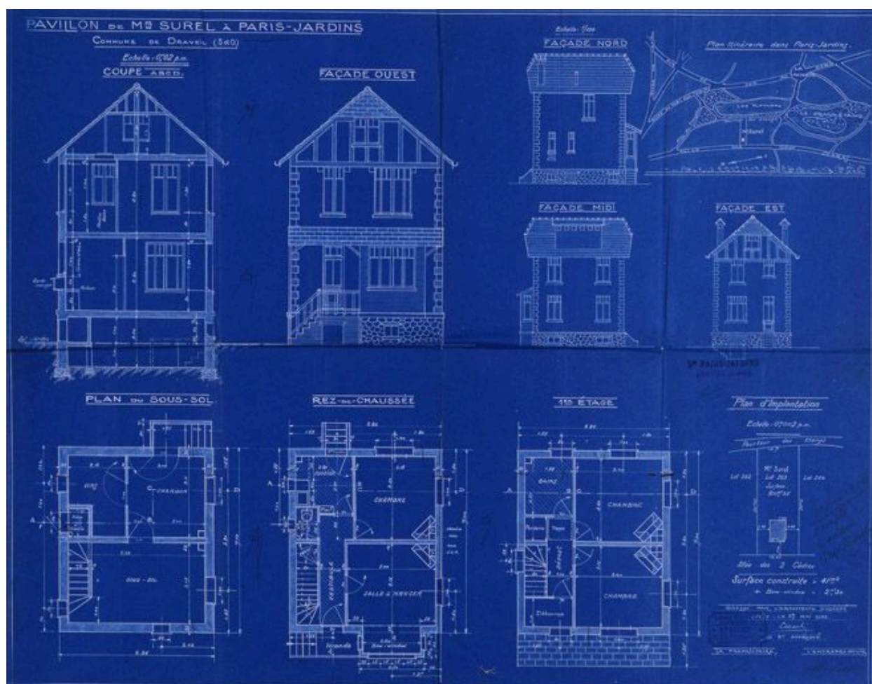
Plans de la maison de M. Surel, 28 allée des Deux-Cèdres : implantation, élévations, coupe et plans par niveaux. Elle a été construite (avec quelques variantes). (Société coopérative "Paris-Jardins" de Draveil, dossier 263)
