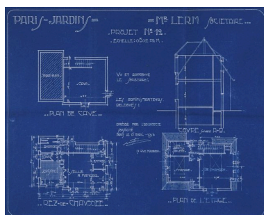
Plans de la maison de M. Lerm : cave, rez-de-chaussée, étage et coupe. (Société coopérative ""Paris-Jardins"" de Draveil, dossier 16) Phot. Philippe Ayrault, Autr. Maurice (architecte) Fournier IVR11_20069100933XA
