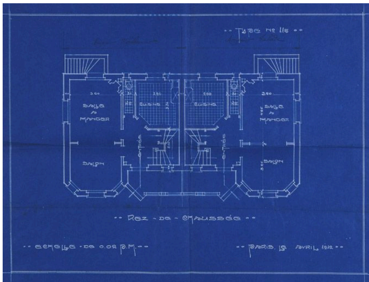
Maison double (à deux logements) du type 115 : plan du rez-de-chaussée. (Société coopérative "Paris-Jardins" de Draveil, dossier 182)
