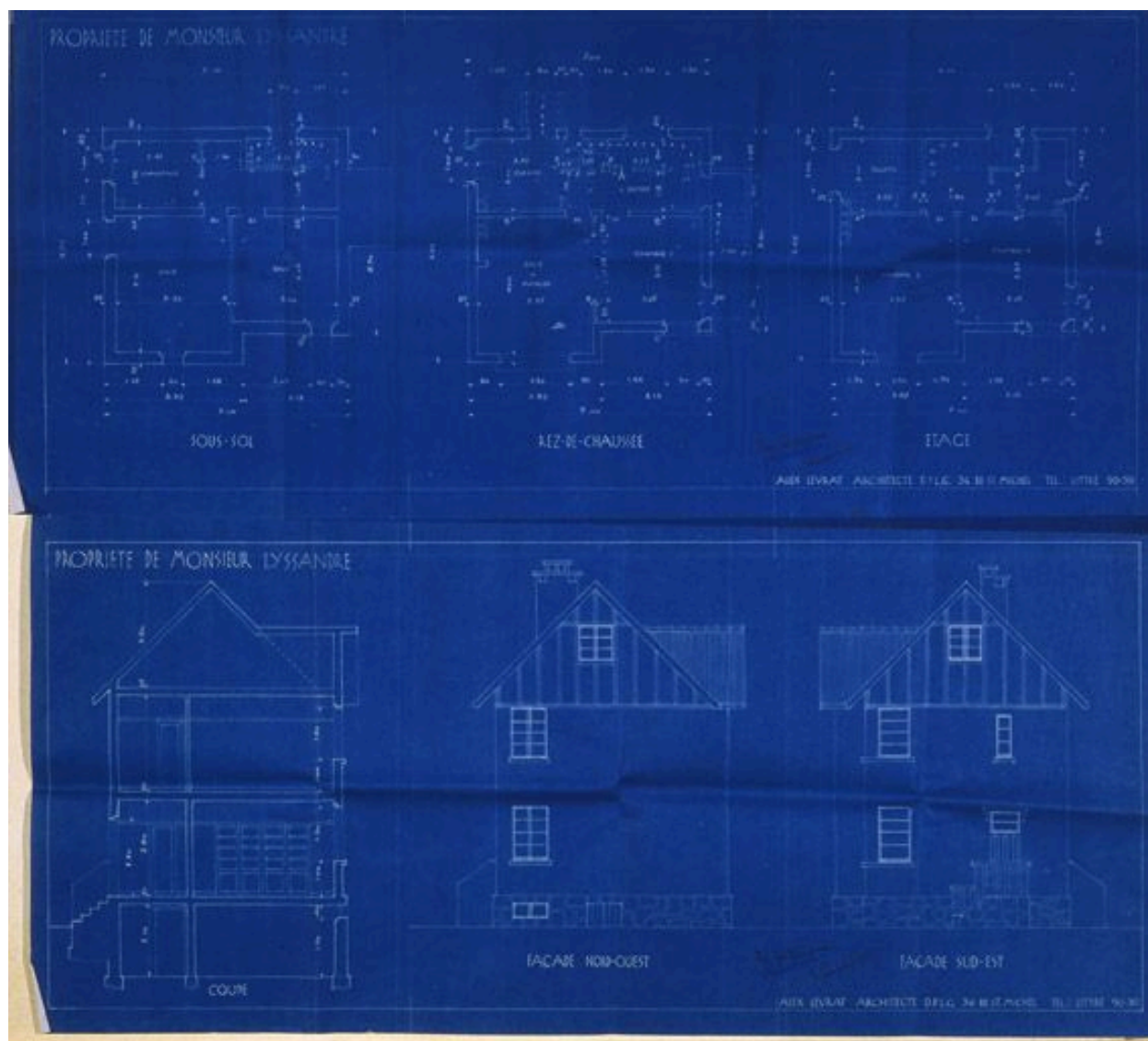
Plan du pavillon construit pour M. Lyssandre : élévations, coupe, plans par niveaux. (Société coopérative ""Paris-Jardins"" de Draveil, dossier 42)
