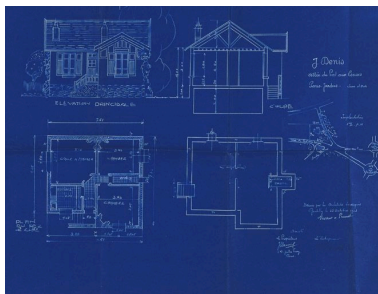
Plan de la maison construite pour le sociétaire J. Denis : élévation principale, coupe, niveaux et implantation. (Société coopérative ""Paris-Jardins"" de Draveil, dossier 101) Phot. Philippe Ayrault, Autr. Pierre (architecte) Prunet, Autr. Roger (architecte) Vasseur IVR11_20069100938XA
