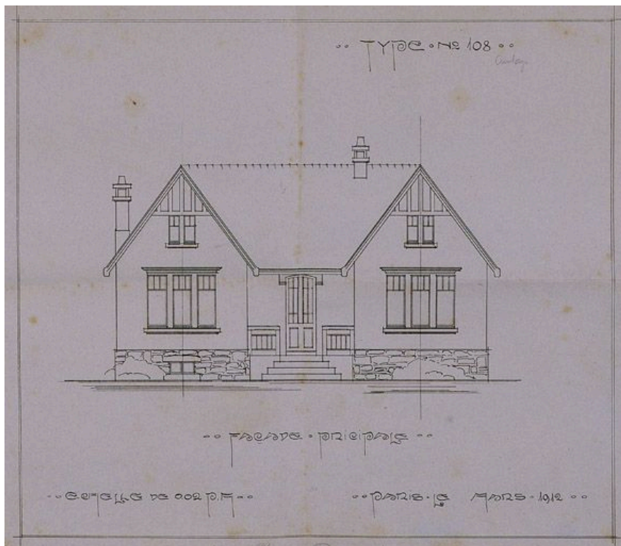
Plan d'une maison du type n° 108 : élévation principale. (Société coopérative ""Paris-Jardins"" de Draveil)
