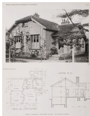
Plan du rez-de-chaussée, coupe et vue d'ensemble du pavillon. Photographie et plans, s.d. Tiré de : Petites habitations économiques et ouvrières./ Hector Saint-
