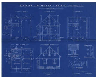
Plans de la maison de M. Durand : implantation, élévations, coupe et plans par niveaux. (Société coopérative ""Paris-Jardins"" de Draveil, dossier 229) Phot. Philippe Ayrault, Autr. Louis (architecte) Martin IVR11_20069100952XA
