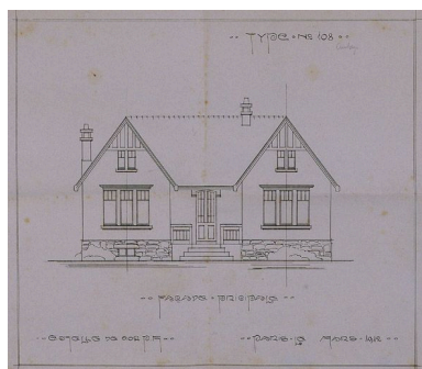
Plan d'une maison du type n° 108 : élévation principale. (Société coopérative "Paris-Jardins" de Draveil) Phot. Philippe Ayrault, Autr. Jean (architecte) Walter IVR11_20069100942XA
