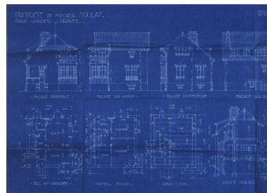
Plan de la maison de M. Soulat, 38 Parc-aux-Daims. Elle a été construite sur les plans de l'architecte Robert Gilles par l'entreprise René Picard (69, rue de Clichy à Paris) : élévations, coupe, plans du sous- sol, du rez-de-chaussée et de l'étage. (Société coopérative ""Paris- Jardins"" de Draveil, dossier 144) Phot. Philippe Ayrault IVR11_20069100931XA
