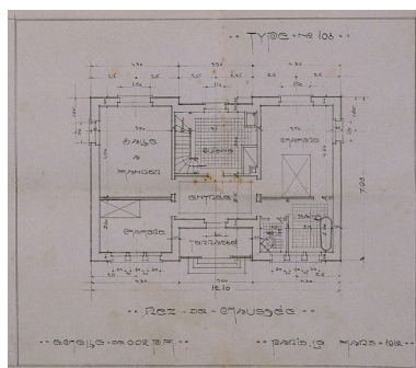
Maison du type n° 108 : plan du rez-de-chaussée. (Société coopérative "Paris-Jardins" de Draveil) Phot. Philippe Ayrault, Autr. Jean (architecte) Walter IVR11_20069100943XA
