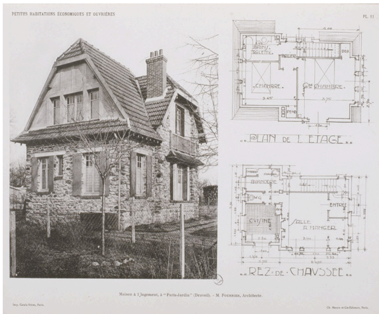
Maison, 31 allée des Vergers. Plans des niveaux et photographie du pavillon. Tiré de : Petites habitations économiques et ouvrières./ Hector Saint-Sauveur. Paris : Ch. Massin et Cie, [192?]. (BHVP, 94066)
