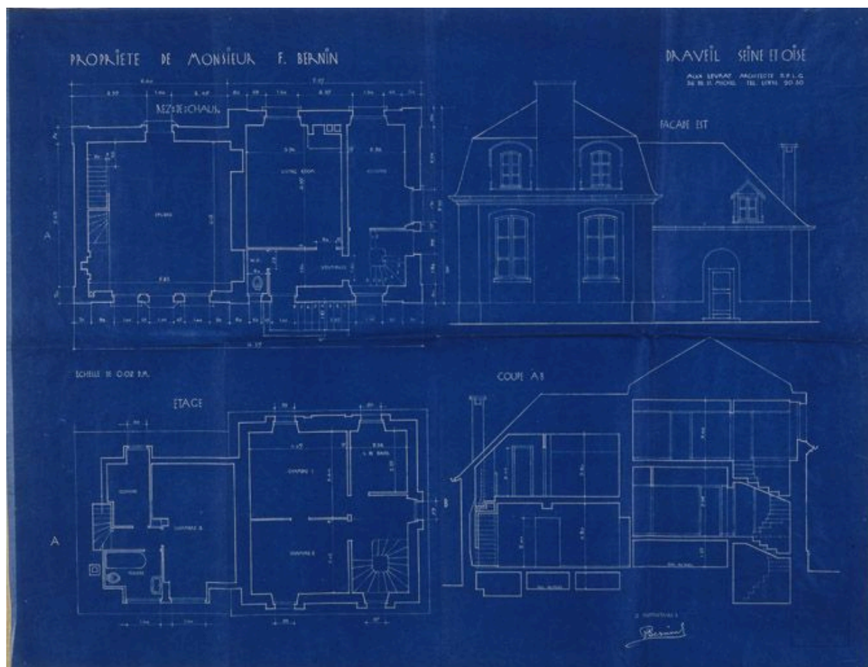
Cour d'honneur : plan du pavillon construit pour M. Bernin : élévations, coupe, plans par niveaux. (Société coopérative ""Paris-Jardins"" de Draveil, dossier 311)
