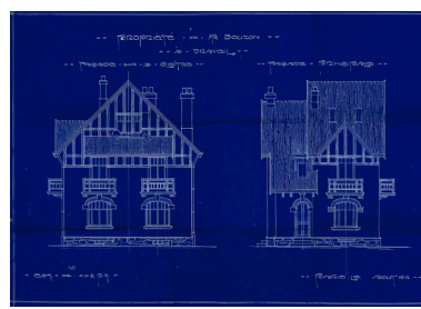
Plan de la maison de M. Bouzon, 1 allée de la Petite-Ferme : façade principale et façade sur le "cloître". (Société coopérative "Paris-Jardins" de Draveil, dossier 92) Phot. Philippe Ayrault, Autr. Jean (architecte) Walter IVR11_20069100945XA
