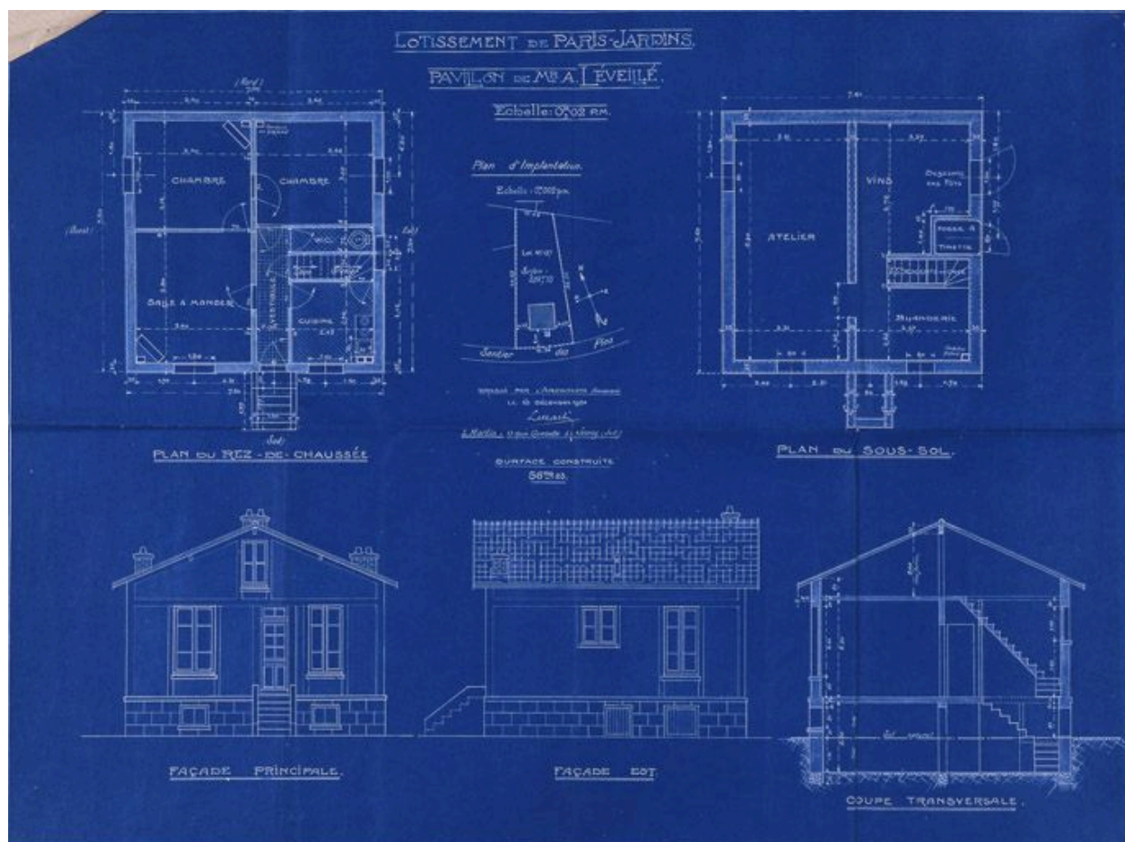
Plans de la maison de M. Léveillé : implantation, élévations, coupe et plans par niveaux. (Société coopérative ""Paris-Jardins"" de Draveil, dossier 137)
