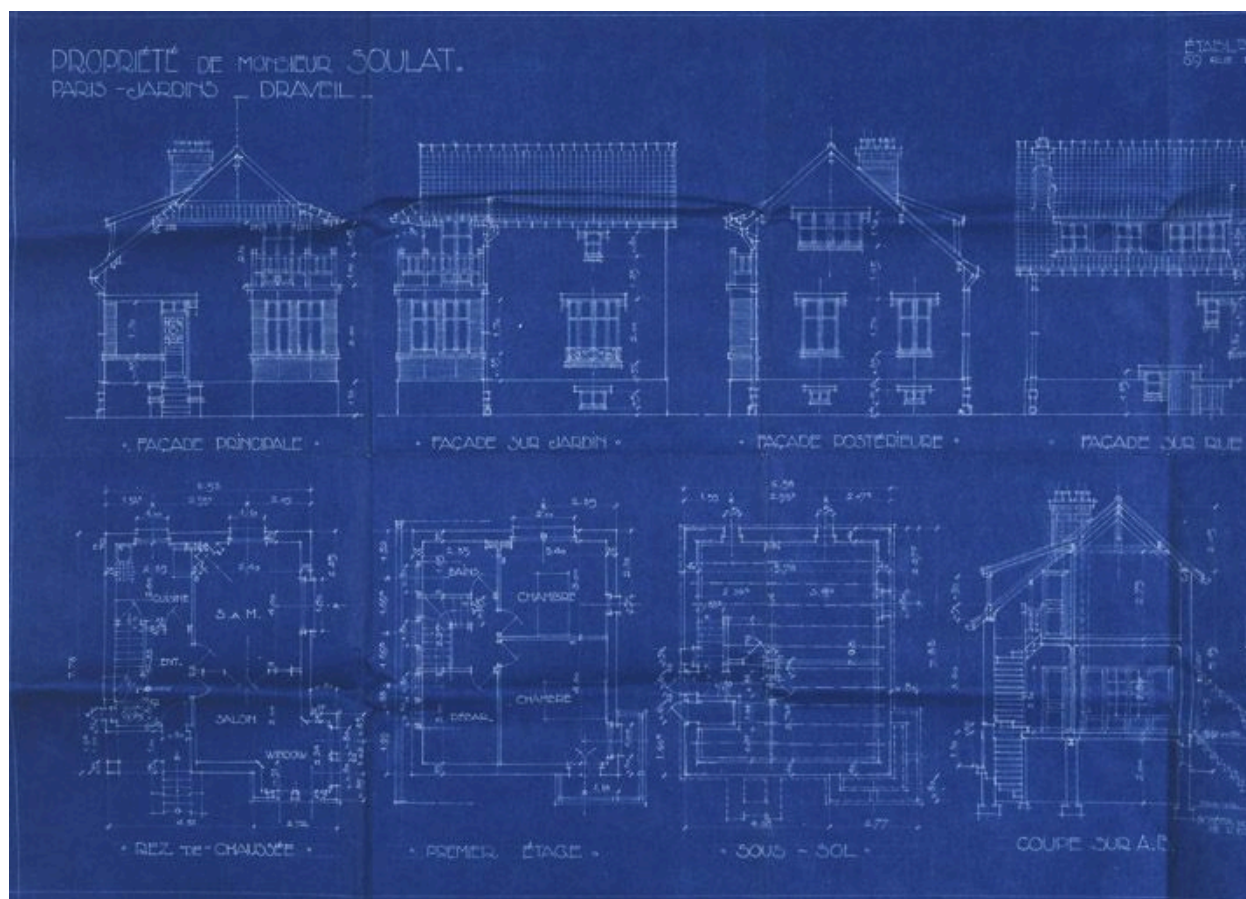
Plan de la maison de M. Soulat, 38 Parc-aux-Daims. Elle a été construite sur les plans de l'architecte Robert Gilles par l'entreprise René Picard (69, rue de Clichy à Paris) : élévations, coupe, plans du sous-sol, du rez-de-chaussée et de l'étage. (Société coopérative "Paris-Jardins" de Draveil, dossier 144)
