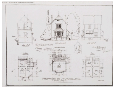
Elévations, coupe et plans d'un pavillon. Plans, 16 avril 1921.
