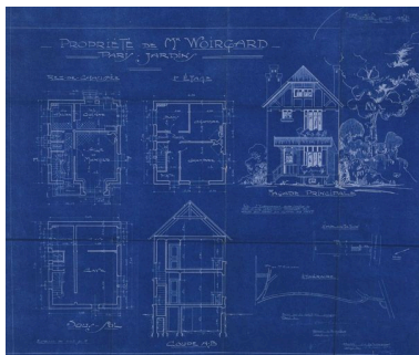
Plan de la maison de M. Woïrgard, 13 allée des Vergers : élévations, coupe, niveaux et implantation. Dans ce type de pavillon à un étage, les pièces sont organisées autour d'un espace ""servant"" (un quart du rectangle) regroupant vestibule, escalier et wc. La façade principale est une façade- pignon et l'entrée, indifféremment sur façade-pignon ou gouttereau, est toujours perpendiculaire au vestibule et placée sous un petit porche. (Société coopérative ""Paris- Jardins"" de Draveil, dossier 7) Phot. Philippe Ayrault, Autr. L. (architecte) Clément-Camus, Autr. Larminat (architecte), Autr. Bultet (entrepreneur) IVR11_20069100940XA
