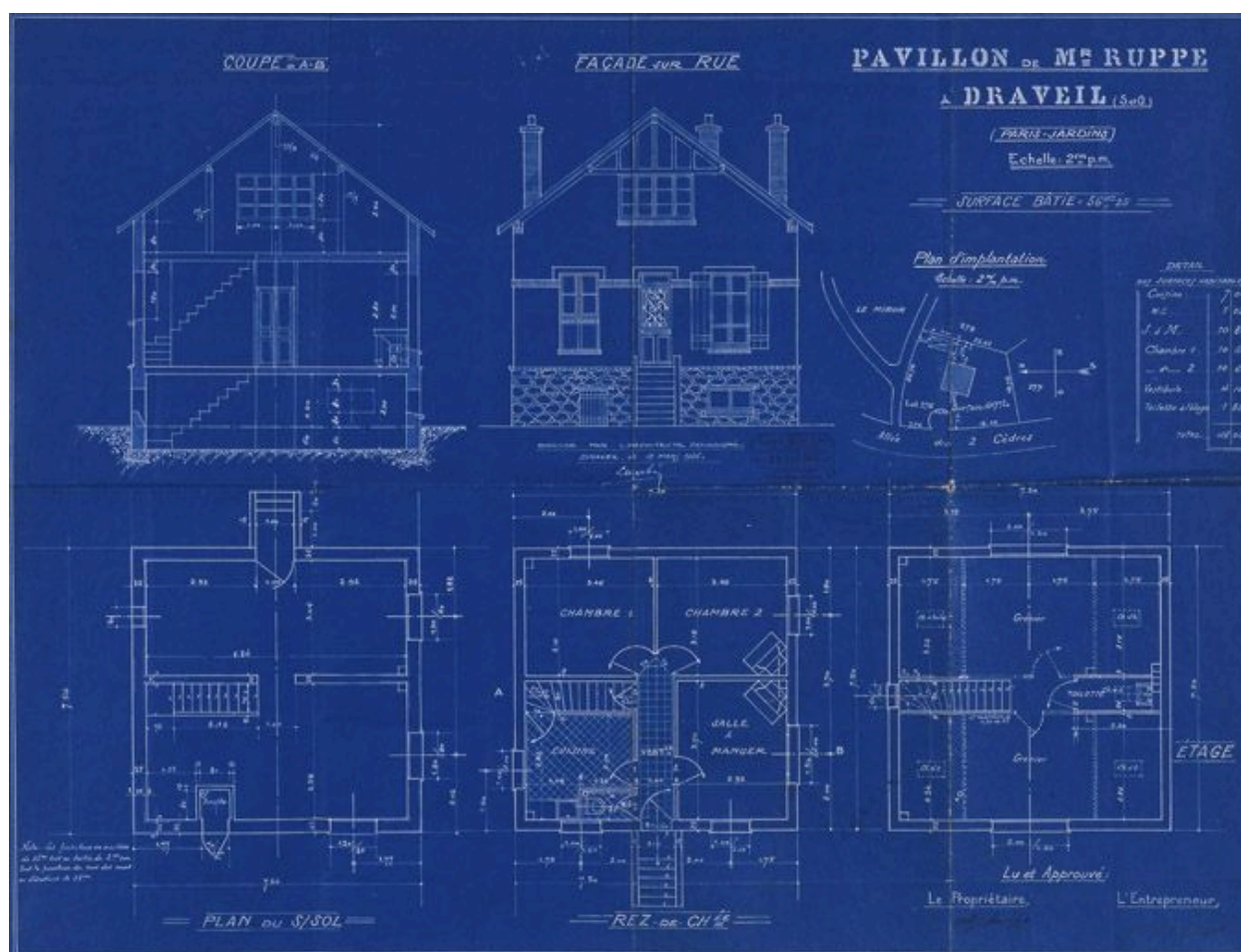
Plans de la maison de M. Ruppe : implantation, élévation principale, coupe et plans par niveaux. (Société coopérative ""Paris-Jardins"" de Draveil, dossier 276)
