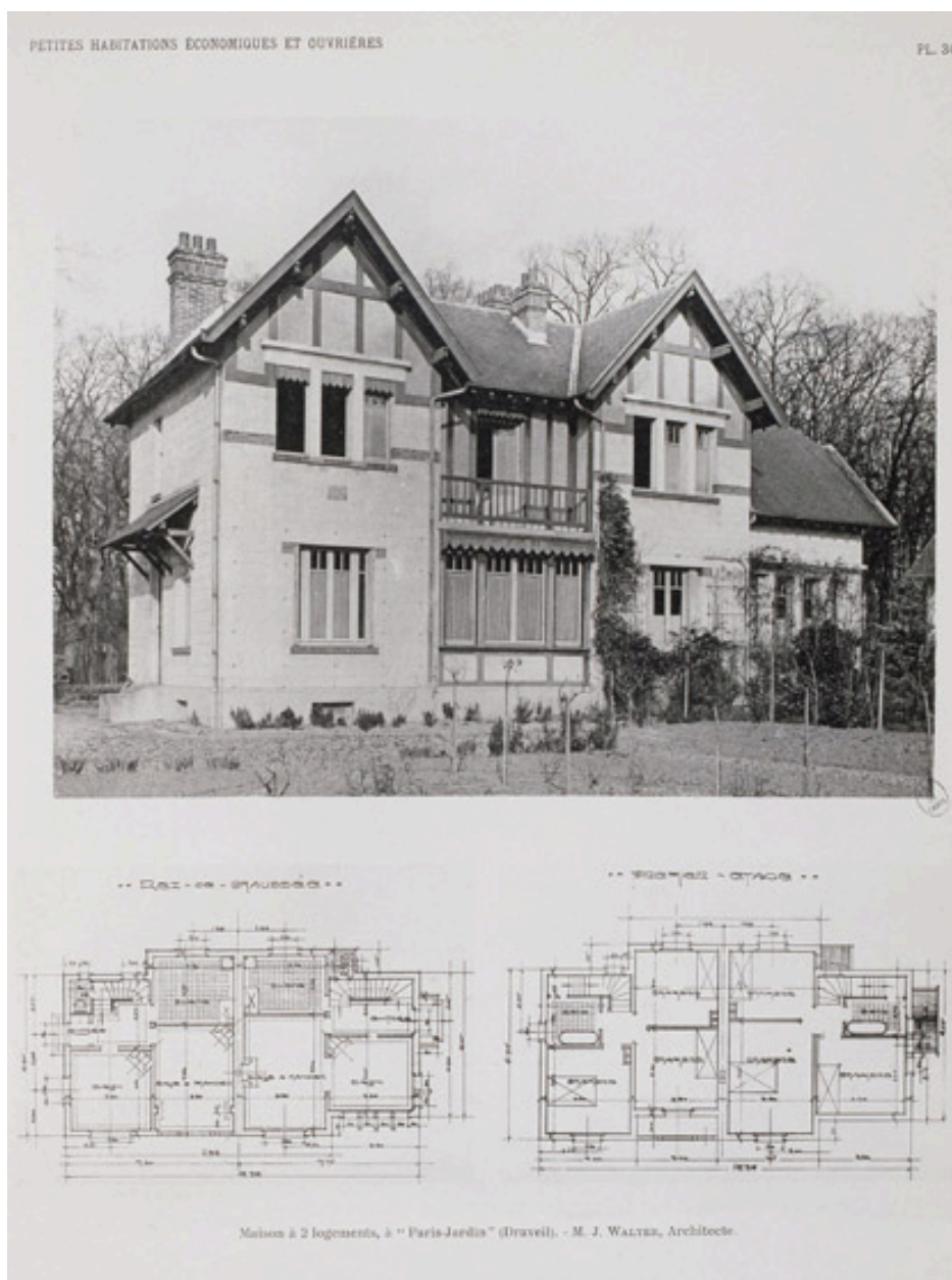
Maison, 19-21 allée de la Perspective. Plans des niveaux et vue d'ensemble du pavillon double. Photographie et plan, s.d. Tiré de : Petites habitations économiques et ouvrières./ Hector Saint-Sauveur. Paris : Ch. Massin et Cie, [192?]. (BHVP, 94066)
