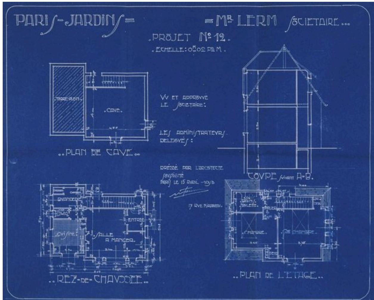
Plans de la maison de M. Lerm : cave, rez-de-chaussée, étage et coupe. (Société coopérative ""Paris-Jardins"" de Draveil, dossier 16)
