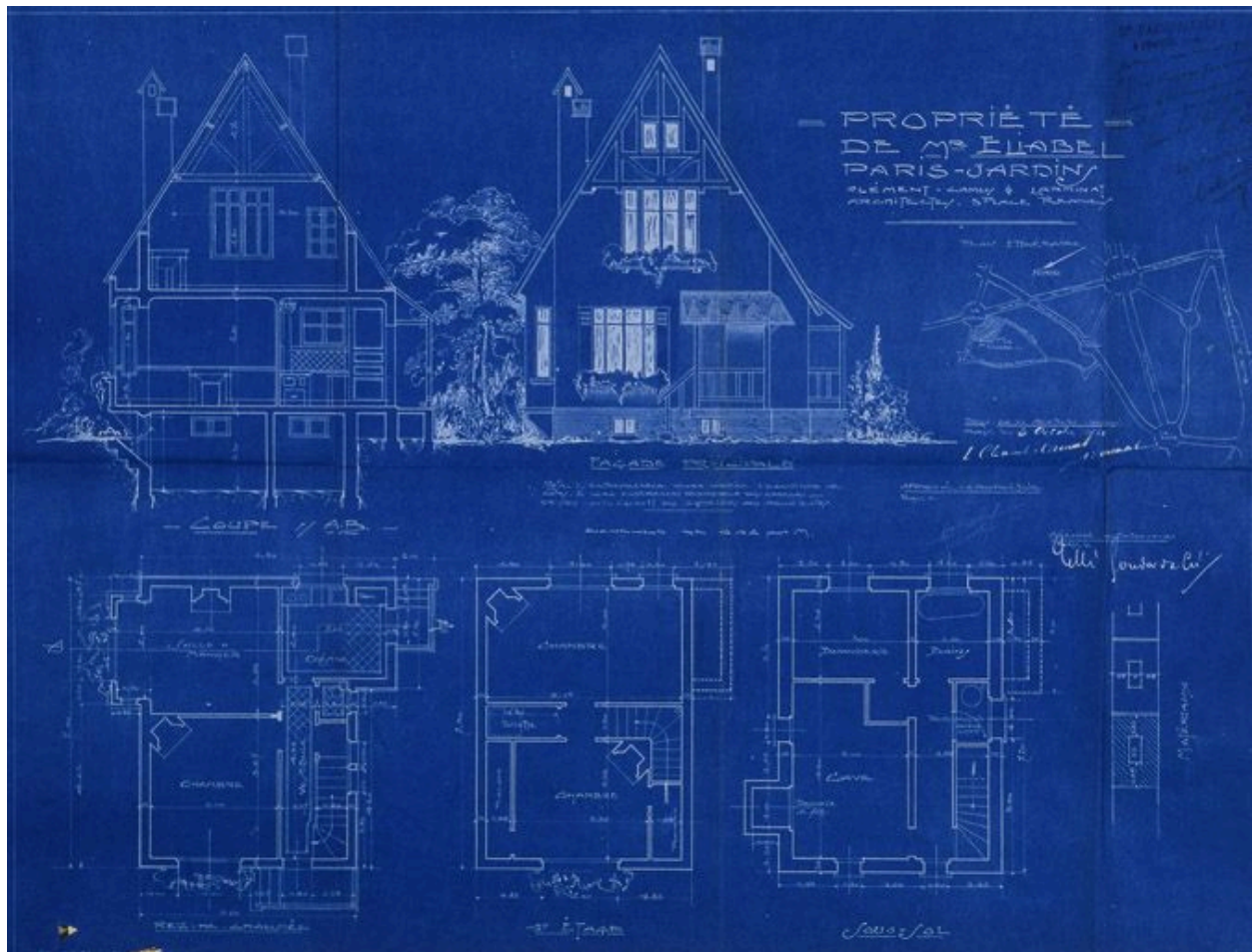
Plans d'une maison construite pour M. Eliabel : implantation, élévation principale, coupe et plans par niveaux. (Société coopérative ""Paris-Jardins"" de Draveil, dossier 172)
