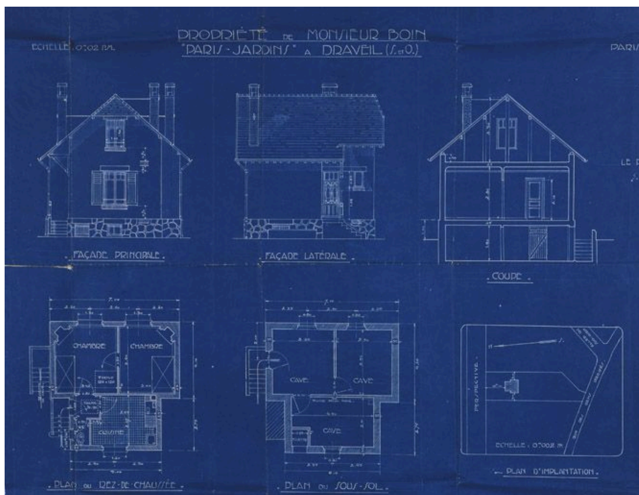
Plan du pavillon de M. Boin, 12 allée de la Perspective : élévations, coupe, plans par niveaux, implantation. Ce pavillon a subi d'importantes transformations. (Société coopérative ""Paris-Jardins"" de Draveil, dossier 239)
