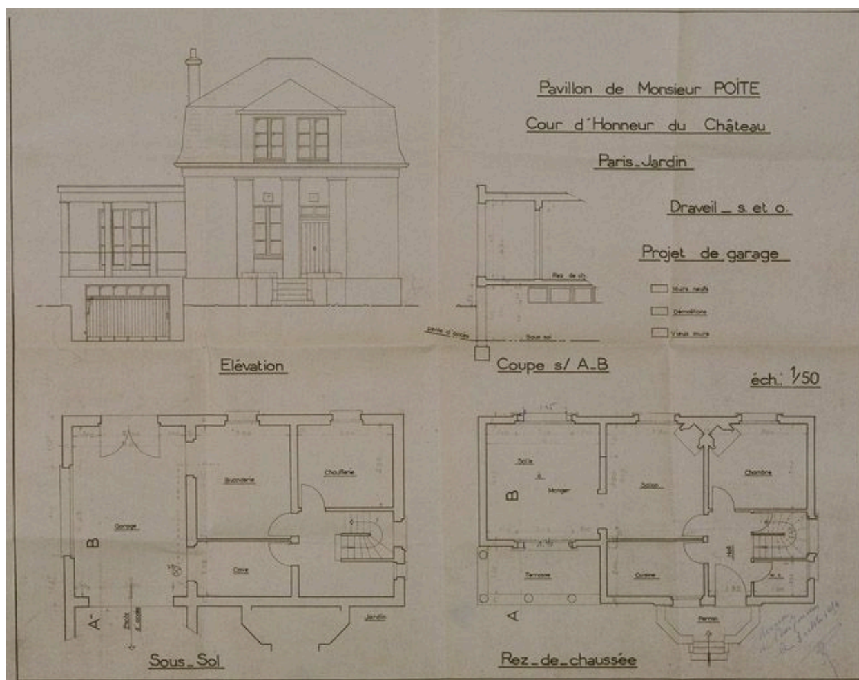
Plans du pavillon construit pour M. Poite, en bordure de la cour d'honneur : élévation principale, sous-sol et rez-de-chaussée, projet de garage. (Société coopérative ""Paris-Jardins"" de Draveil, dossier 314)
