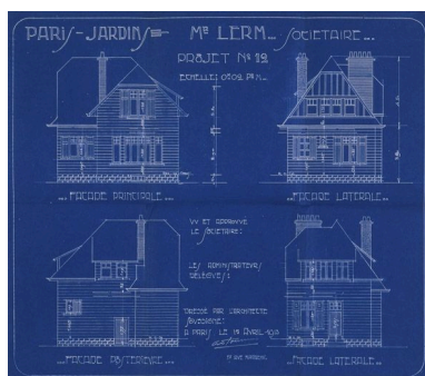
Plan de la maison de M. Lerm, 31 allée des Vergers : élévations. (Société coopérative ""Paris-Jardins"" de Draveil, dossier 16) Phot. Philippe Ayrault, Autr. Maurice (architecte) Fournier IVR11_20069100934XA
