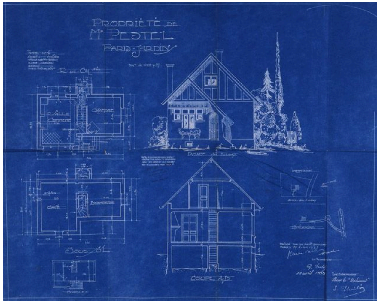
Plans de la maison de M. Pestel (type n° 1) : implantation, élévation, coupe et plans par niveaux. (Société coopérative ""Paris-Jardins"" de Draveil, dossier 271)
