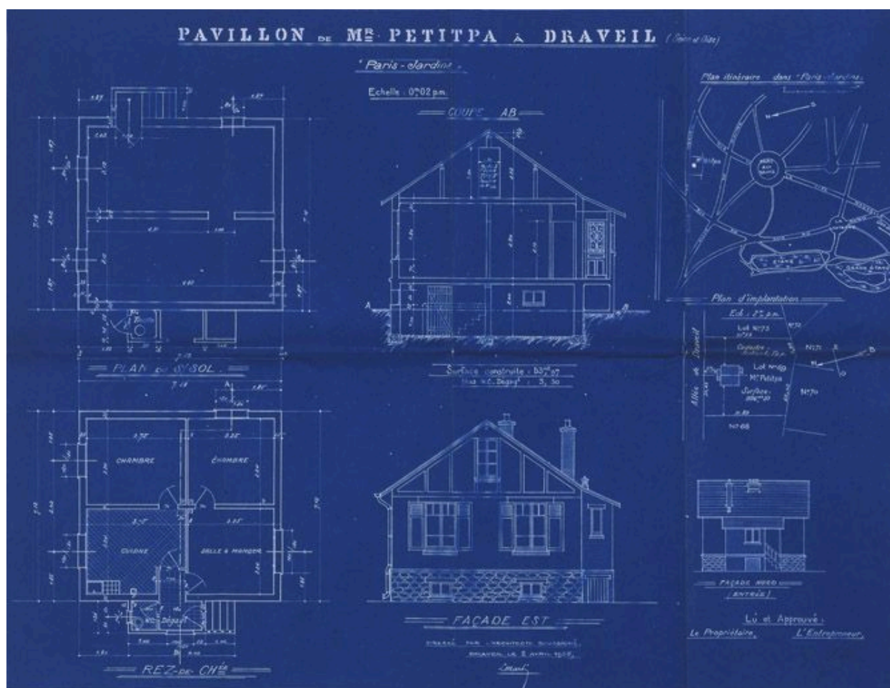
Plan de la maison construite pour M. Petipa, 16 allée des Vergers : élévations, coupe, plans du sous-sol et du rez-de-chaussée, implantation. Cette maison a été agrandie. (Société coopérative "Paris-Jardins" de Draveil, dossier 69)
