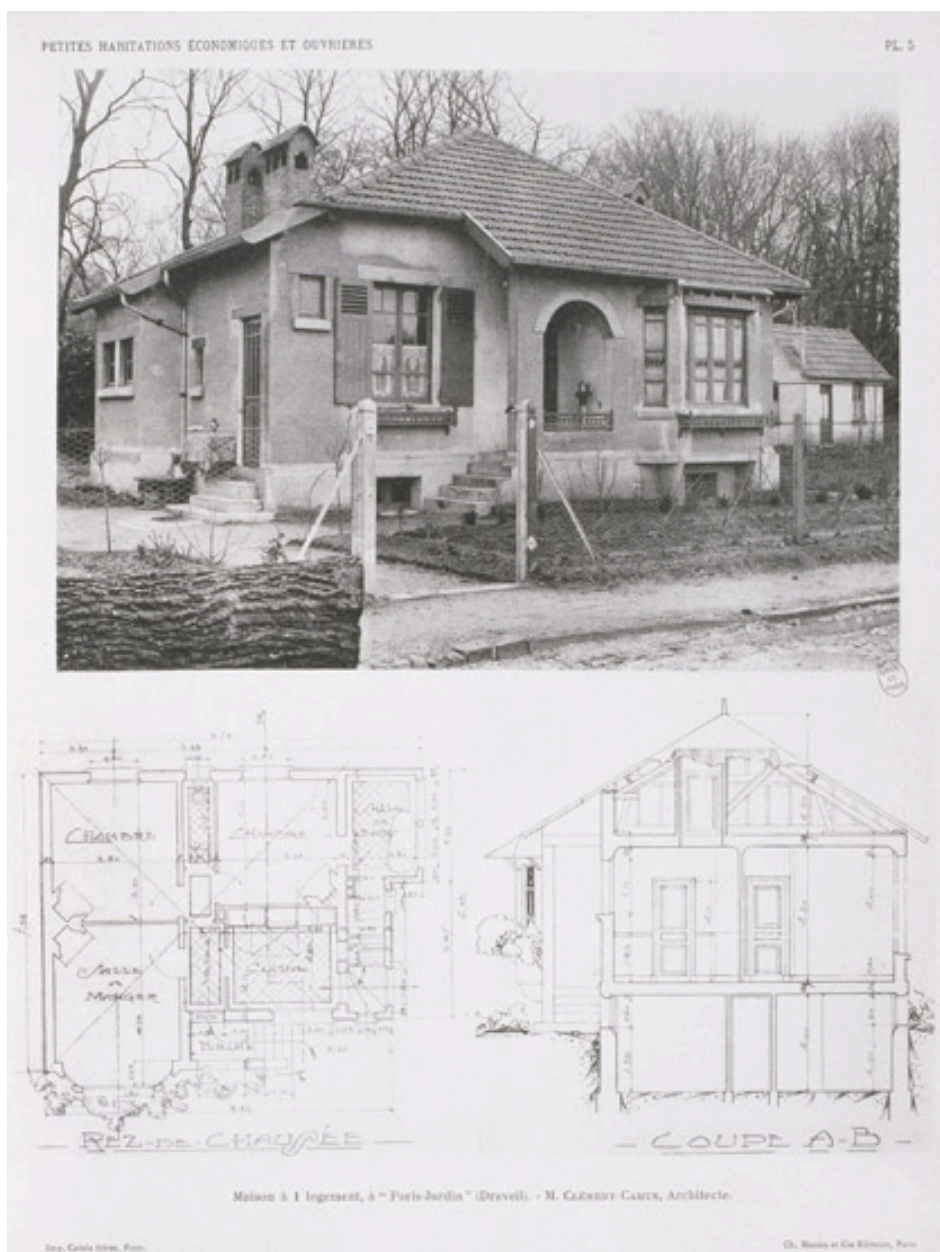
Plans des niveaux et vue d'ensemble d'un pavillon en rez-de-chaussée. Photographie et plans, s.d. Tiré de : Petites habitations économiques et ouvrières./ Hector Saint-Sauveur. Paris : Ch. Massin et Cie, [192?]. (BHVP, 94066)
