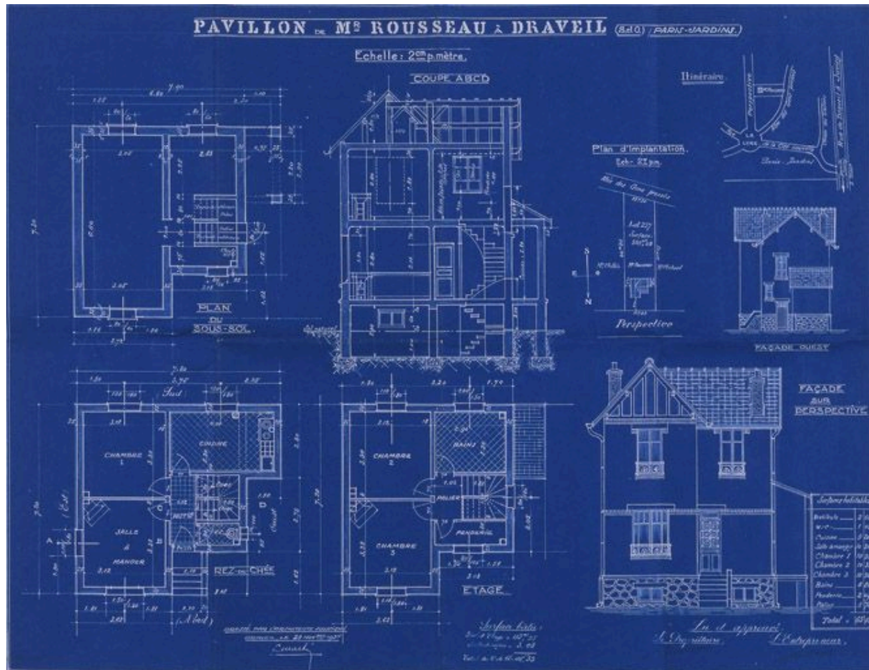
Plans de la maison de M. Rousseau, 8 allée de la Perspective : implantation, élévations, coupe et plans par niveaux. (Société coopérative "Paris-Jardins" de Draveil, dossier 237)
