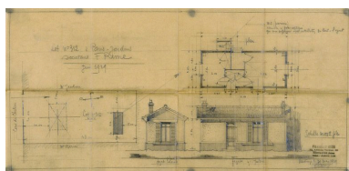
Plan d'une maisonnette en rez-de-chaussée dressé par l'entrepreneur Franklin Rime (Montrouge, 38 avenue Verdier), pour le lot 312 lui appartenant ; calque, 31 mai 1929. Ce type d'édifice, facilement démontable, de 18 m2 maximum (au lieu de 12 précédemment), a été autorisé en 1921. (Société coopérative ""Paris-Jardins"" de Draveil, dossier 312) Phot. Philippe Ayrault IVR11_20069100925XA
