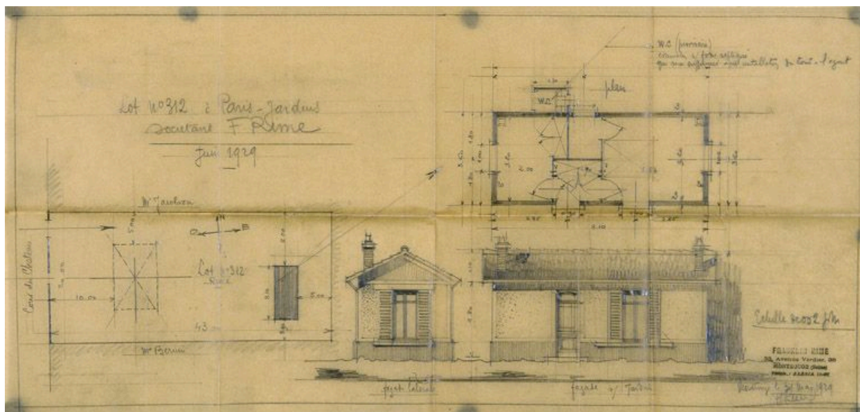
Plan d'une maisonnette en rez-de-chaussée dressé par l'entrepreneur Franklin Rime (Montrouge, 38 avenue Verdier), pour le lot 312 lui appartenant ; calque, 31 mai 1929. Ce type d'édifice, facilement démontable, de 18 m 2 maximum (au lieu de 12 précédemment), a été autorisé en 1921. (Société coopérative ""Paris-Jardins"" de Draveil, dossier 312)
