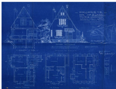
Plans d'une maison construite pour M. Eliabel : implantation, élévation principale, coupe et plans par niveaux. (Société coopérative ""Paris-Jardins"" de Draveil, dossier 172) Phot. Philippe Ayrault, Autr. L. (architecte) Clément-Camus, Autr. R. (architecte) Larminat IVR11_20069100959XA
