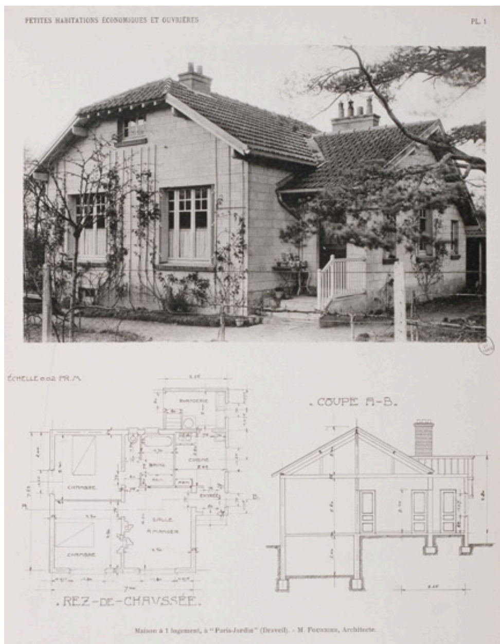
Plan du rez-de-chaussée, coupe et vue d'ensemble du pavillon. Photographie et plans, s.d. Tiré de : Petites habitations économiques et ouvrières./ Hector Saint-Sauveur. Paris : Ch. Massin et Cie, [192?]. (BHVP, 94066)
