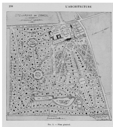
Plan d'ensemble du lotissement. Plan, 5 mars 1910. Tiré de : L'Architecture, 1914, p.237-240. (BHVP, Per F° 599)
