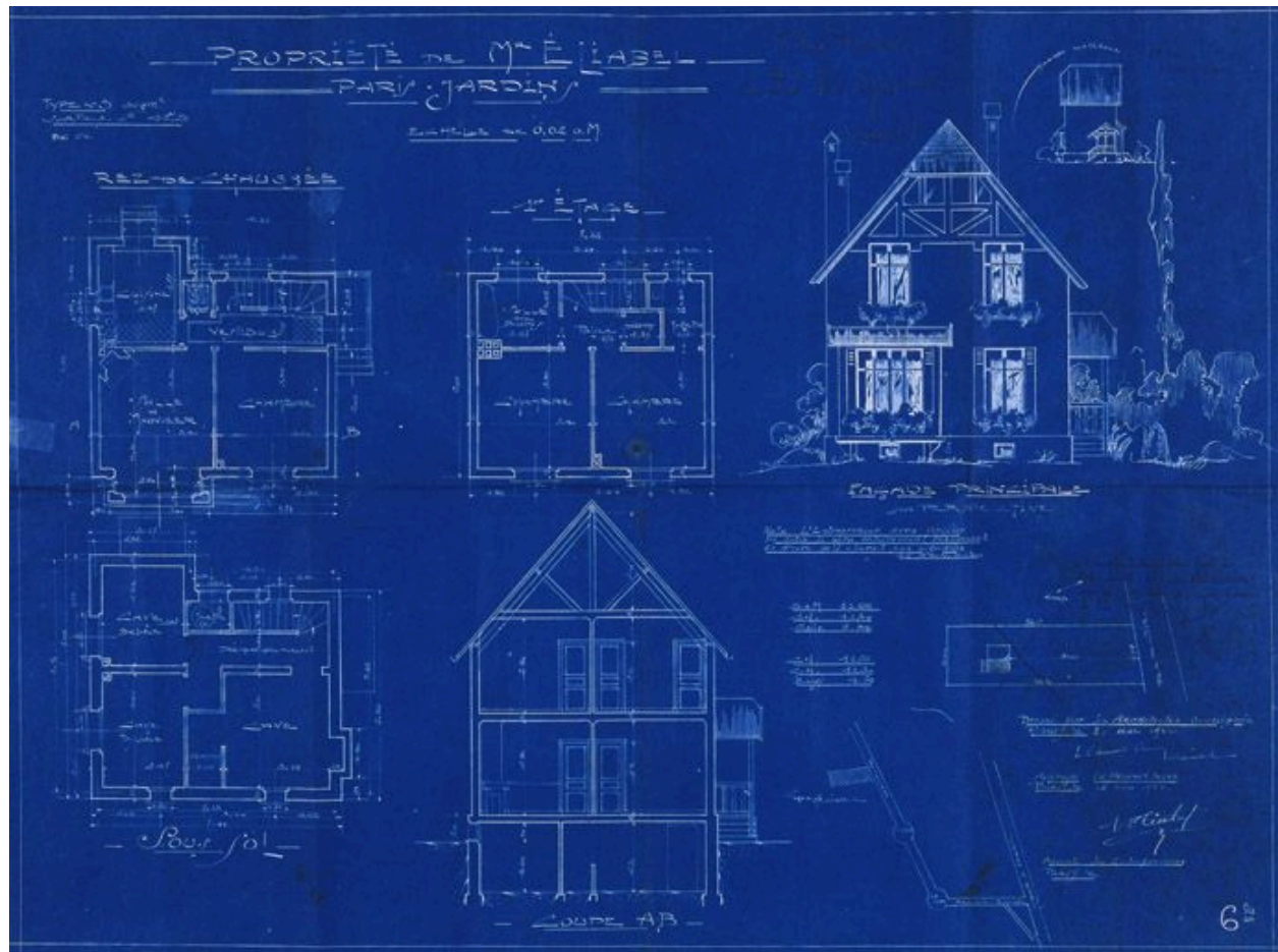
Plans de la maison de M. Eliabel (type n° 3 augmenté) : implantation, élévation principale, coupe et plans par niveaux. (Société coopérative "Paris-Jardins" de Draveil, dossier 172)
