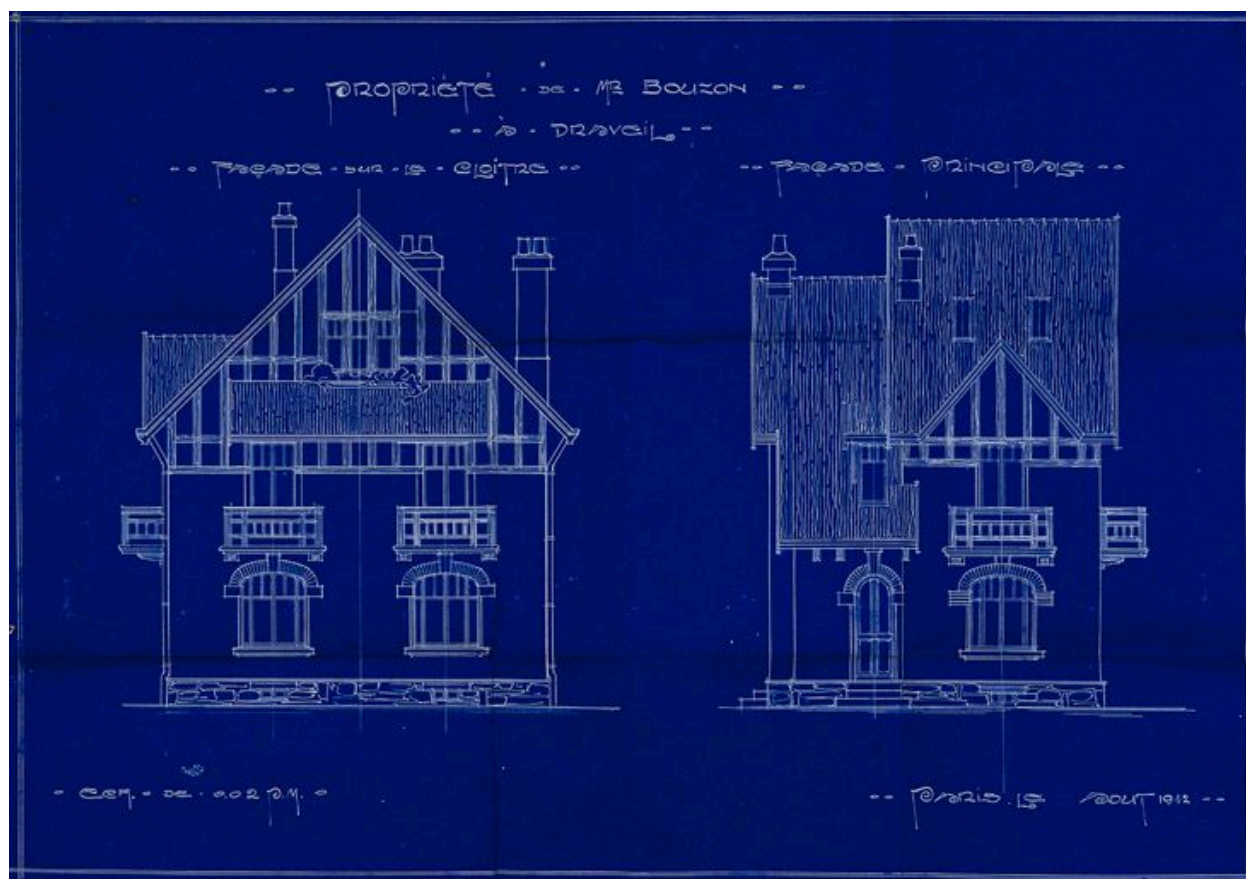
Plan de la maison de M. Bouzon, 1 allée de la Petite-Ferme : façade principale et façade sur le "cloître". (Société coopérative "Paris-Jardins" de Draveil, dossier 92)
