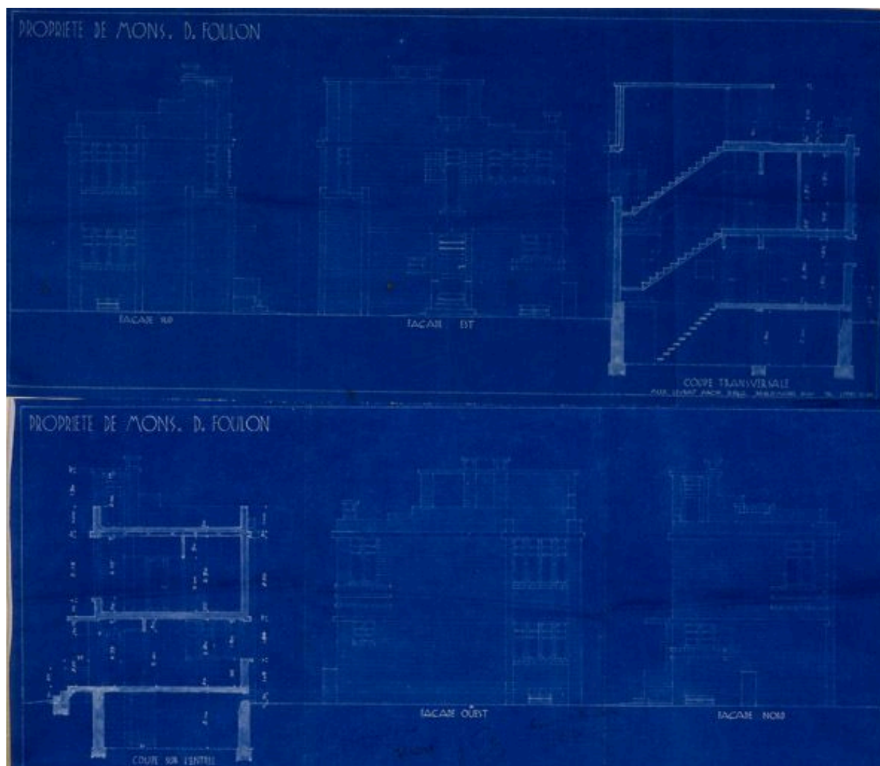
Plan du pavillon construit pour M. Foulon : élévations et coupes. (Société coopérative ""Paris-Jardins"" de Draveil, dossier 921)
