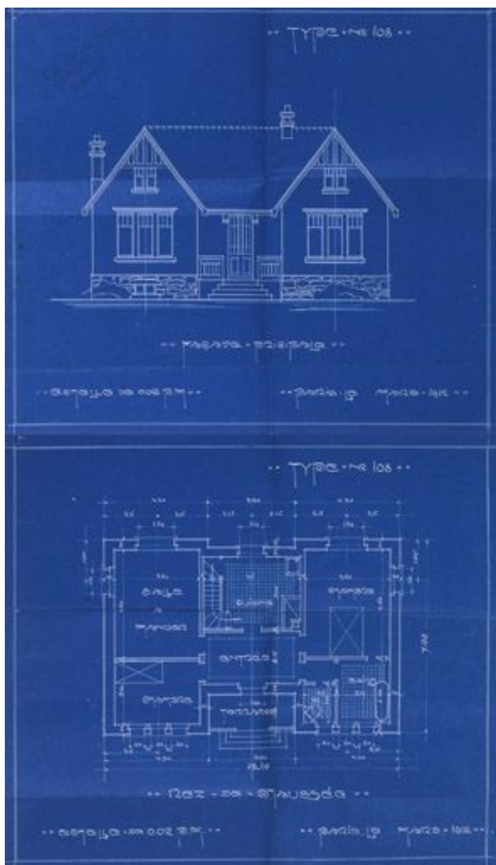
Plan d'une maison du type n° 108 : élévation principale et rez-de-chaussée. (Société coopérative ""Paris-Jardins"" de Draveil, dossier 238)
