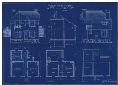
Plan d'un pavillon : élévations, coupe et niveaux. (Société coopérative ""Paris-Jardins"" de Draveil, dossier 101) Phot. Philippe Ayrault, Autr. Pierre (architecte) Prunet, Autr. Roger (architecte) Vasseur IVR11_20069100937XA
